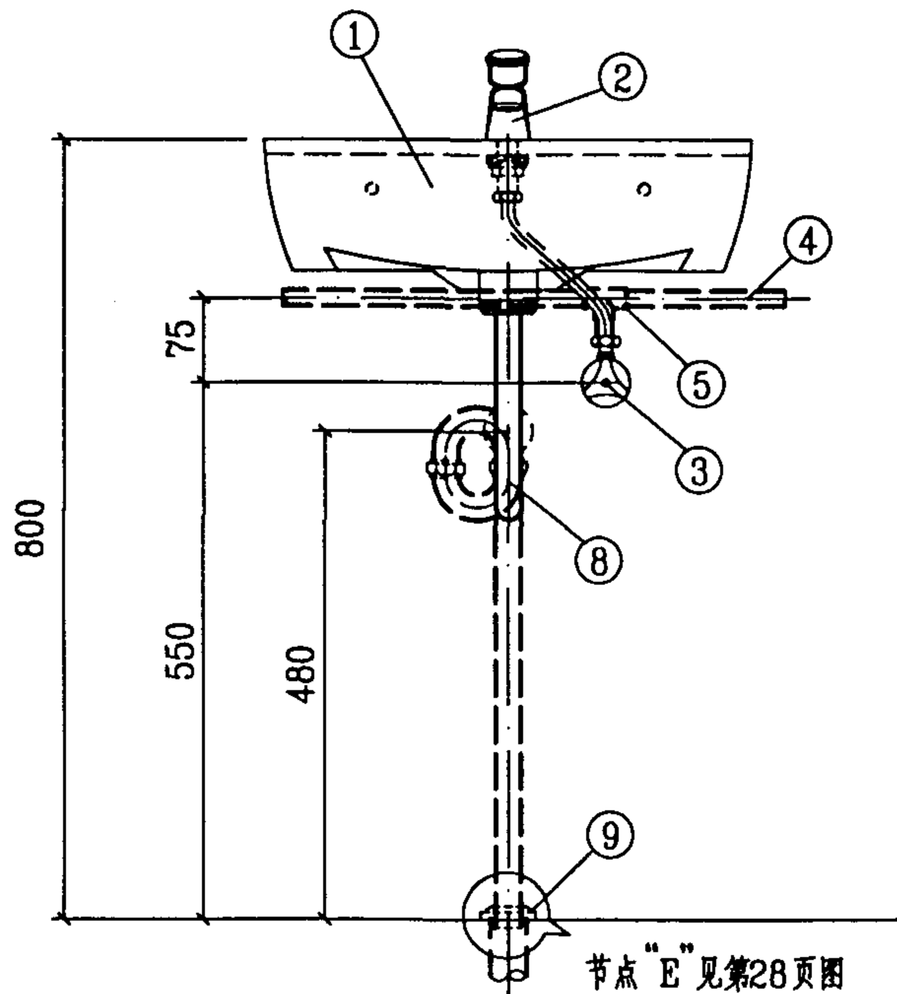
立面图
