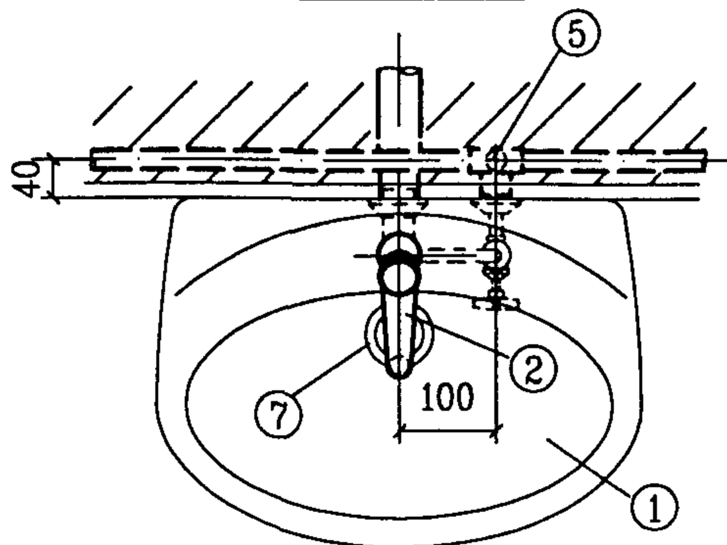
平面图
