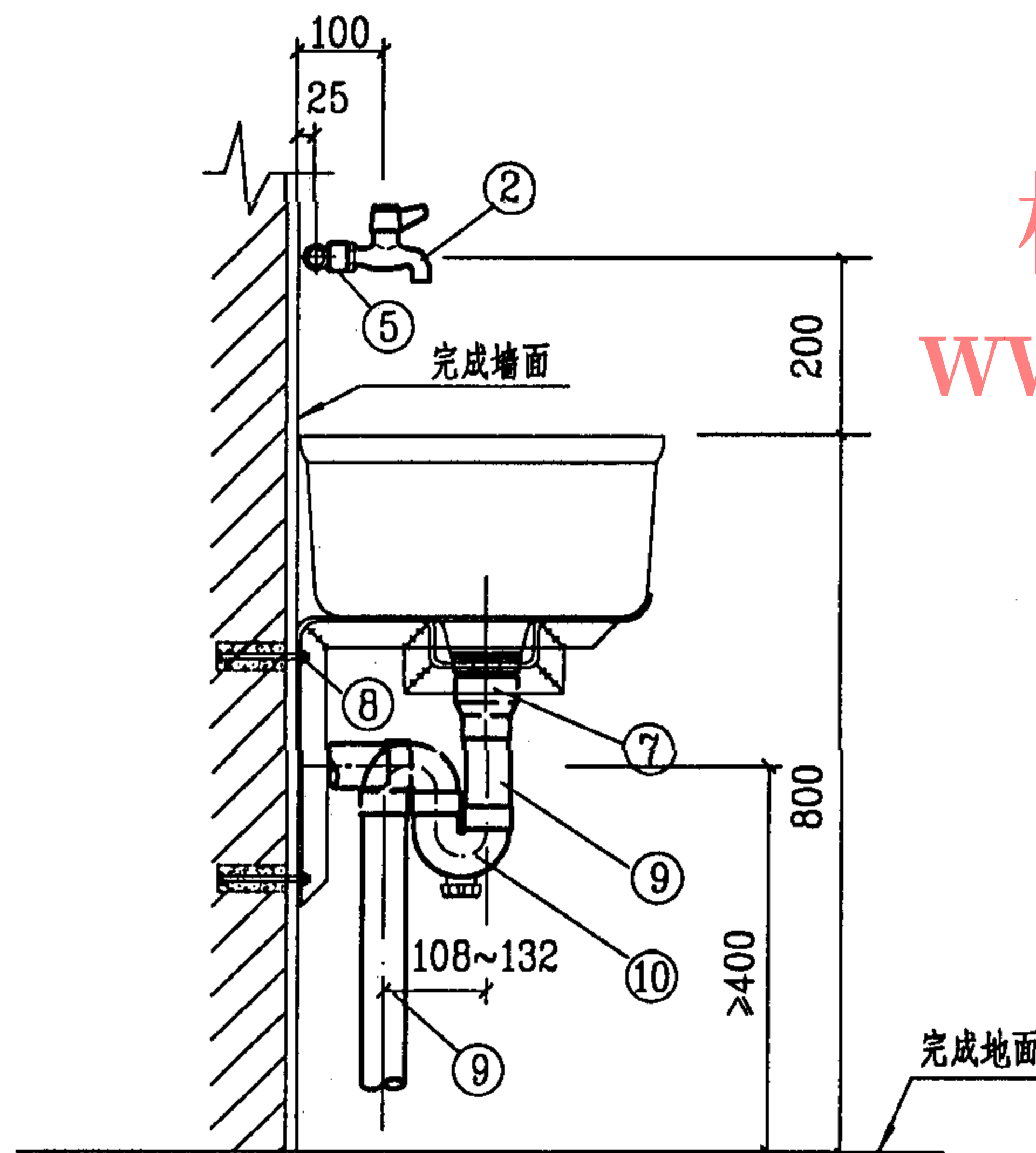
侧面图
