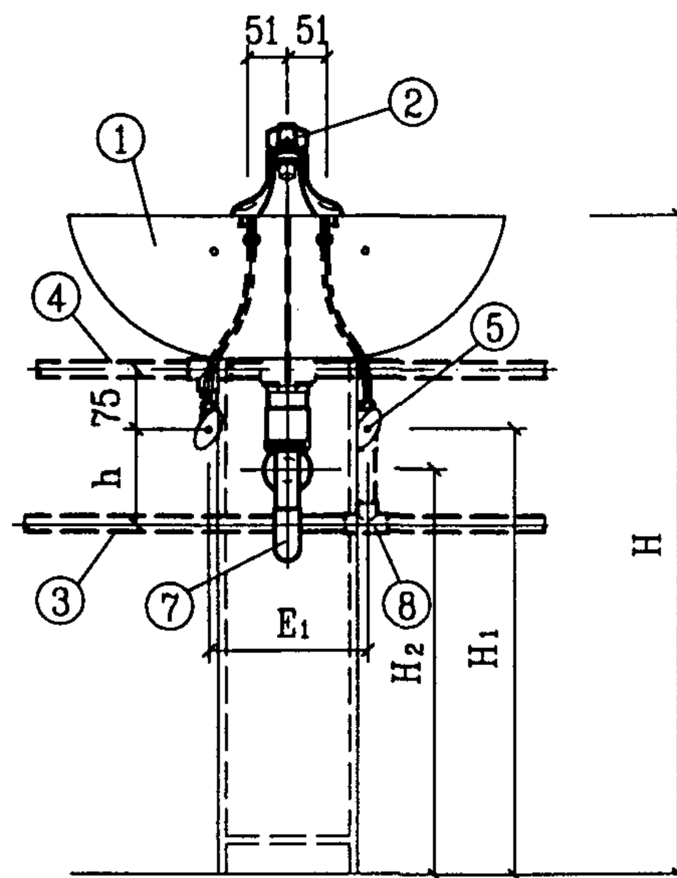
立面图
