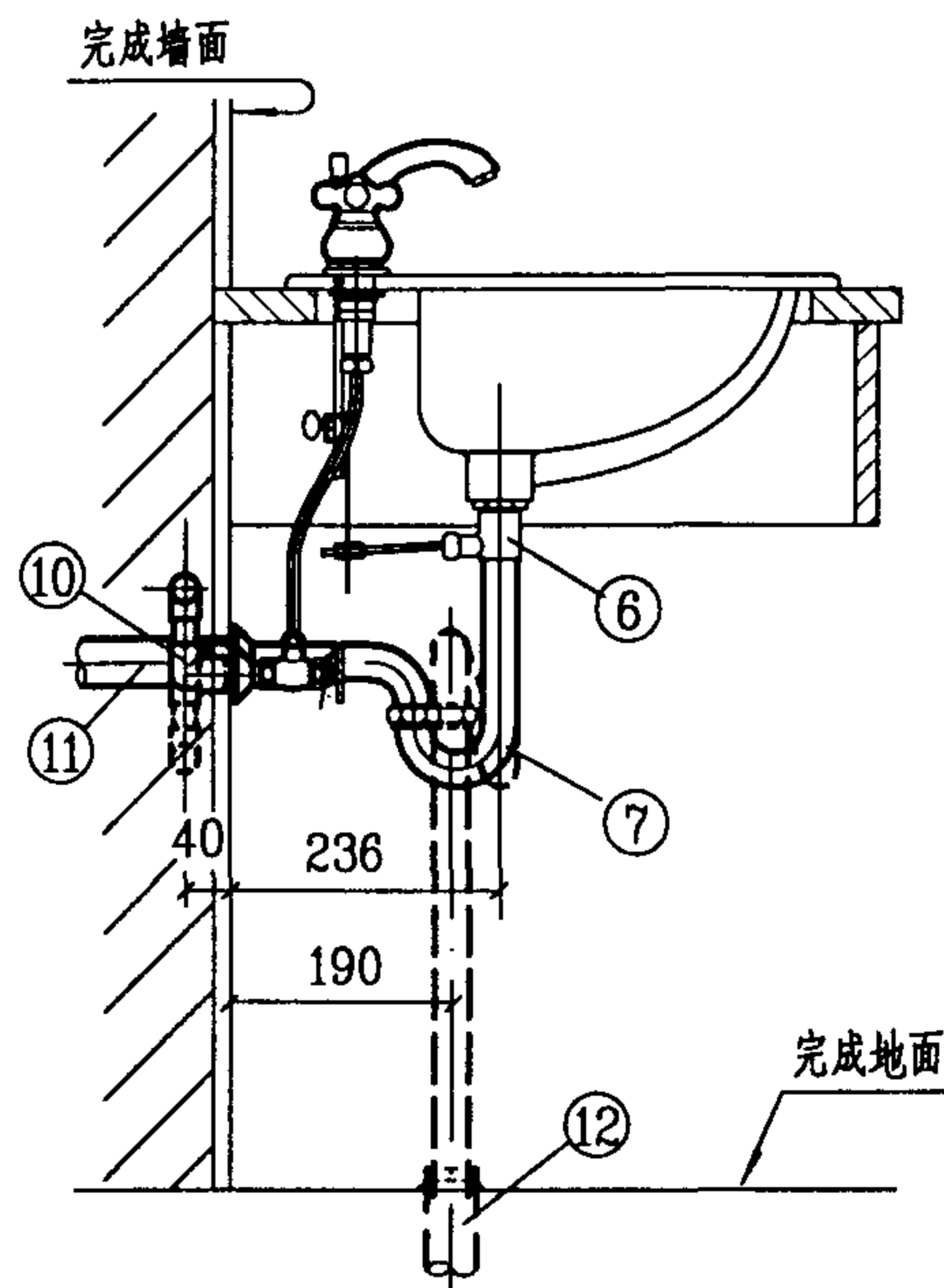
2-2 剖面图
