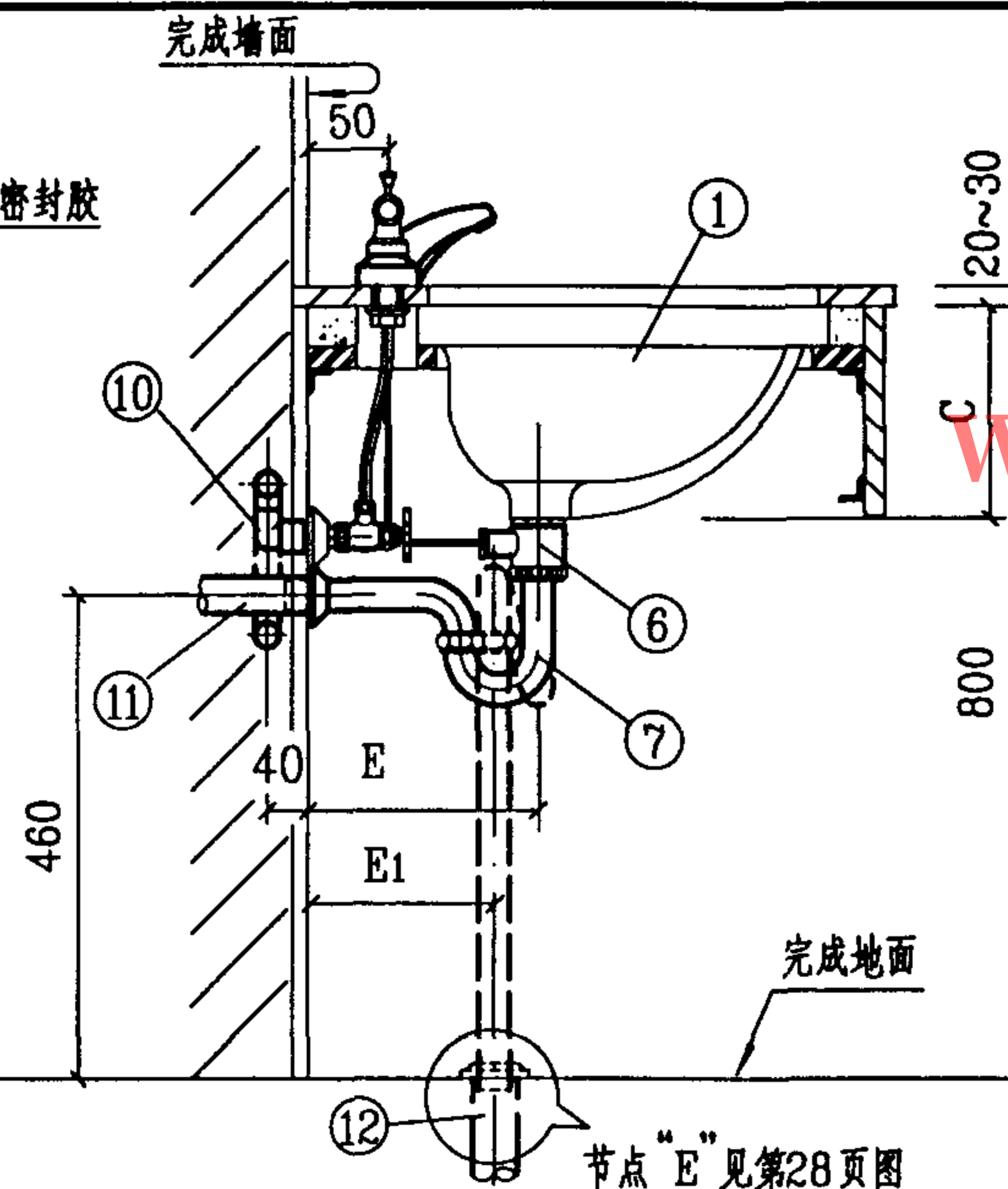
2-2 剖面图
