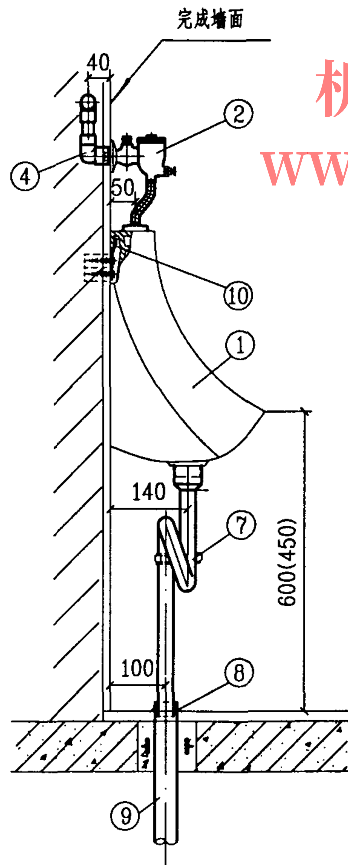
侧面图
