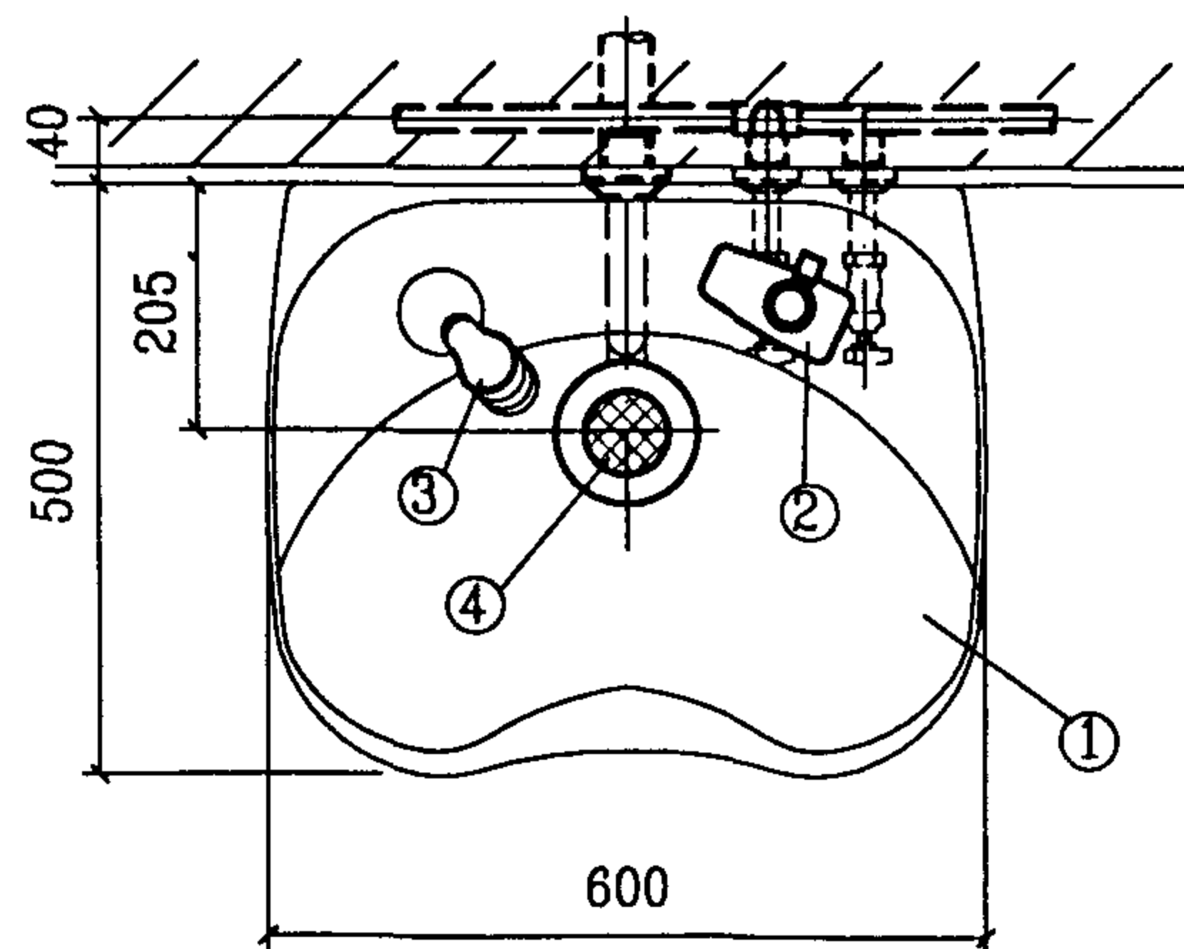
平面图
