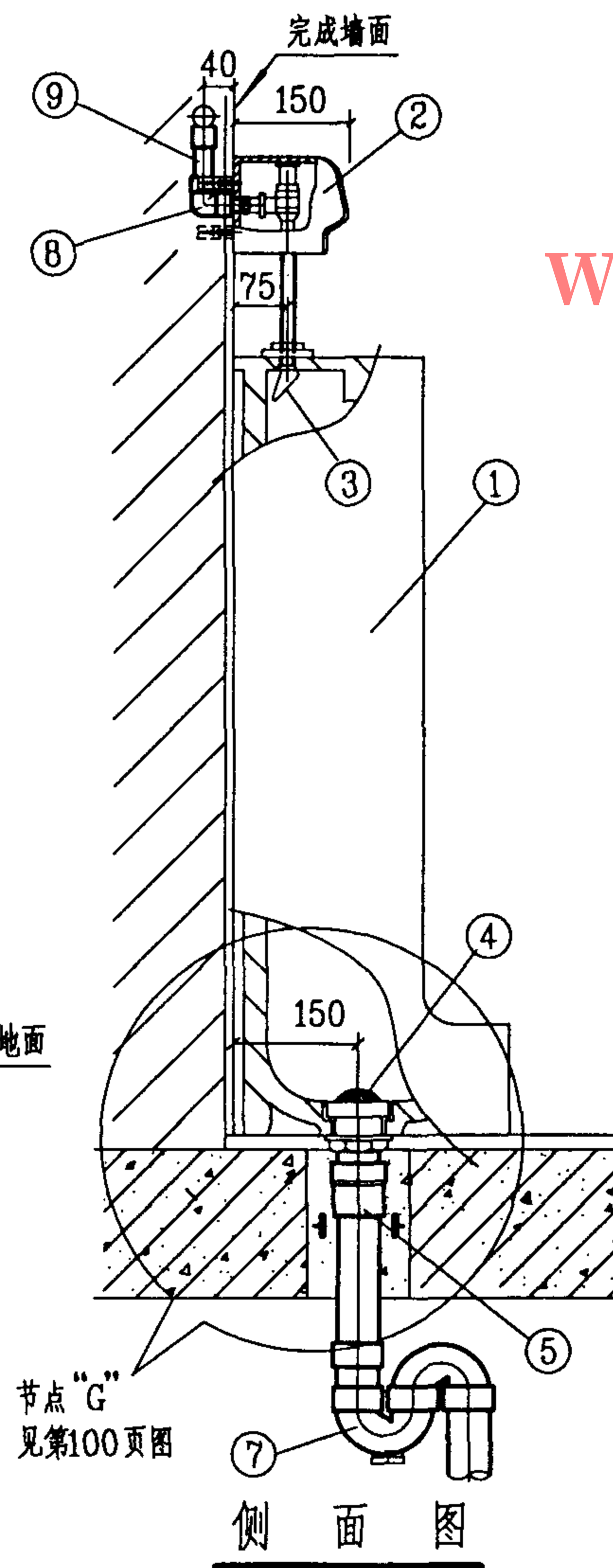
感应式冲洗阀落地式小便器安装图
