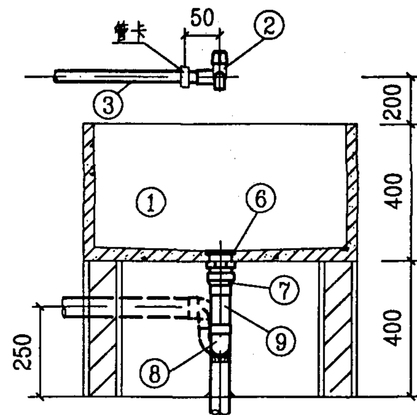
4-4剖面图
