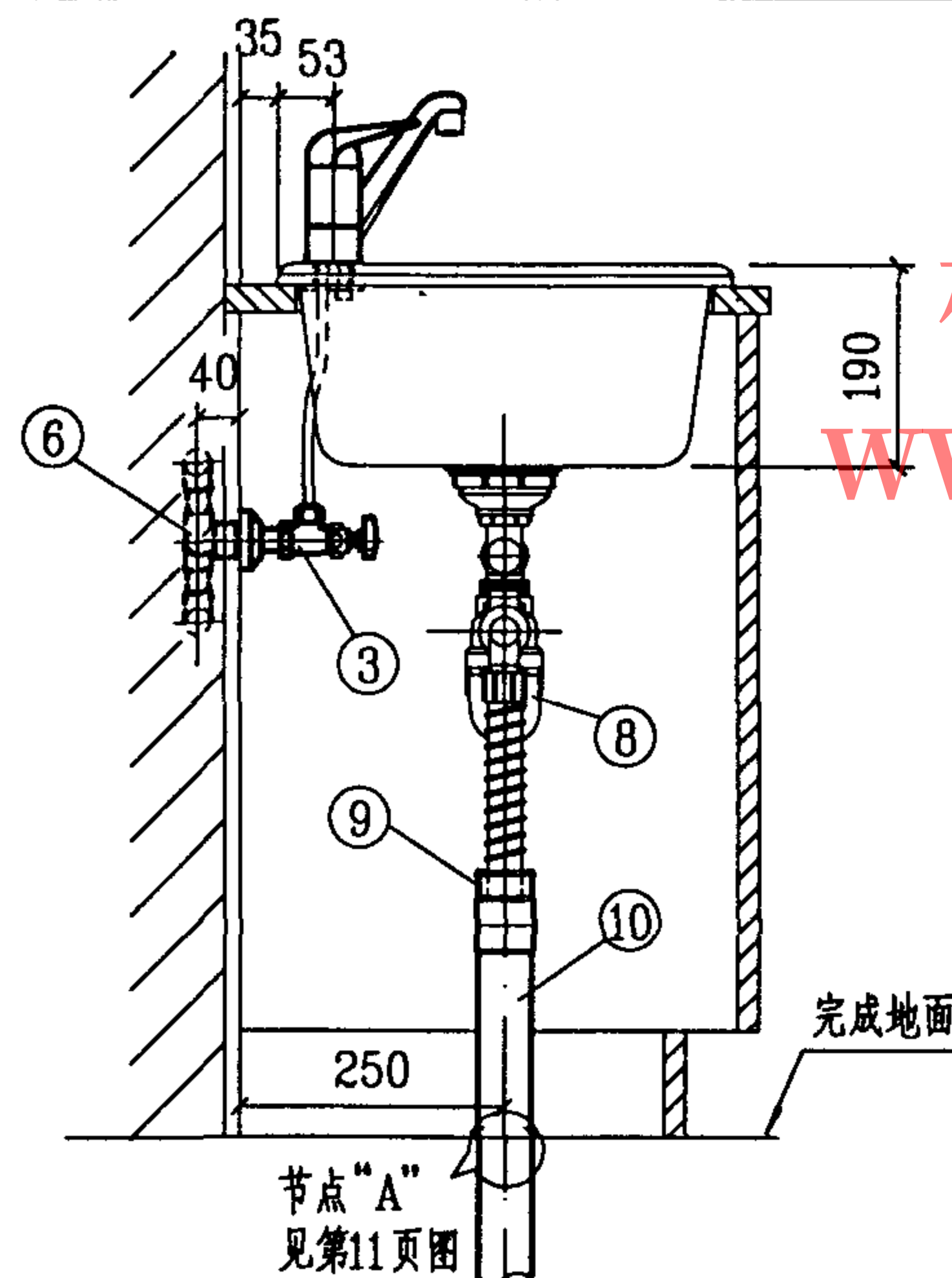
2-2 剖面图
