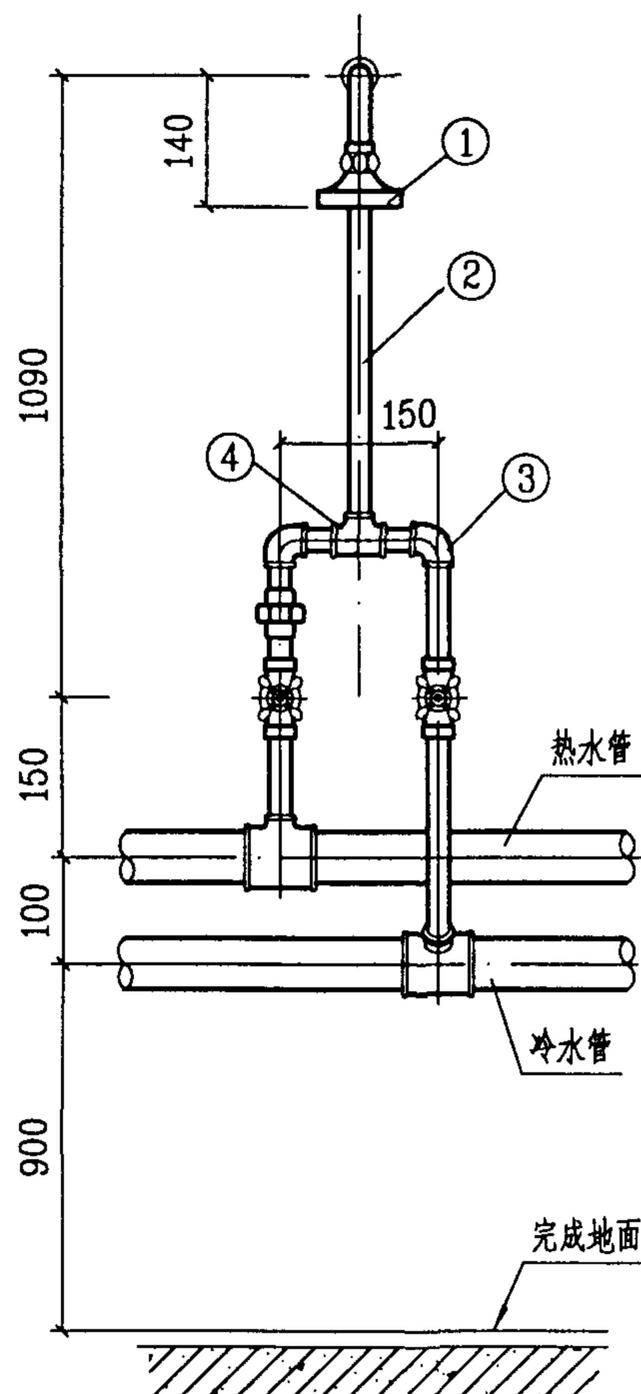
立面图
