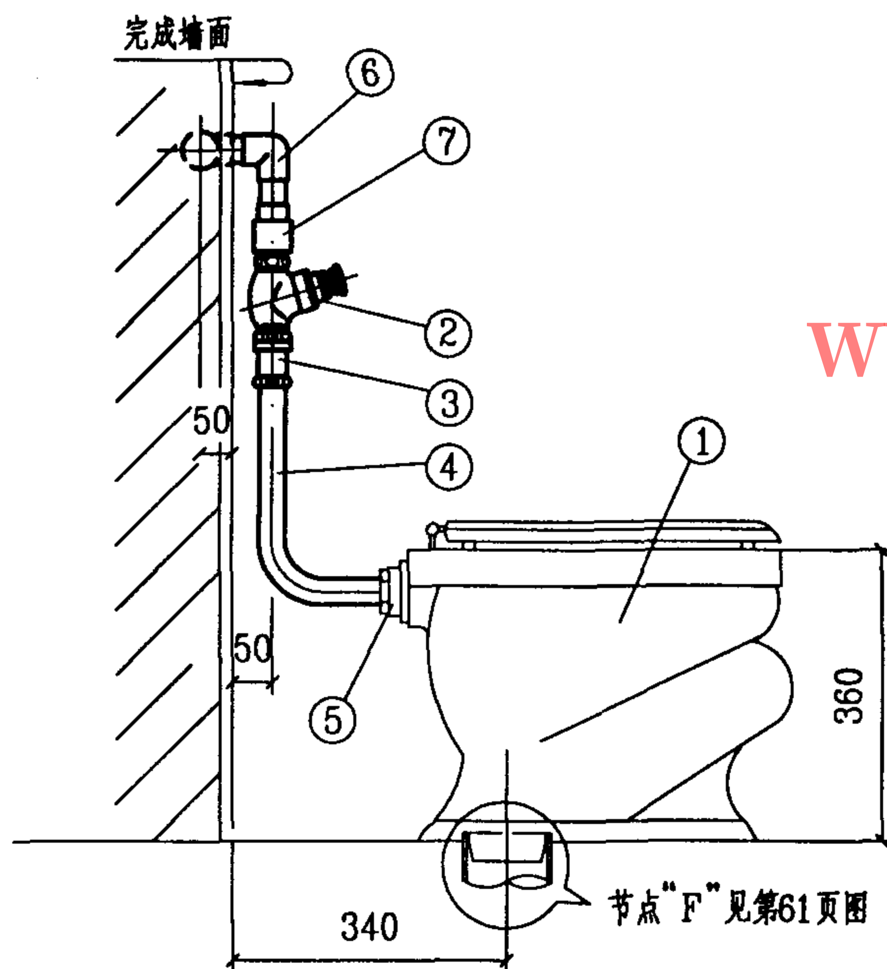
侧面图
