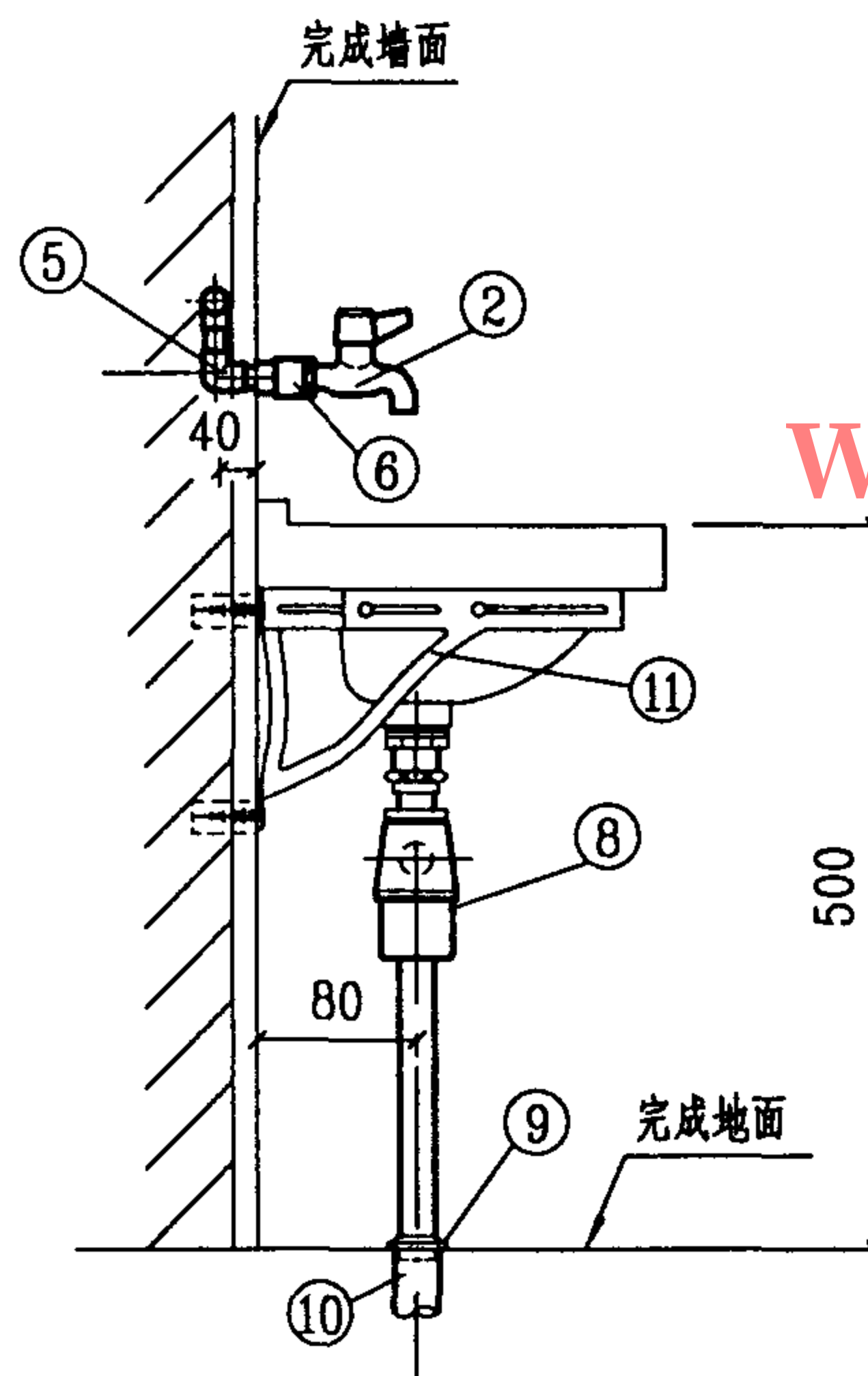
侧面图
