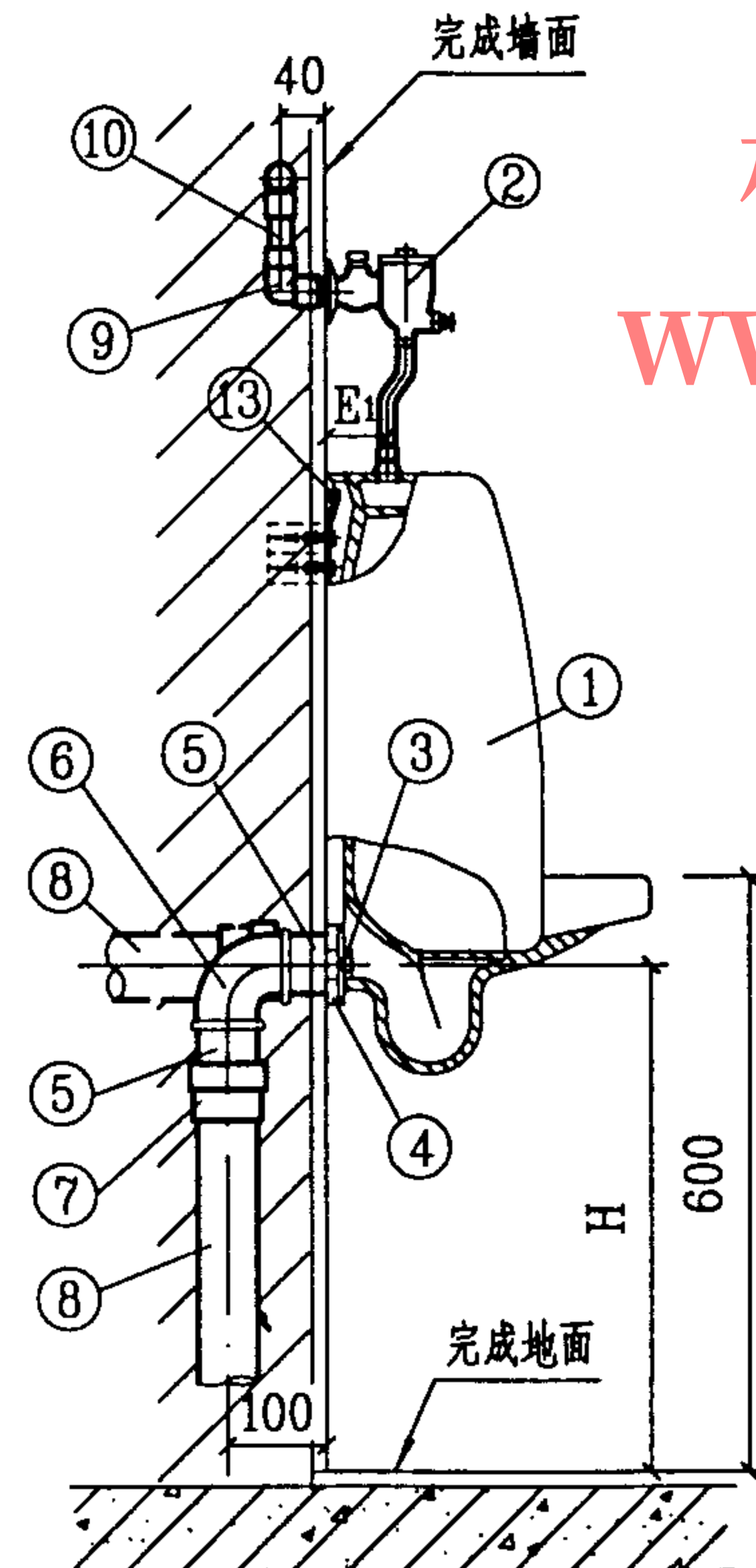
侧面图
