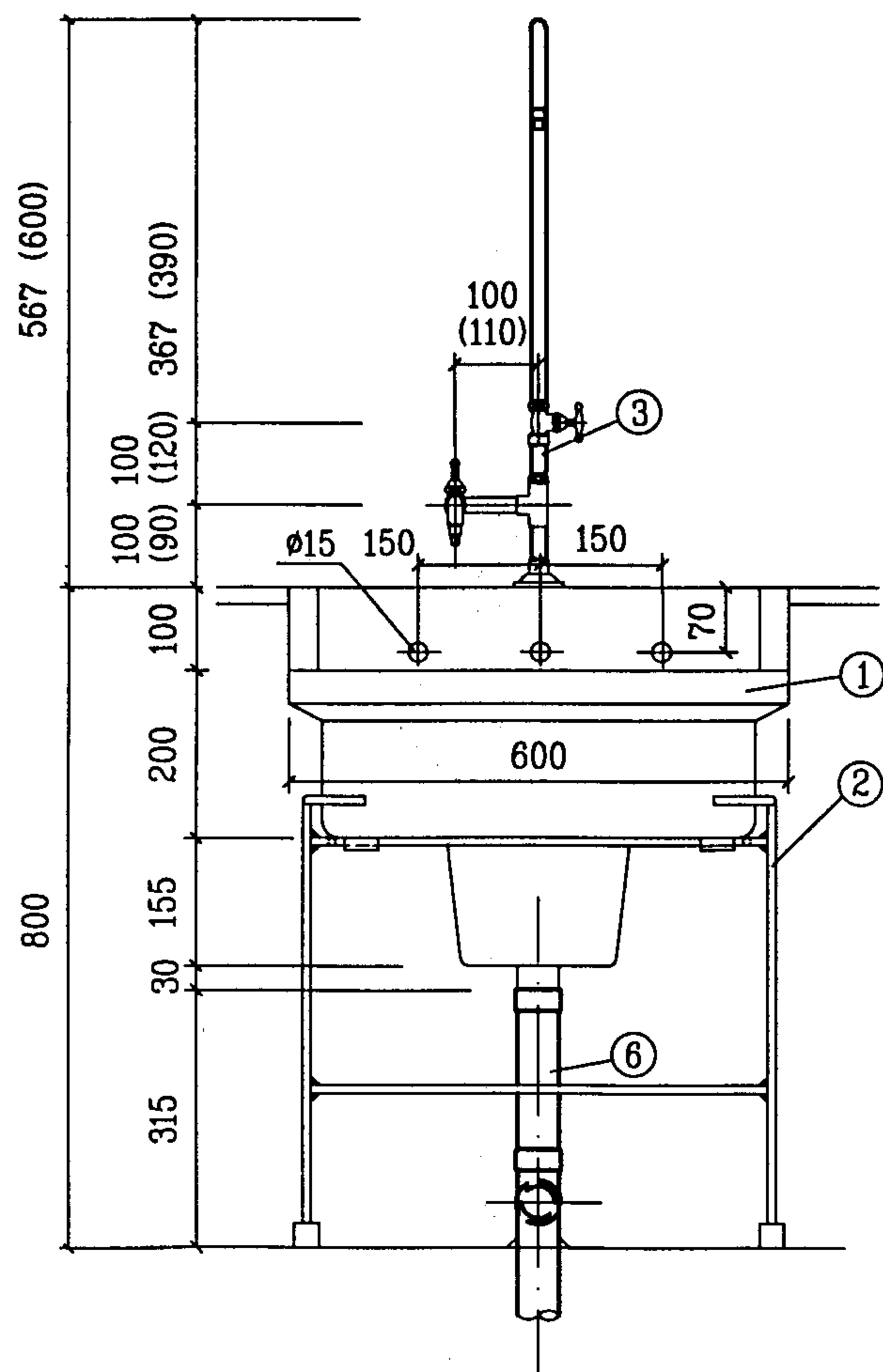
立 面 图
