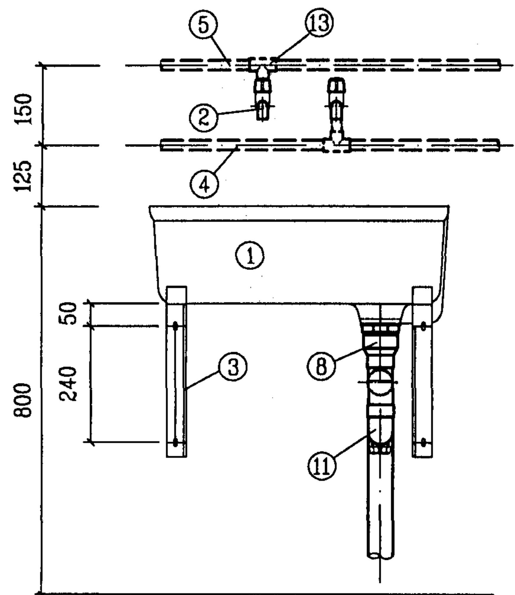
立面图
