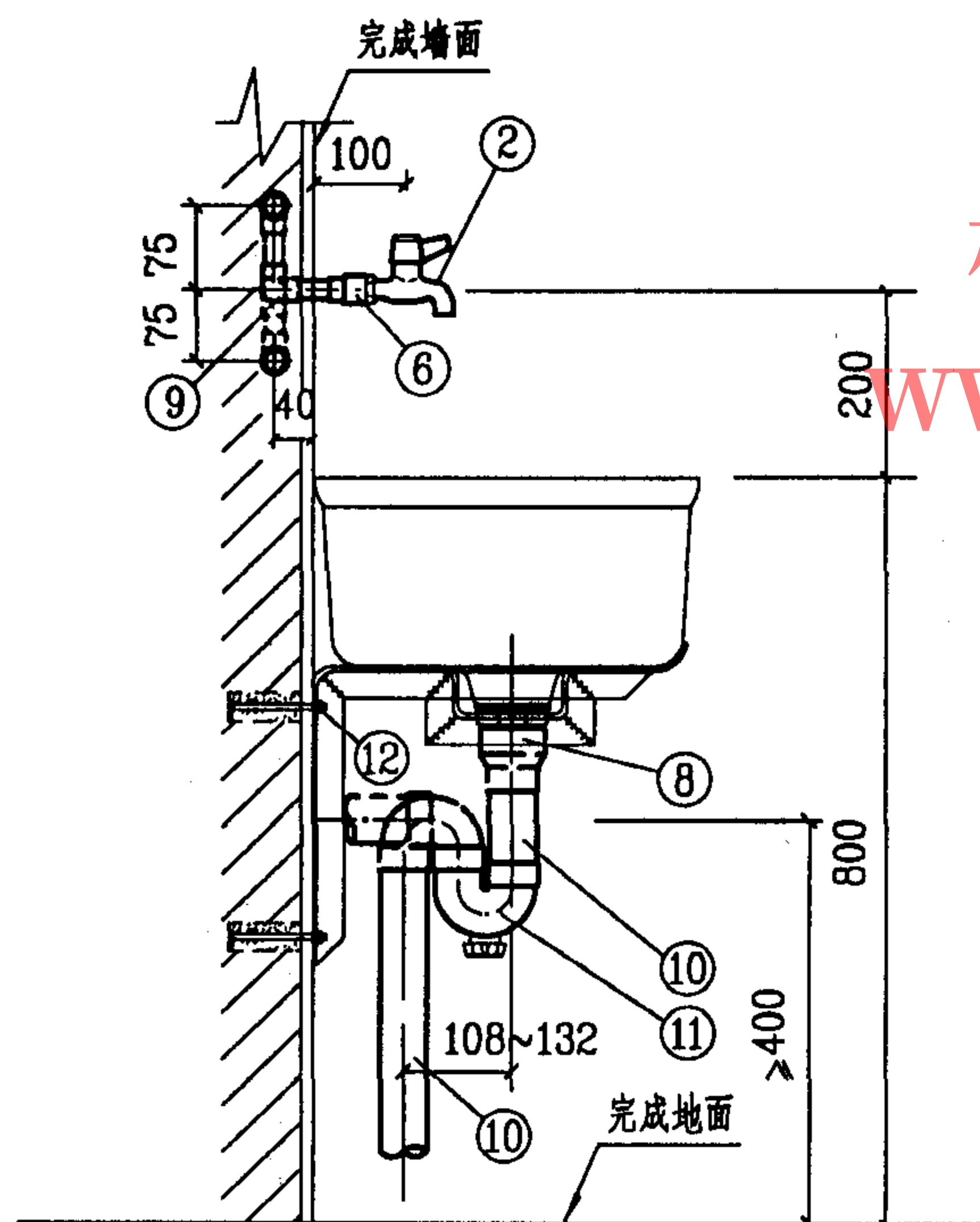
侧面图
