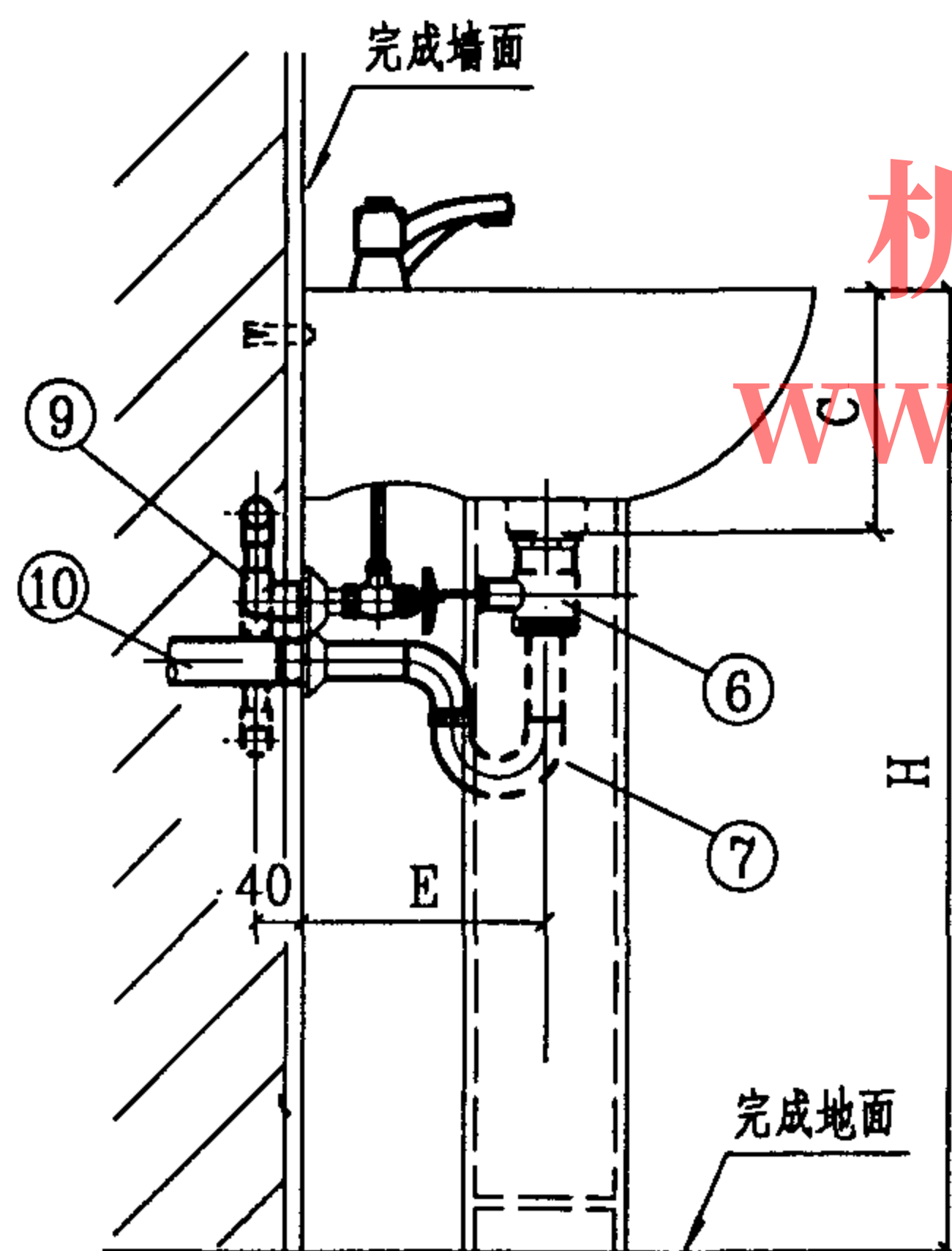
侧面图
