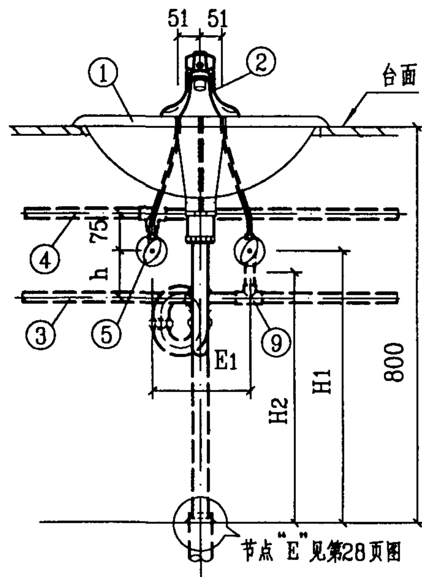
1-1 剖面图
