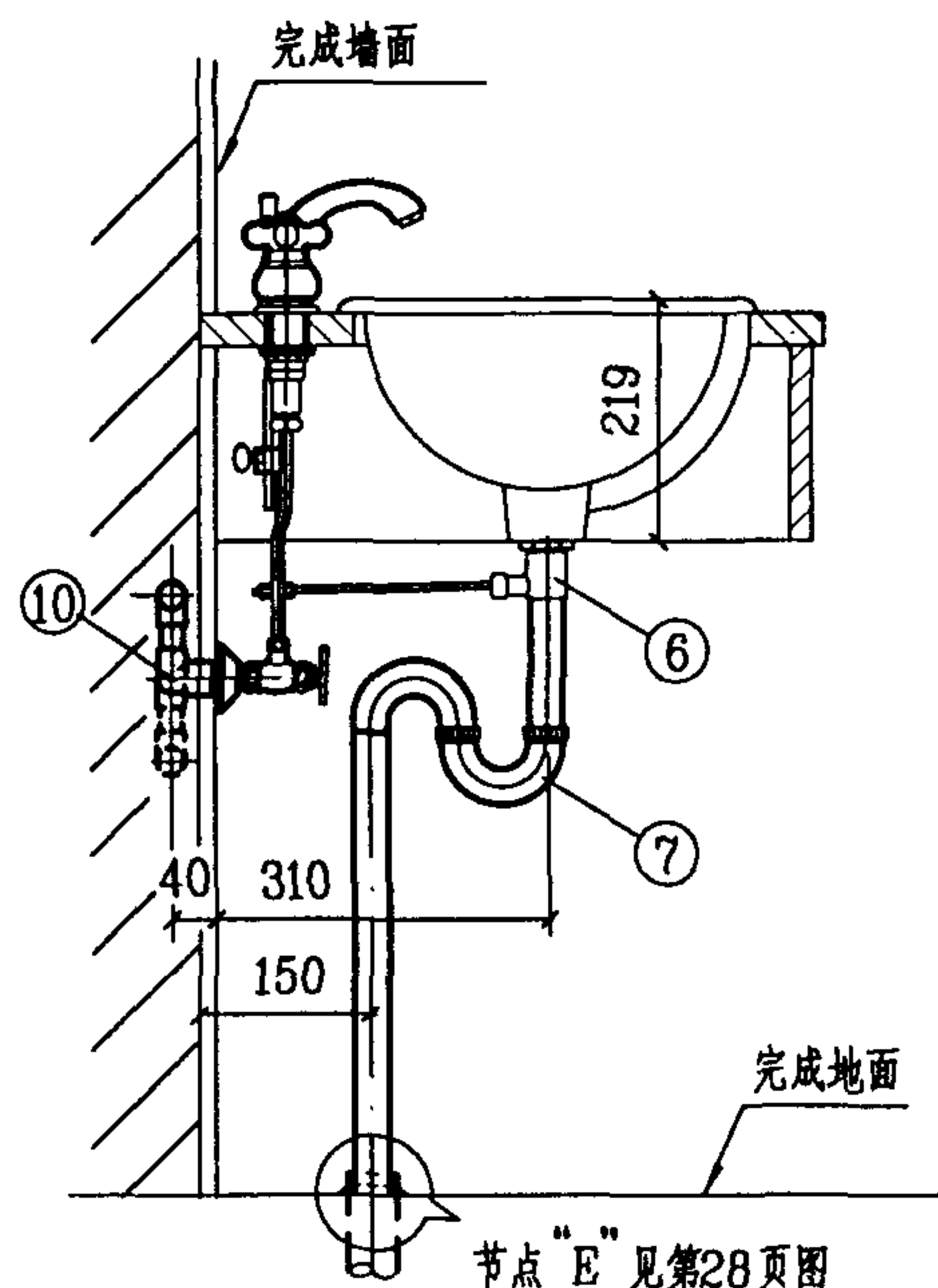
2-2 剖面图
