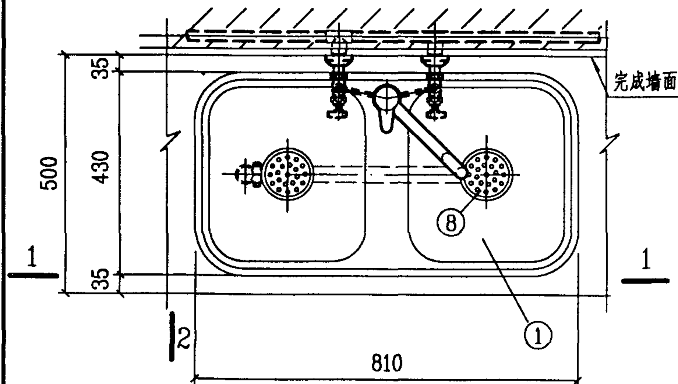
平面图
