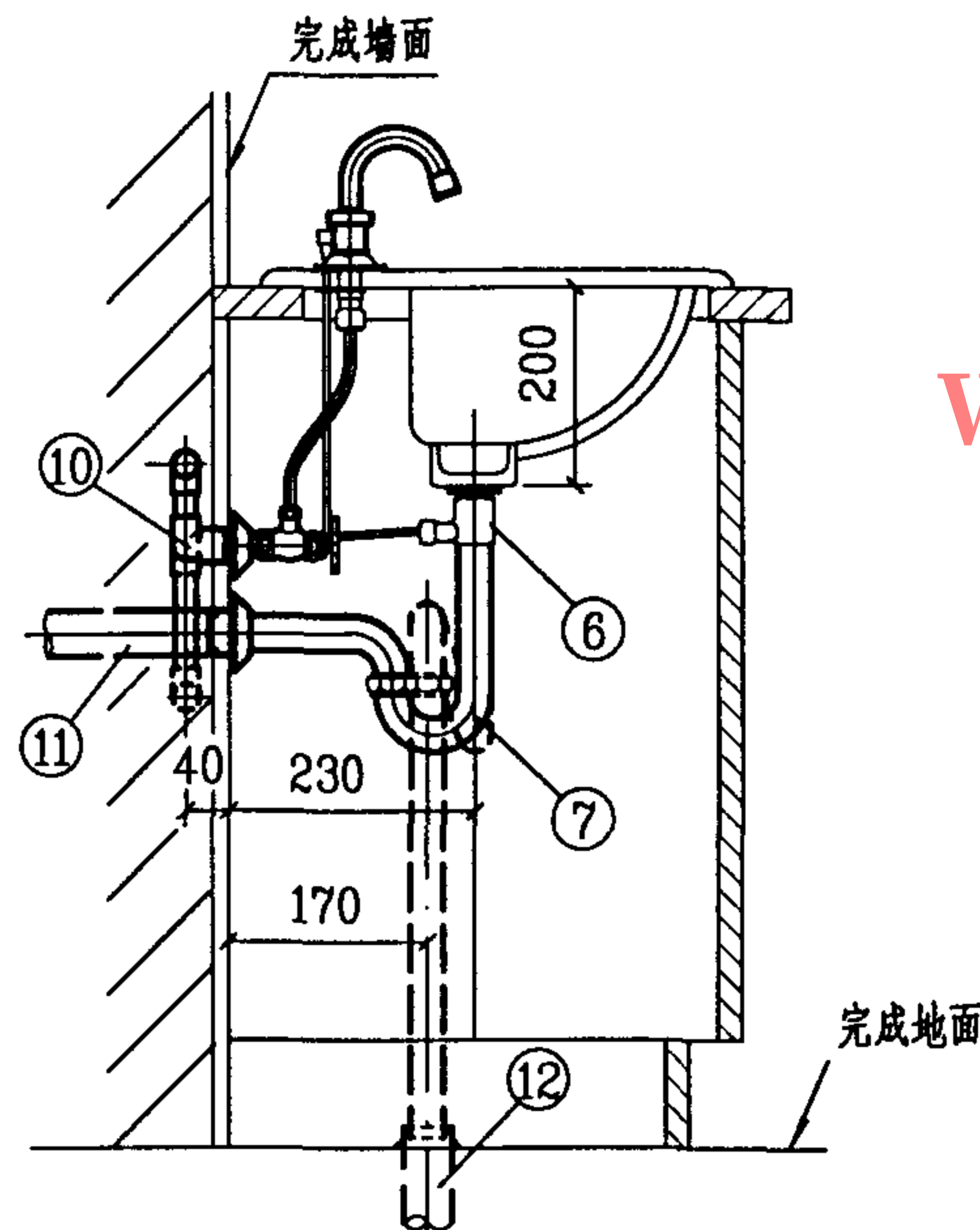
2-2 剖面图
