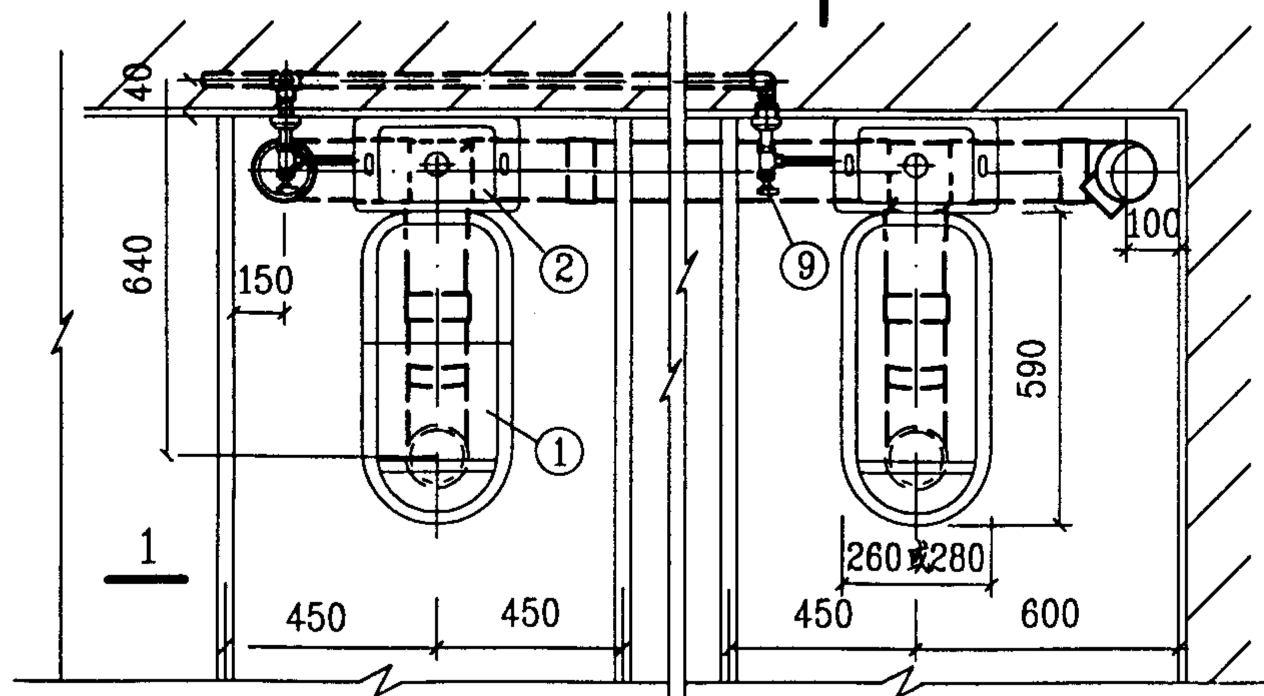
平面图
