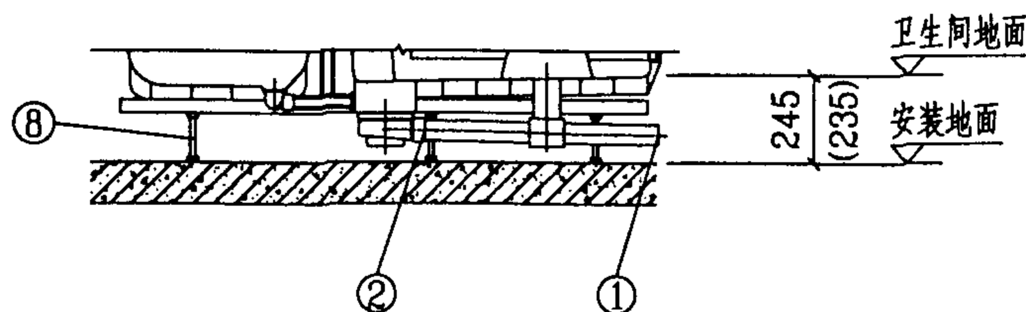
地漏横排同层排水
