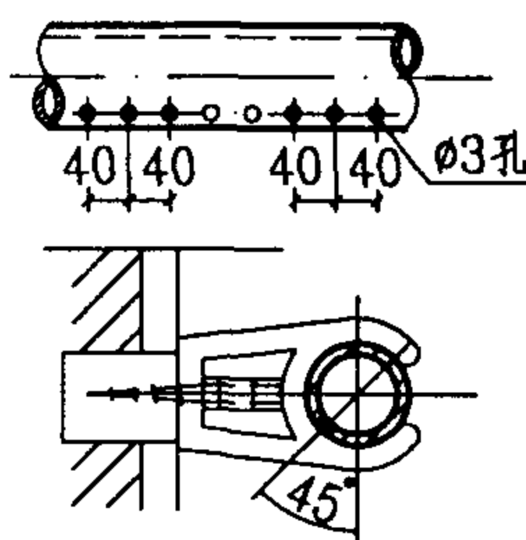
多孔管详图
