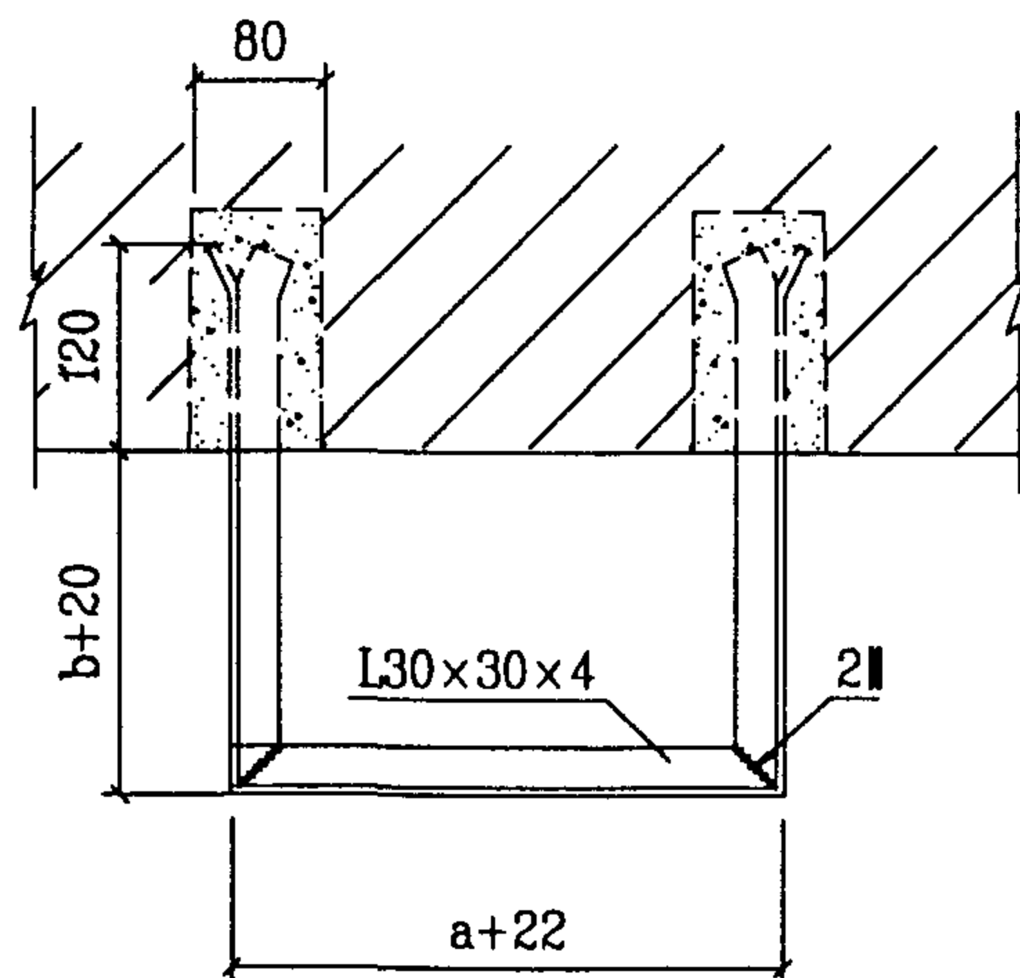
水箱支架图
