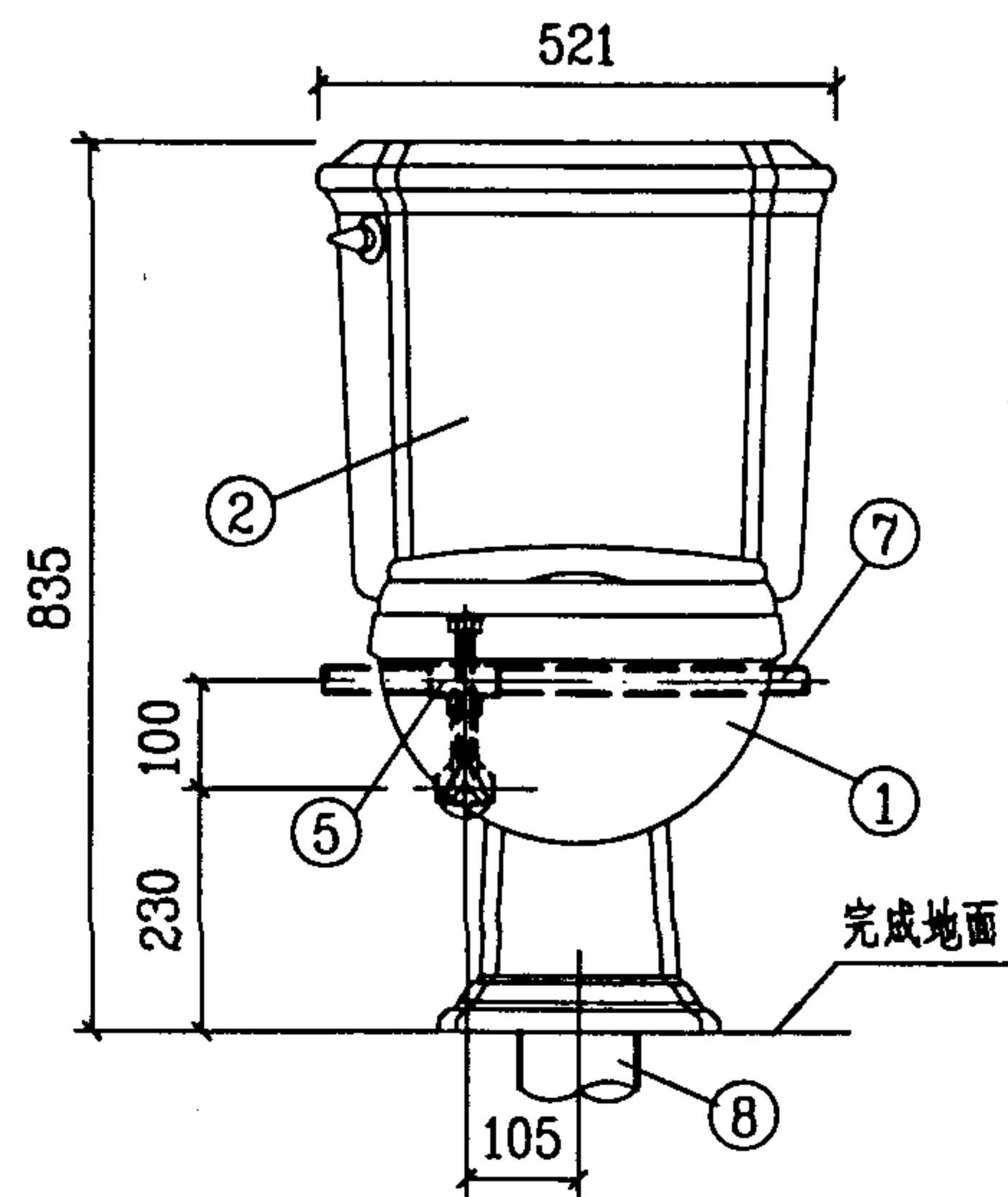
立面图
