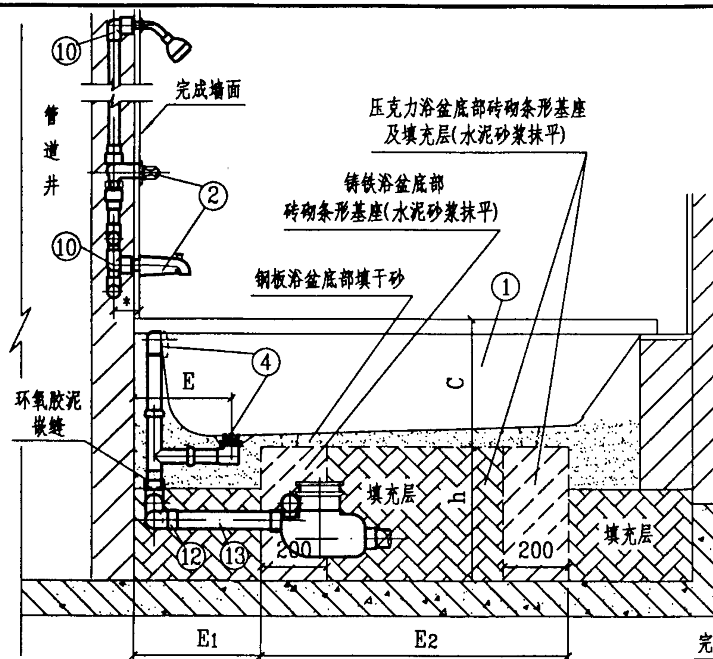
1-1 剖面图
