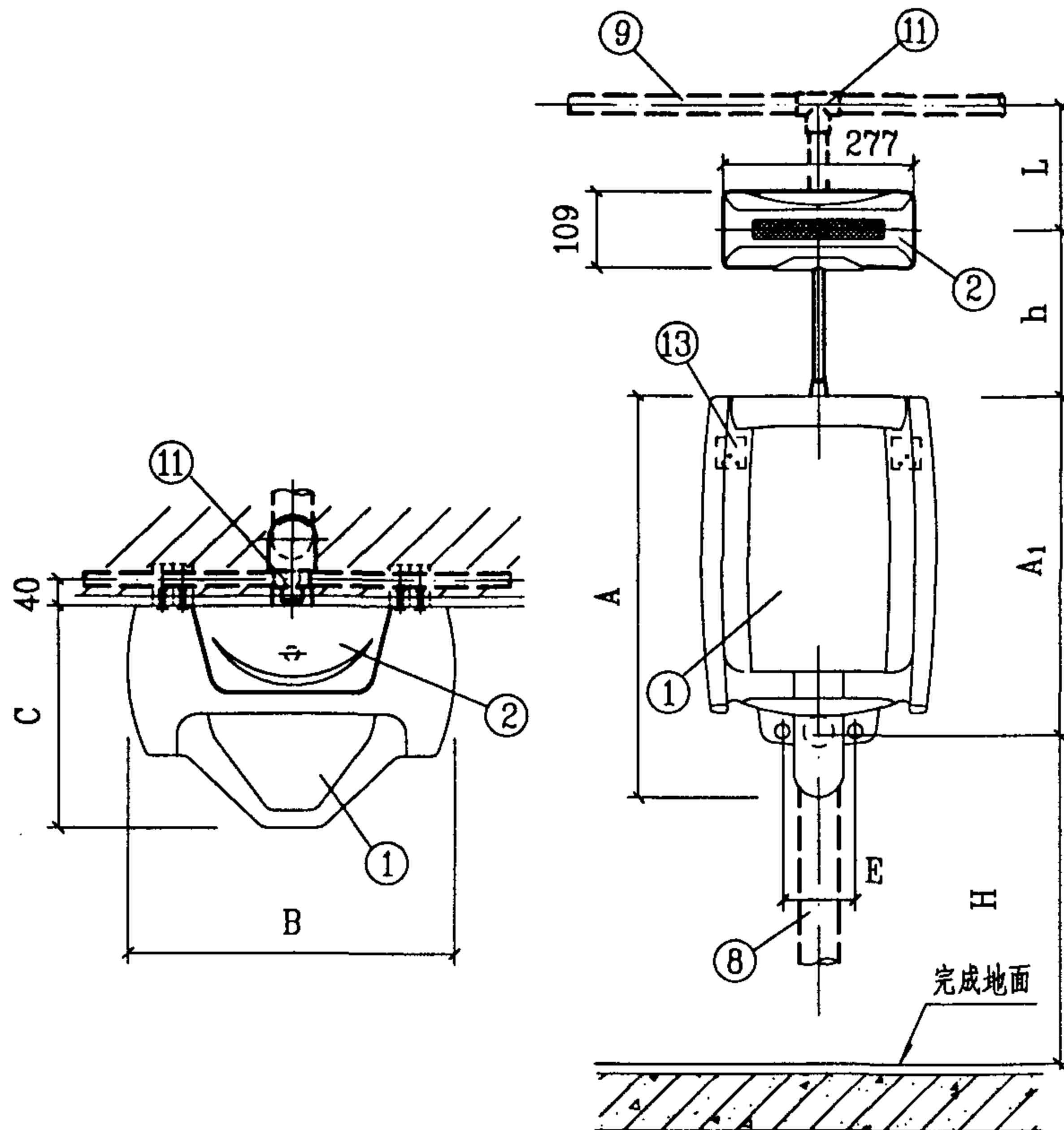
平面图
