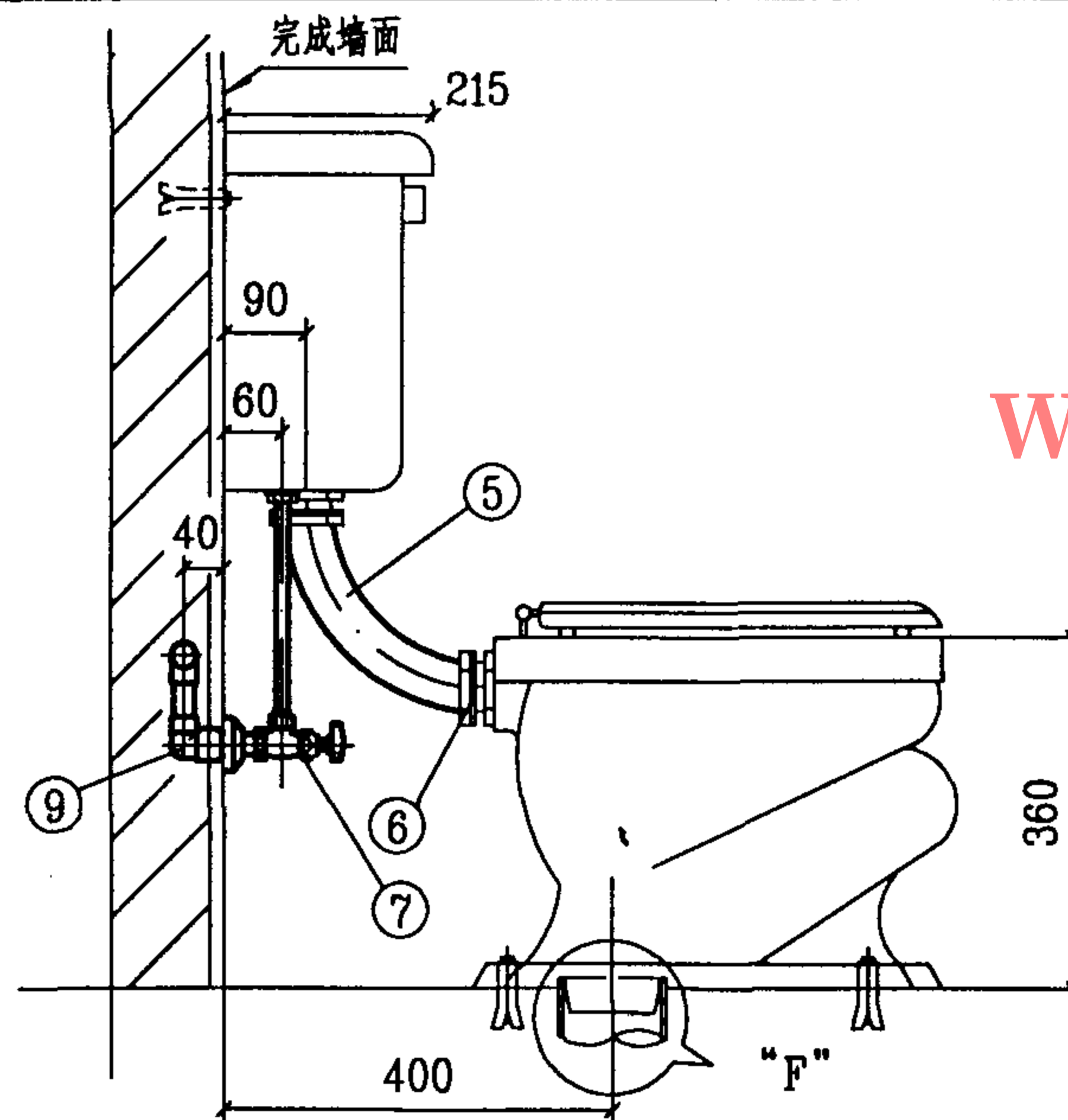
侧面图
