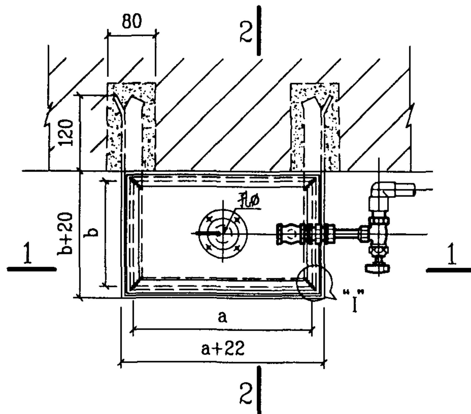
平面图
