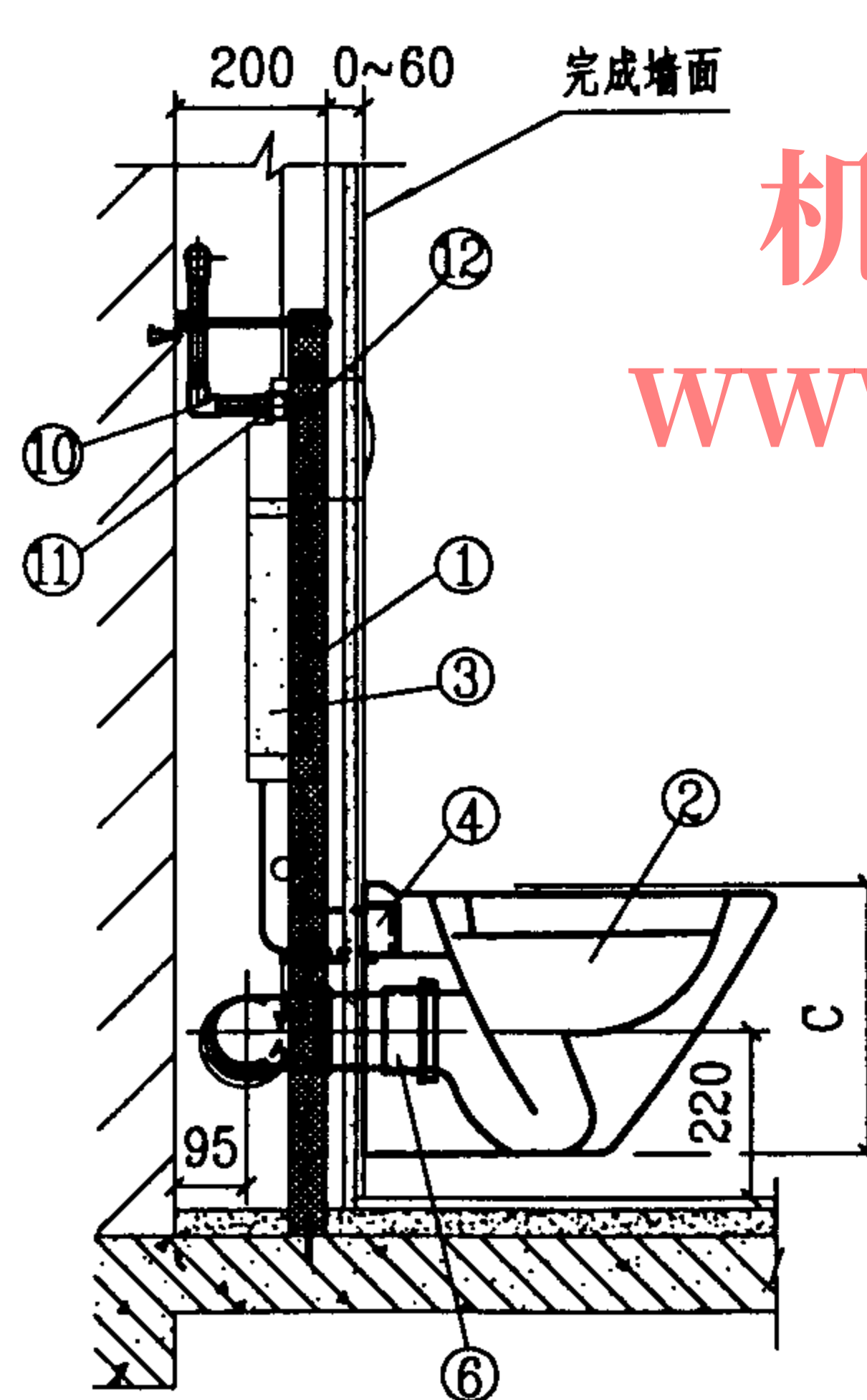
侧面图
