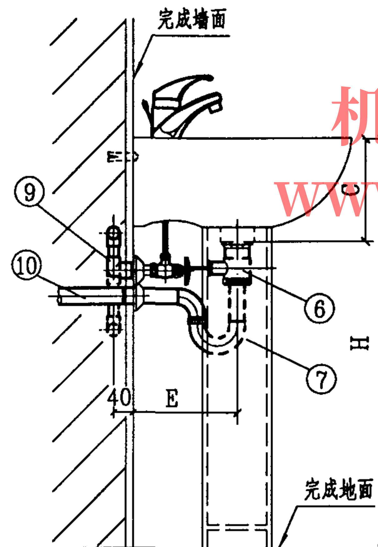
侧面图
