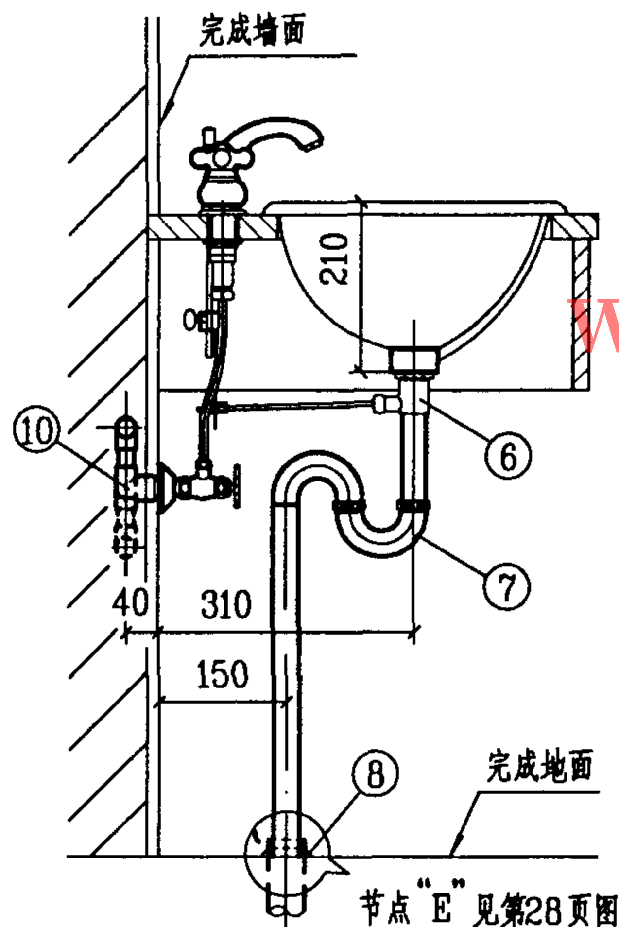
2-2 剖面图
