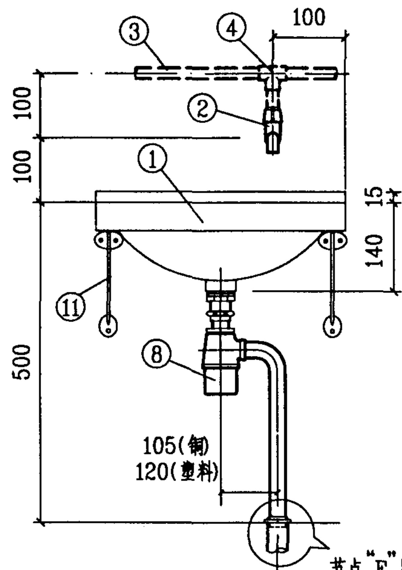
立面图
