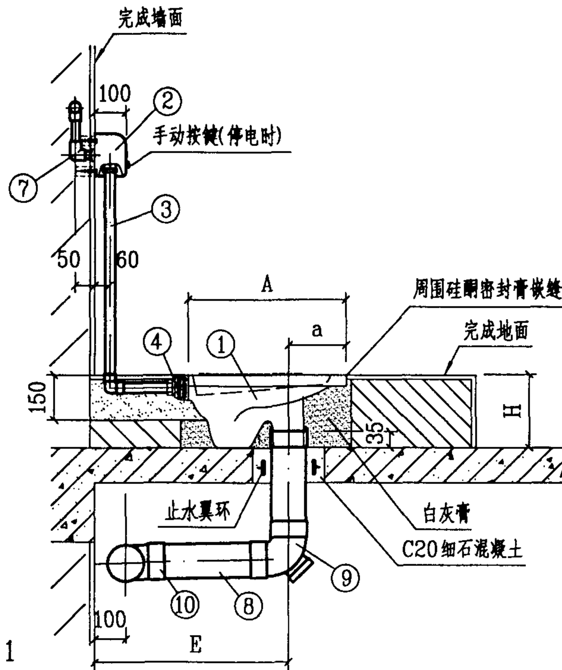
2-2 剖面图
