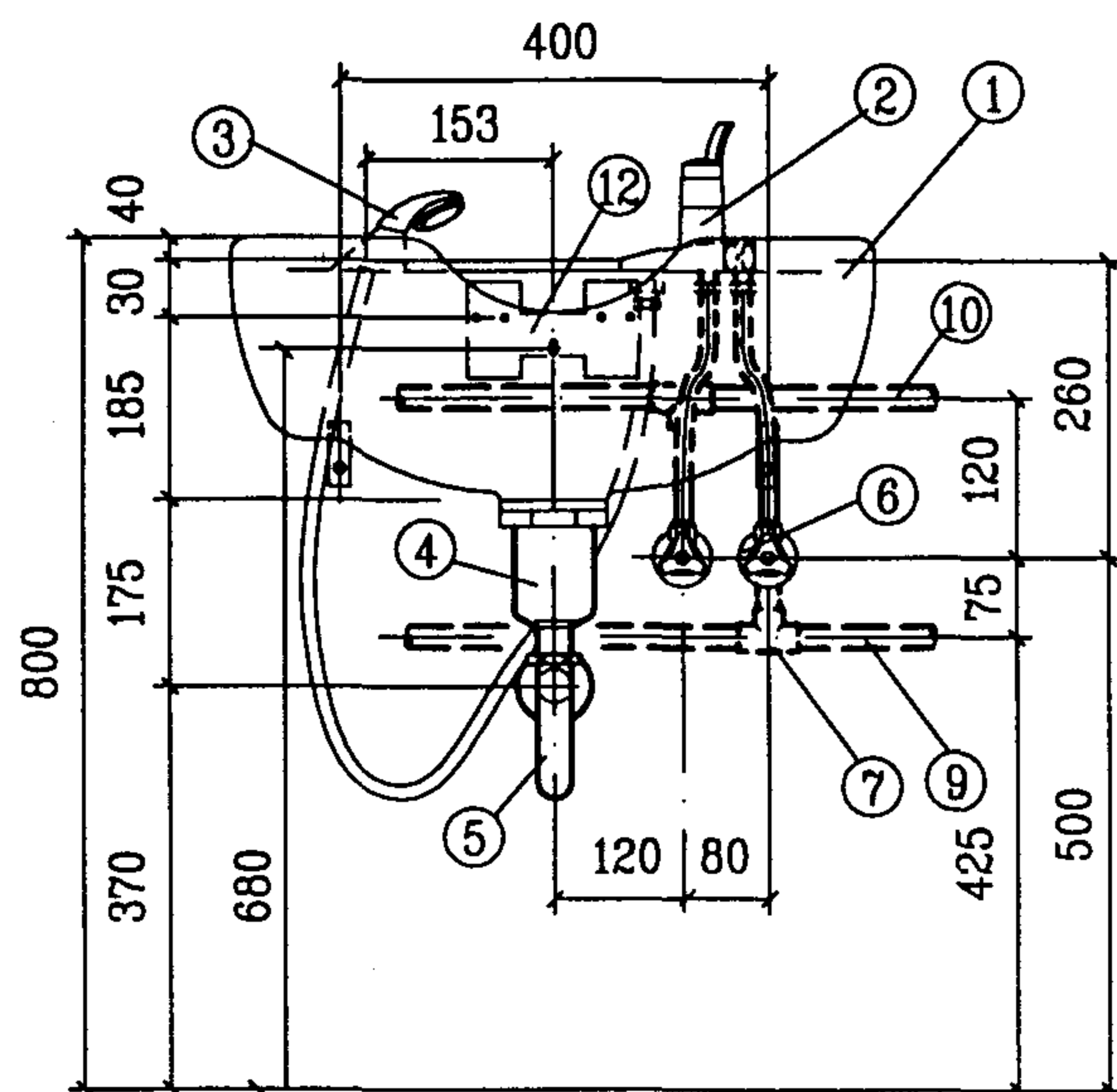
立面图
