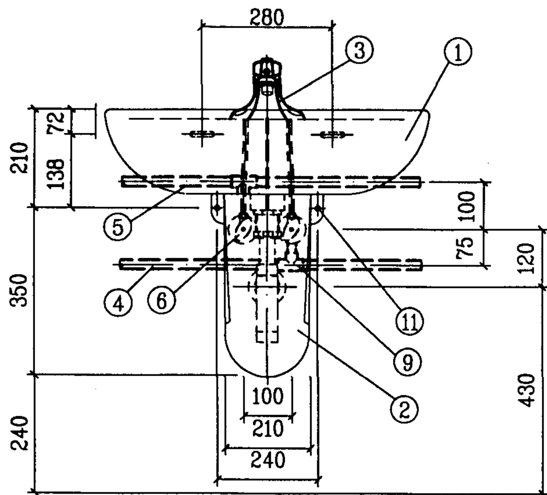
立面图
