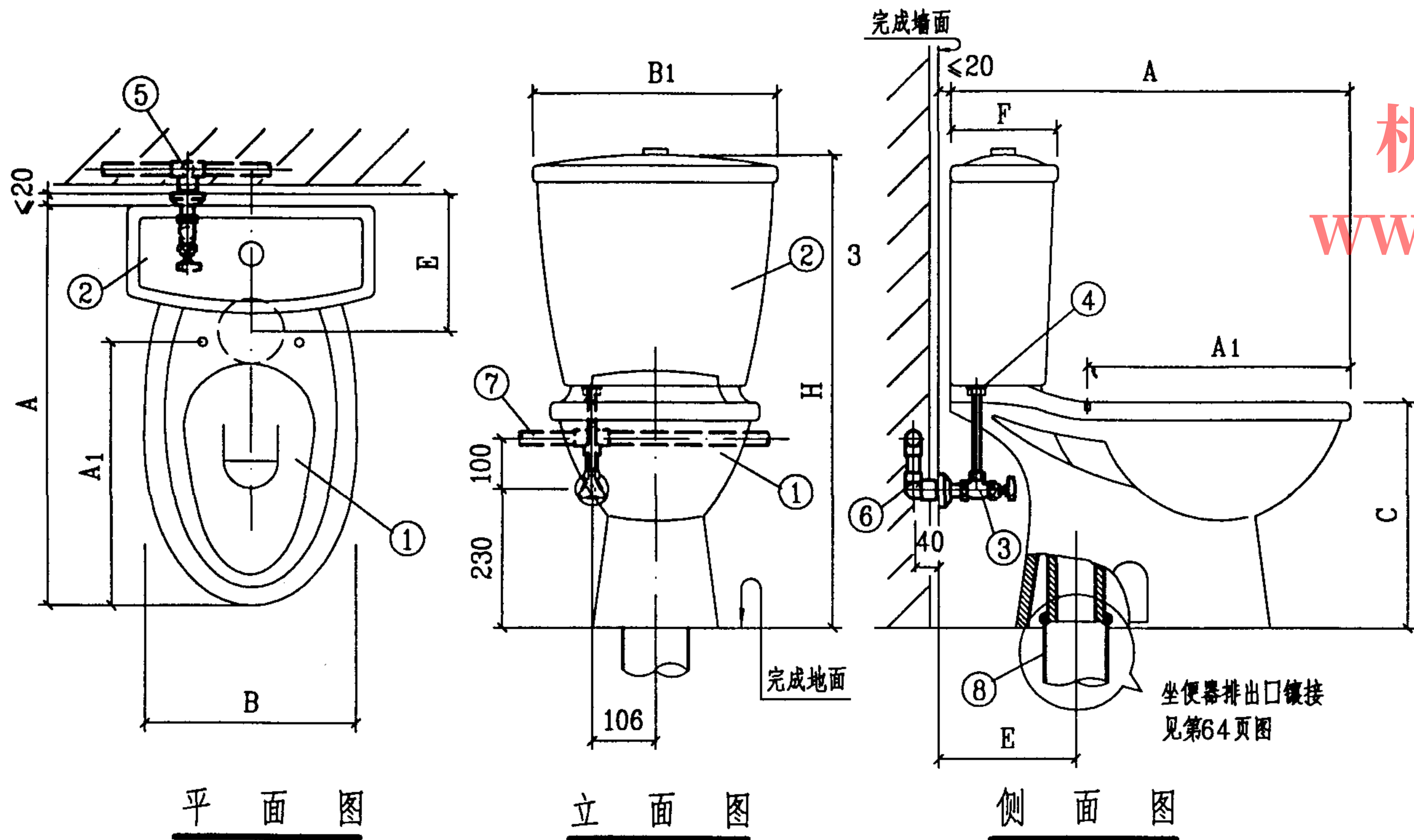
坐箱式坐便器尺寸表
