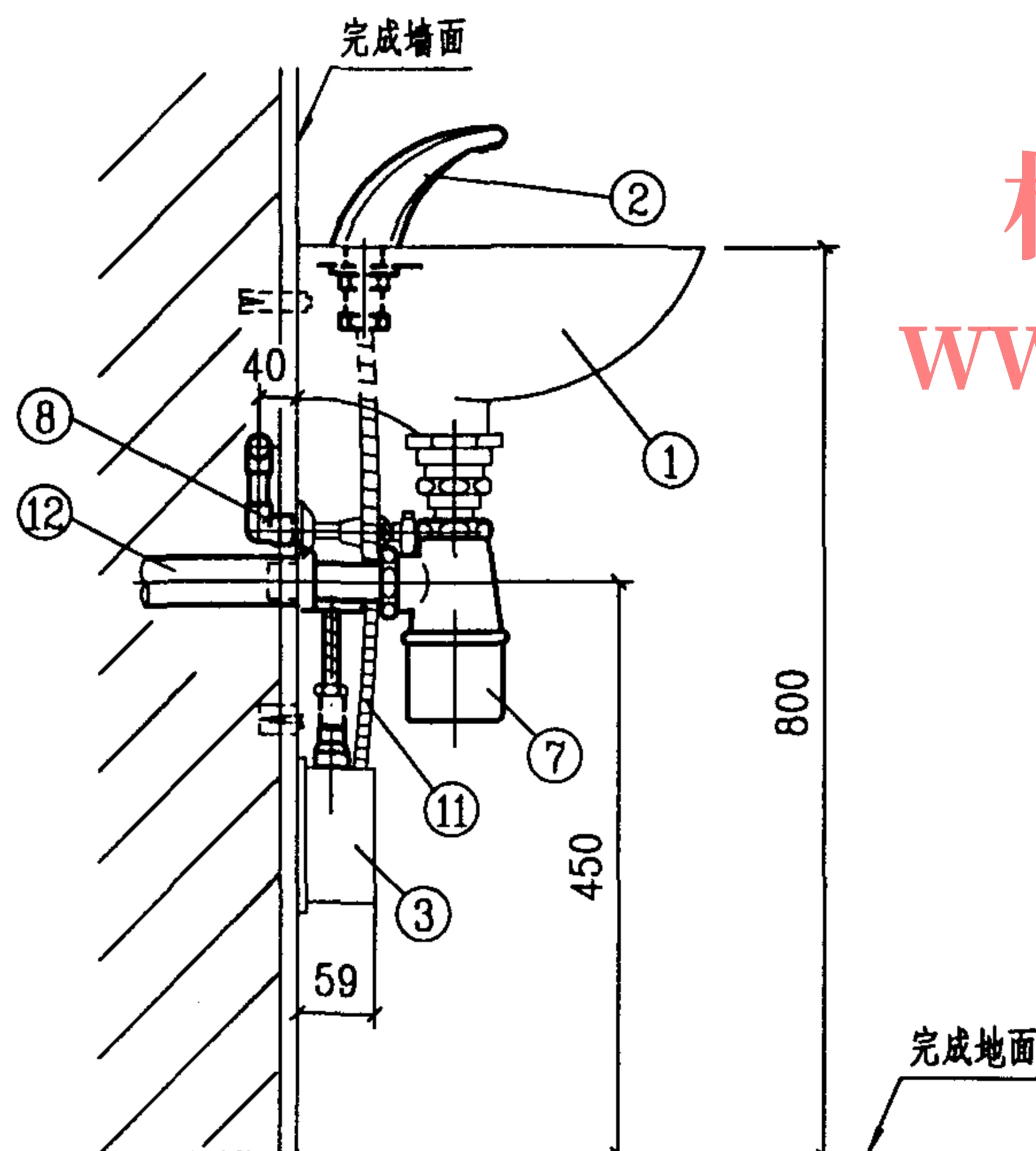
侧面图
