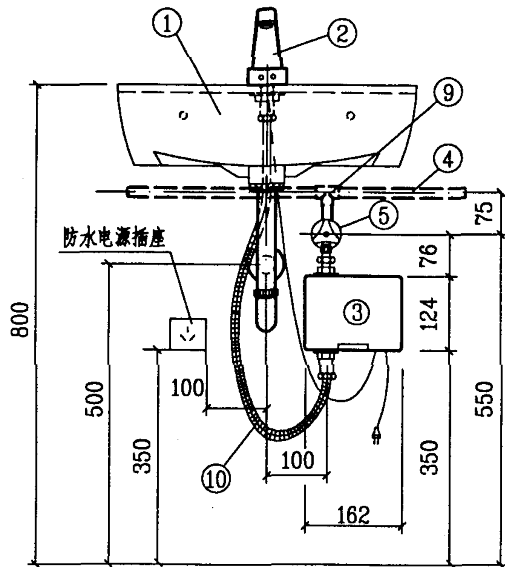
立面图
