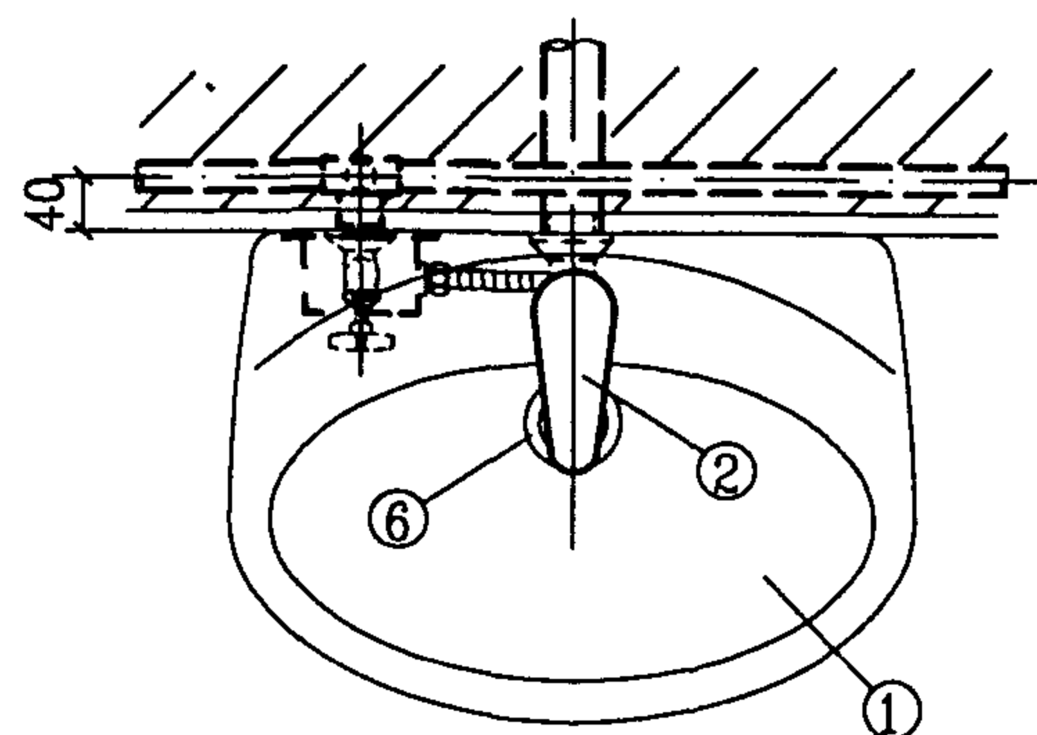
平面图
