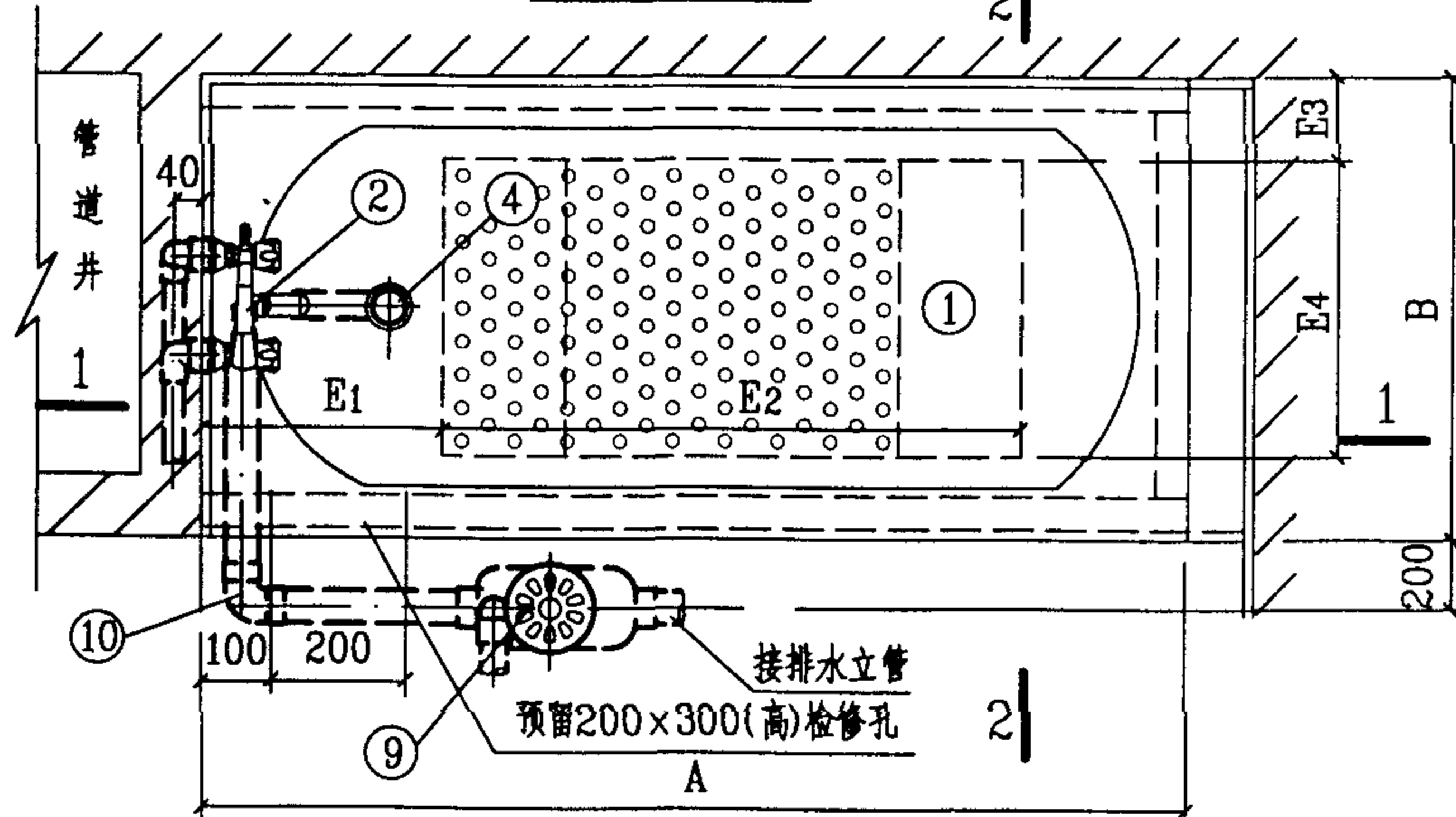
平面图
