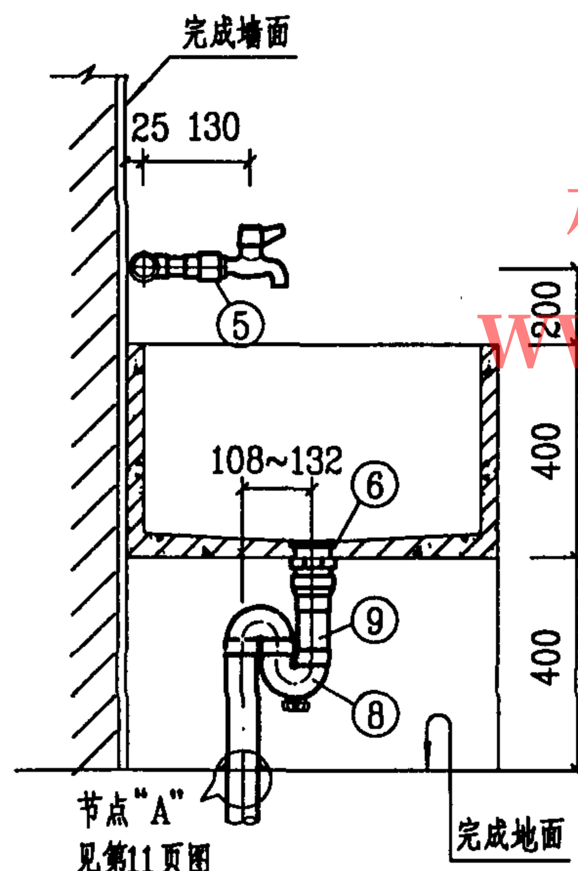
3-3剖面图
