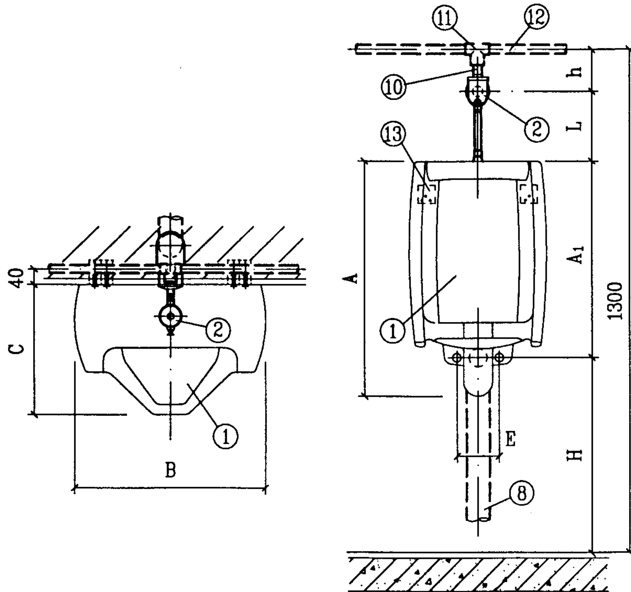
平面图
