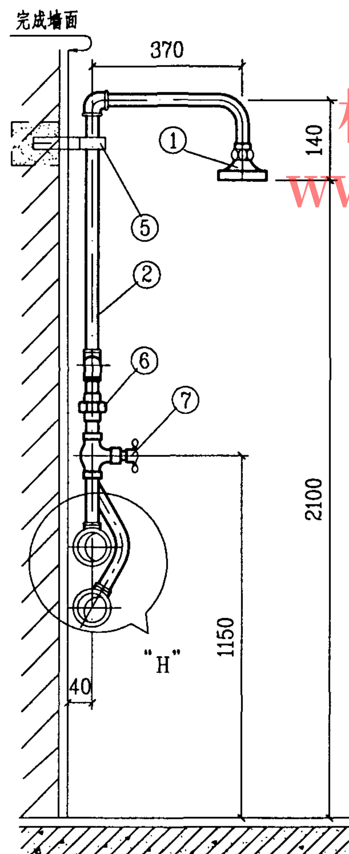
侧面图
