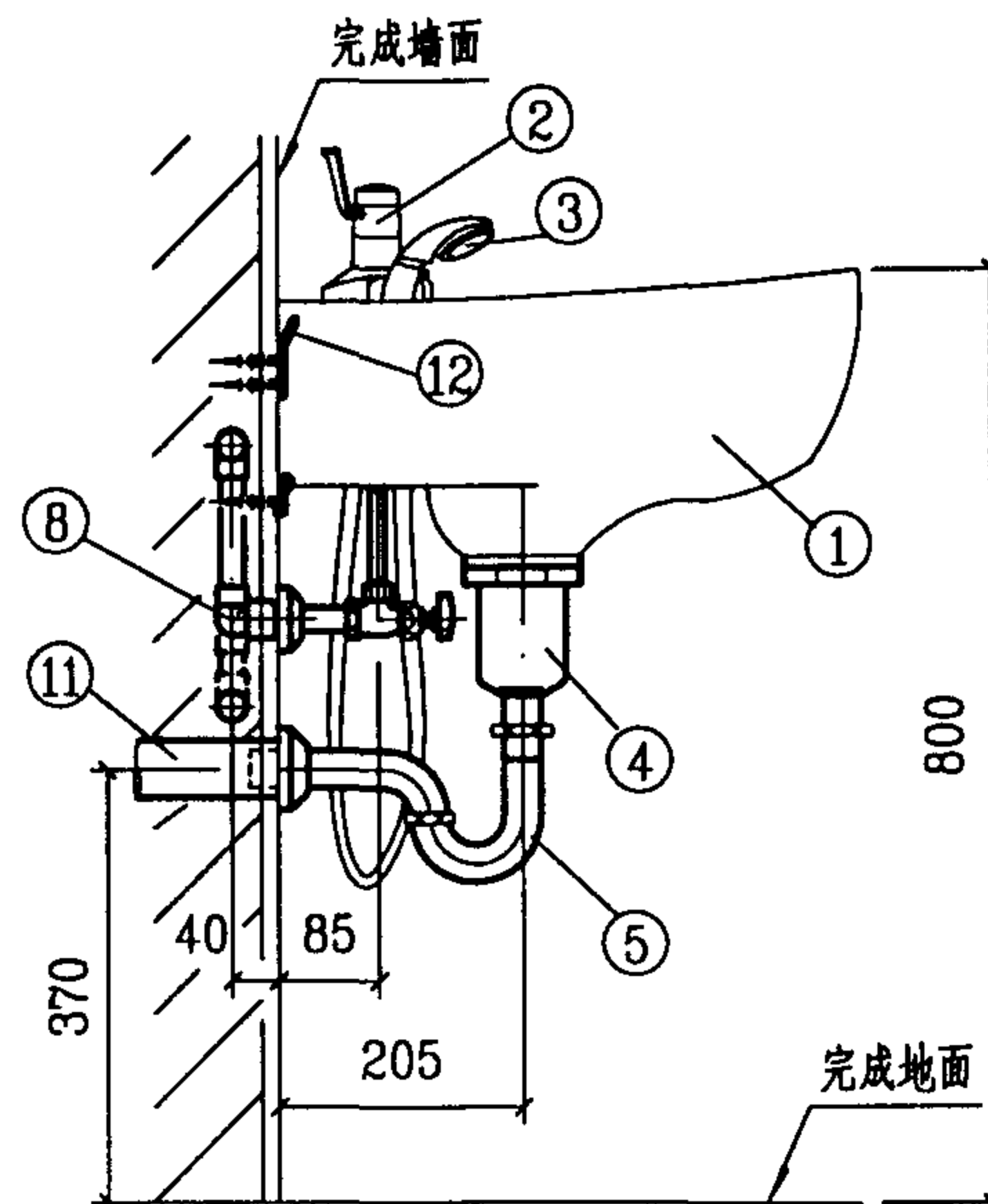
侧面图
