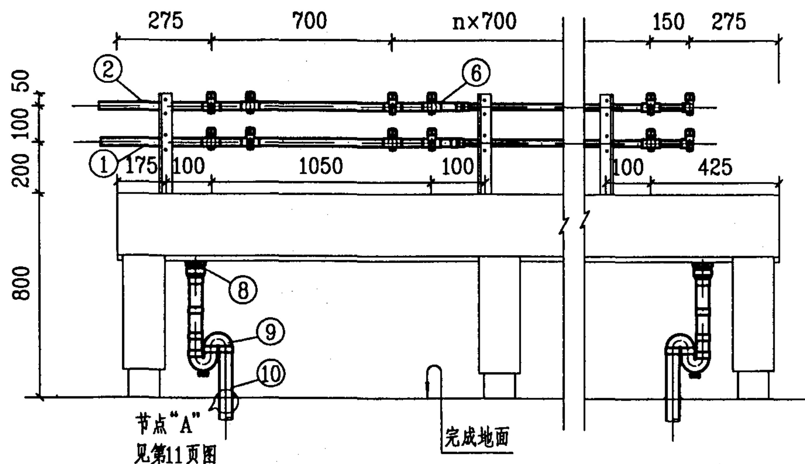
立面图
