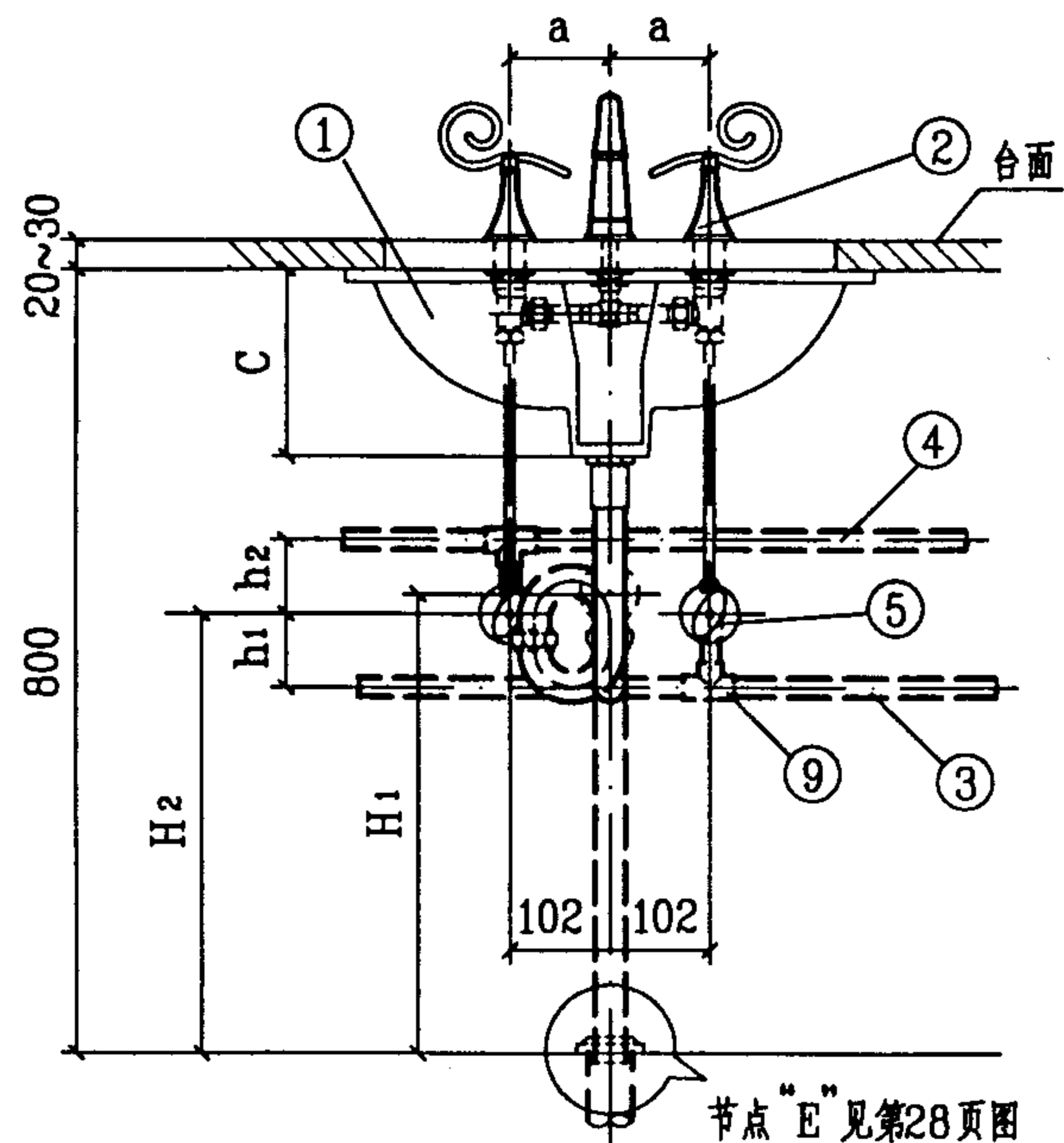
1-1 剖面图
