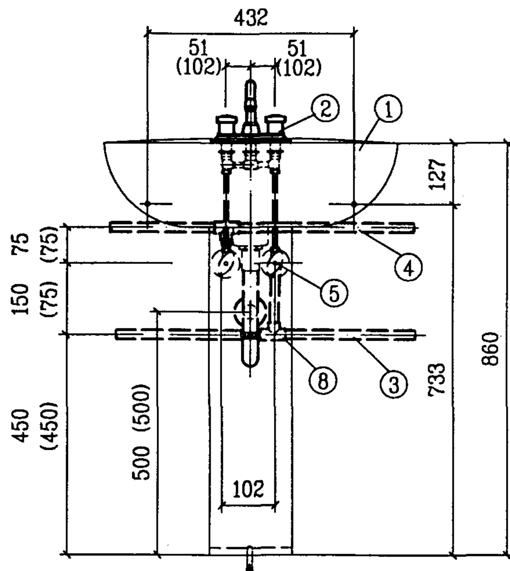
立面图
