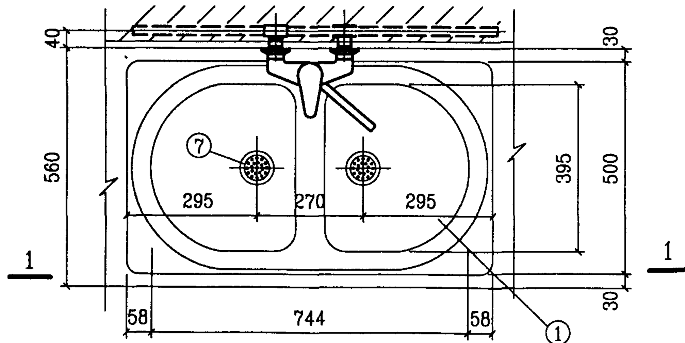
平面图
