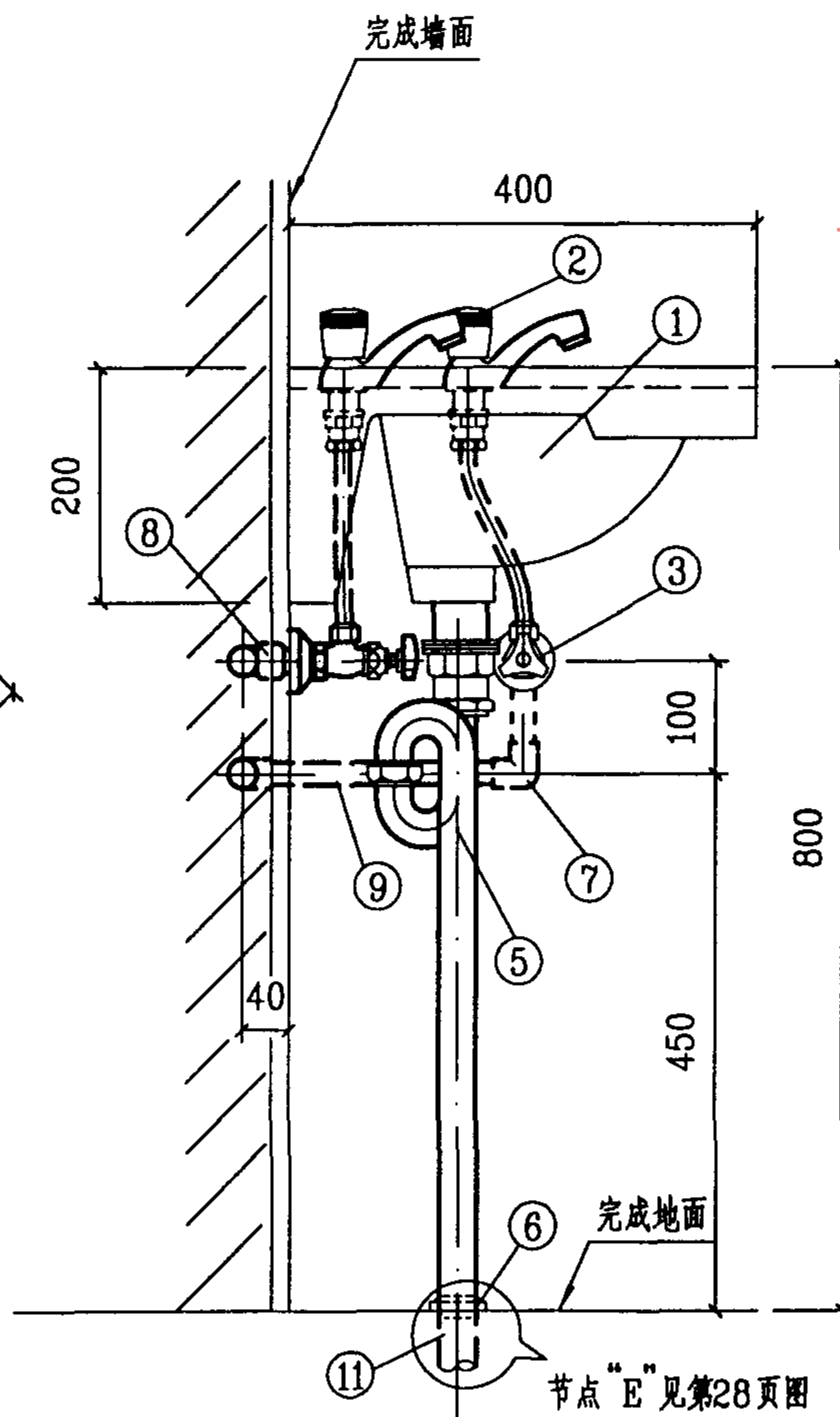
立面图
