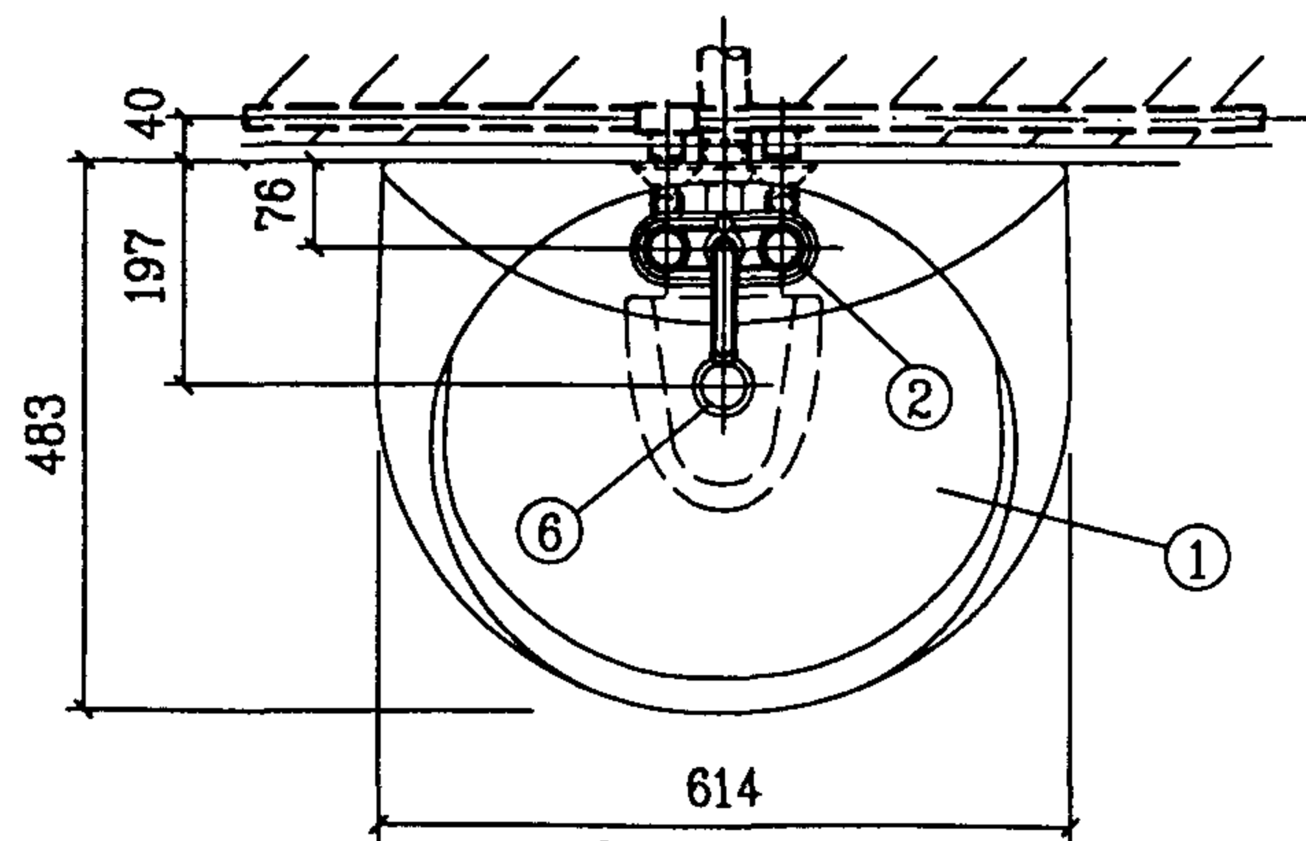
平面图
