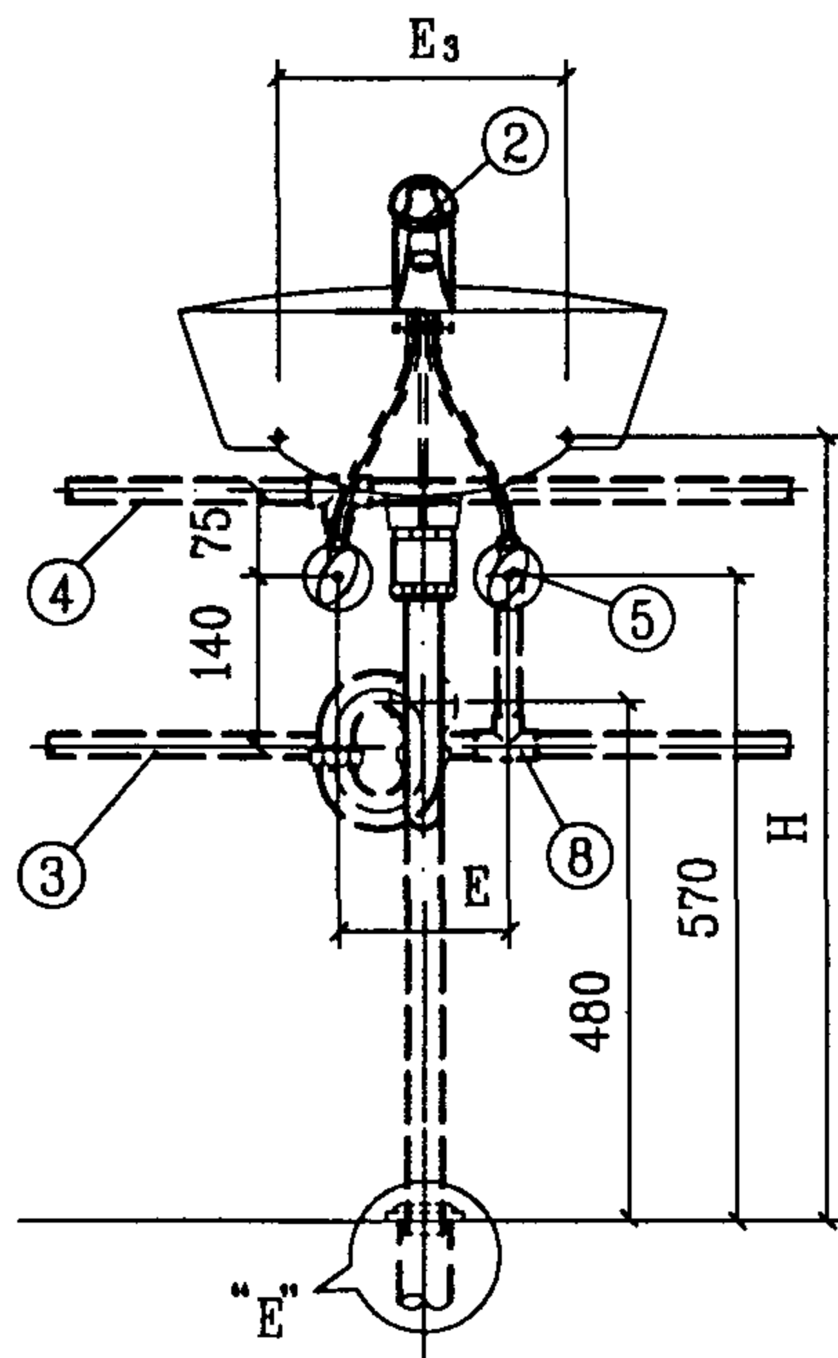
立面图
