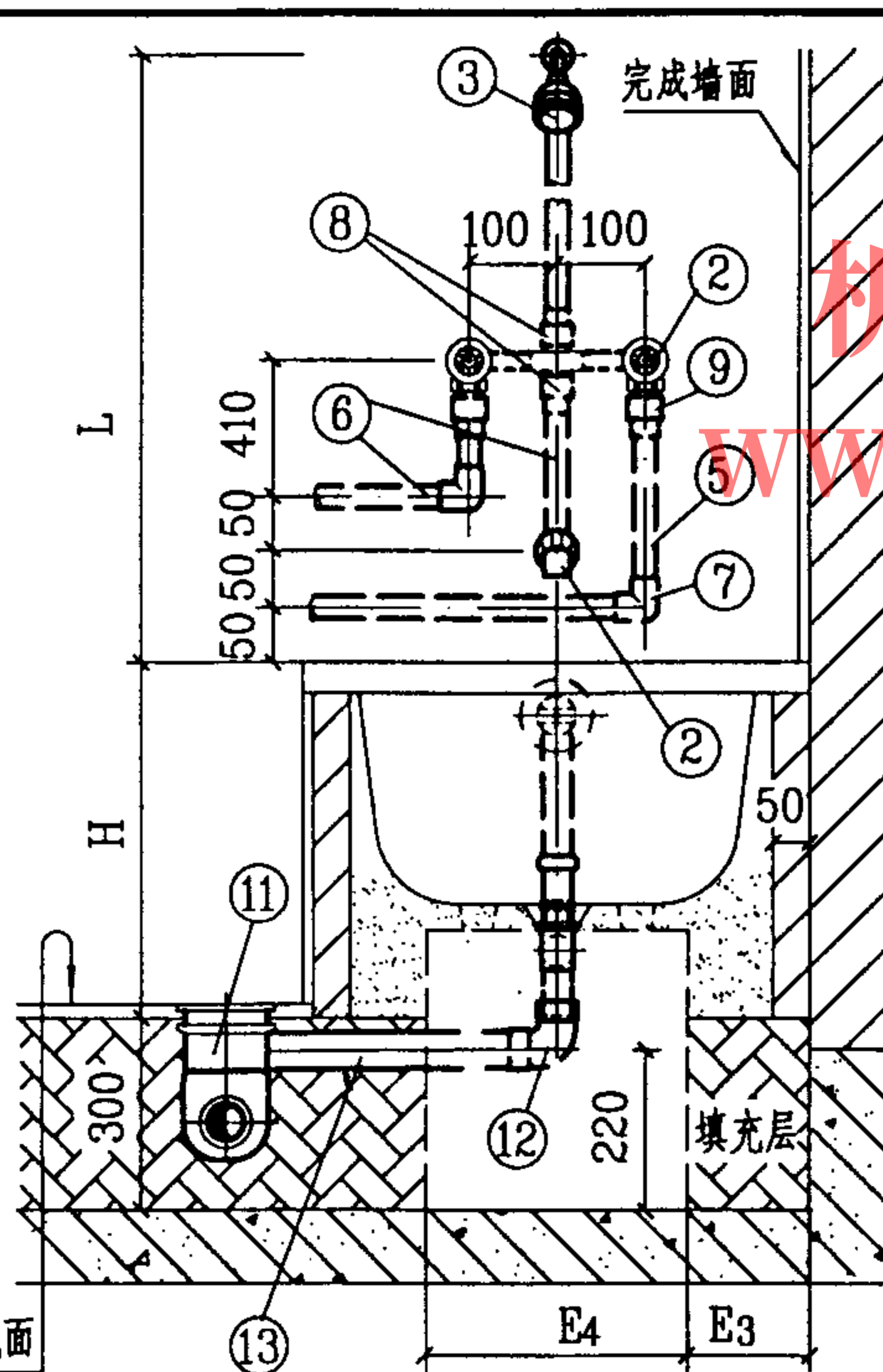
2-2 剖面图
