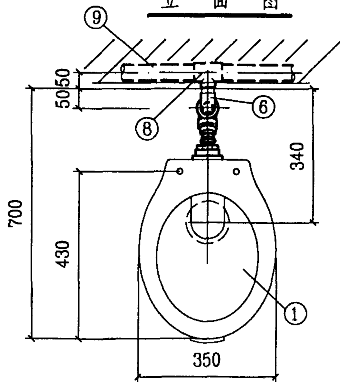
平面图
