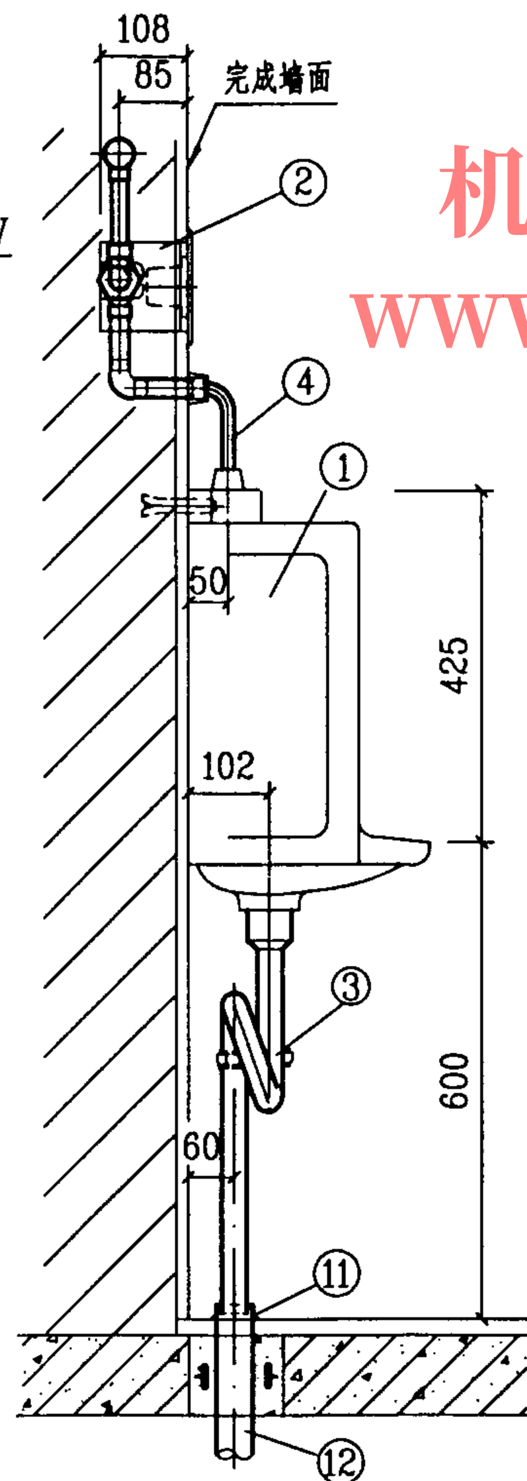
侧面图
