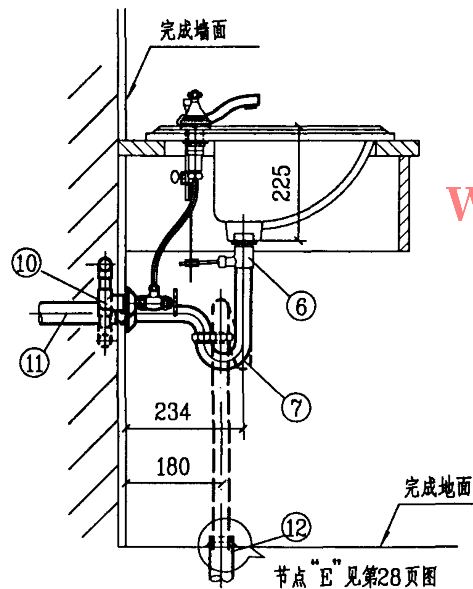
2-2 剖面图
