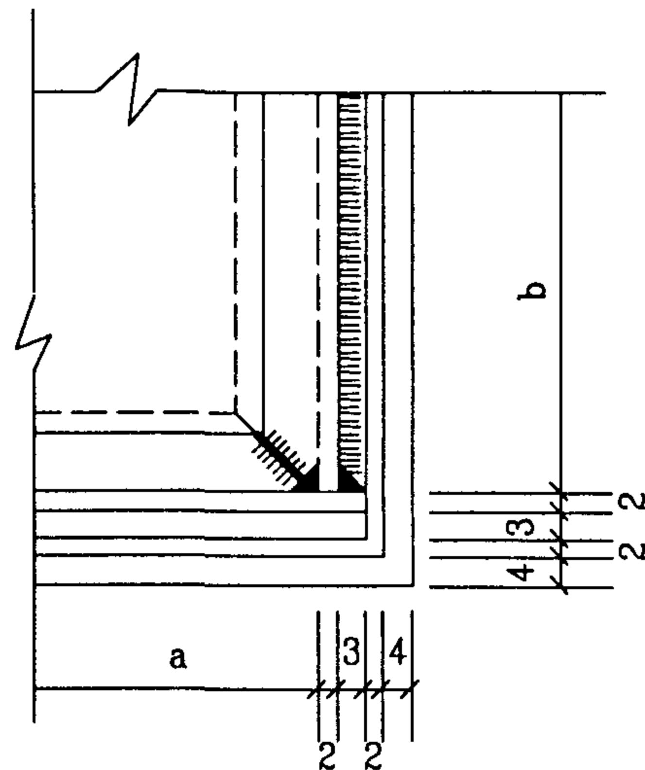
节点“Ⅰ”
