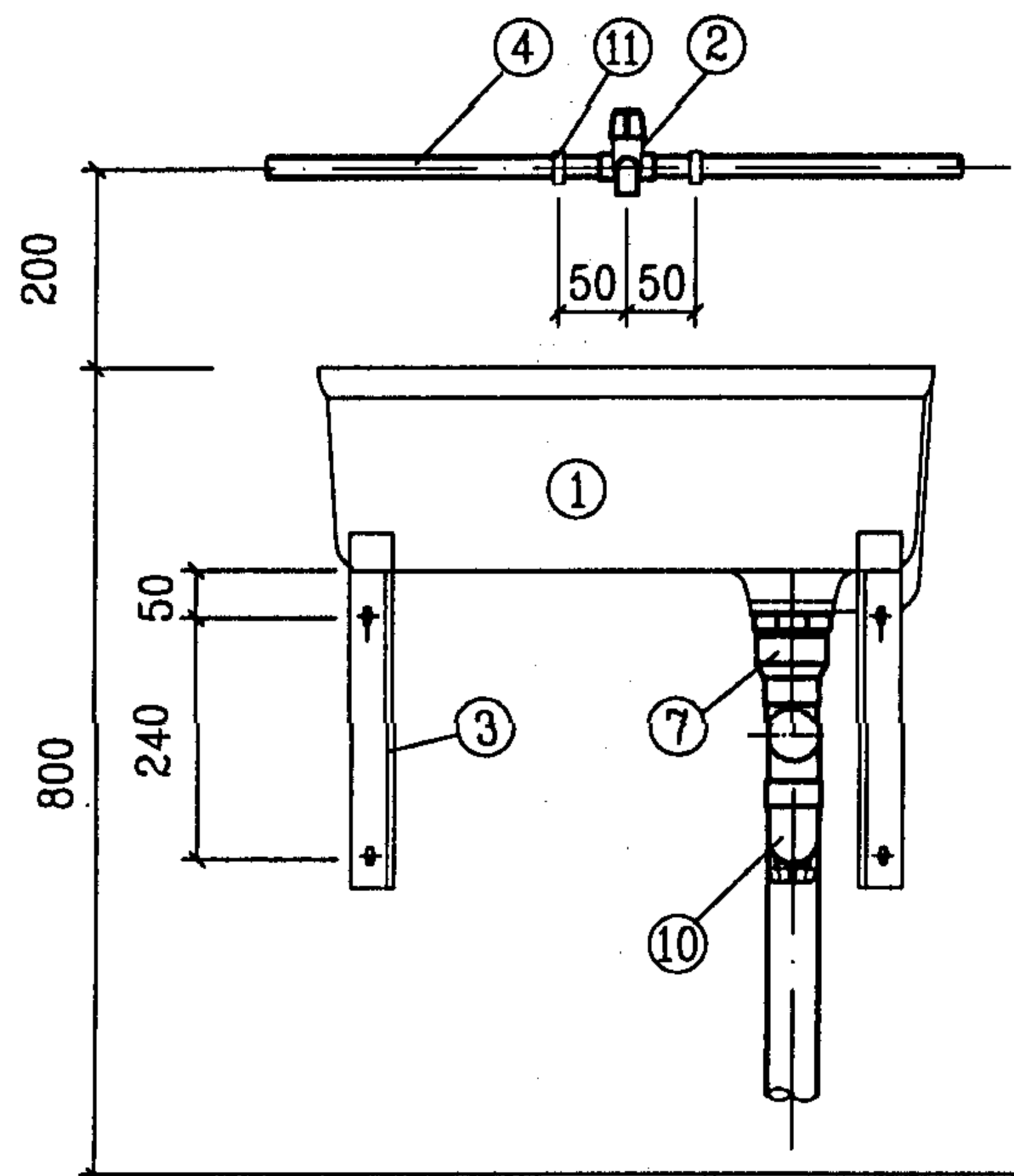
立面图
