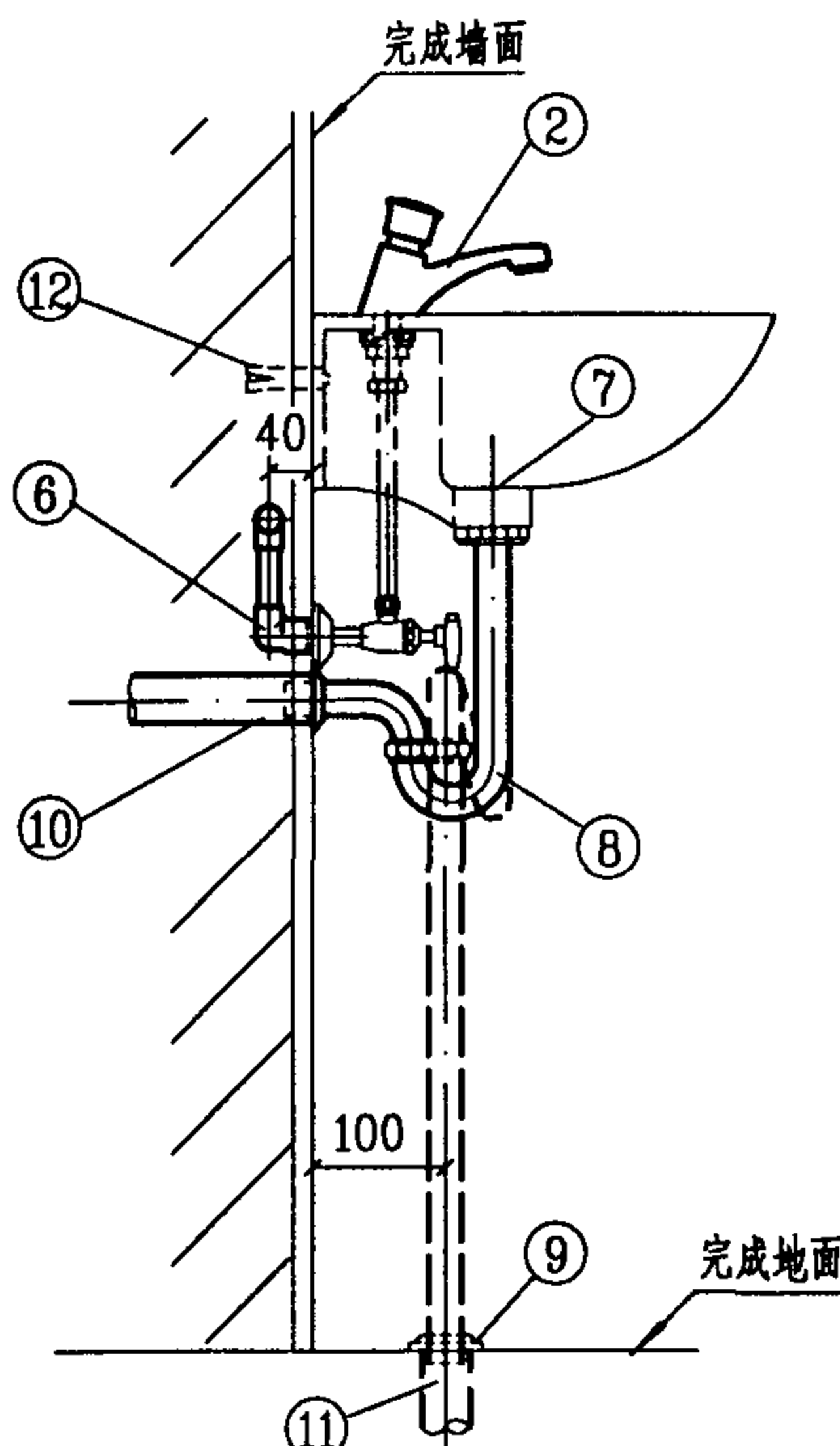
侧面图
