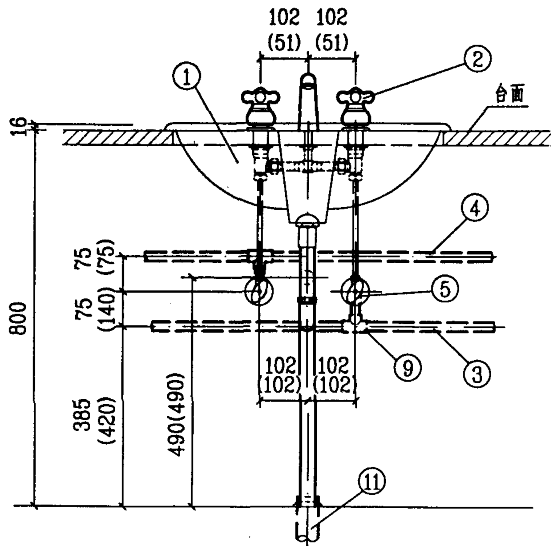
1-1 剖面图
