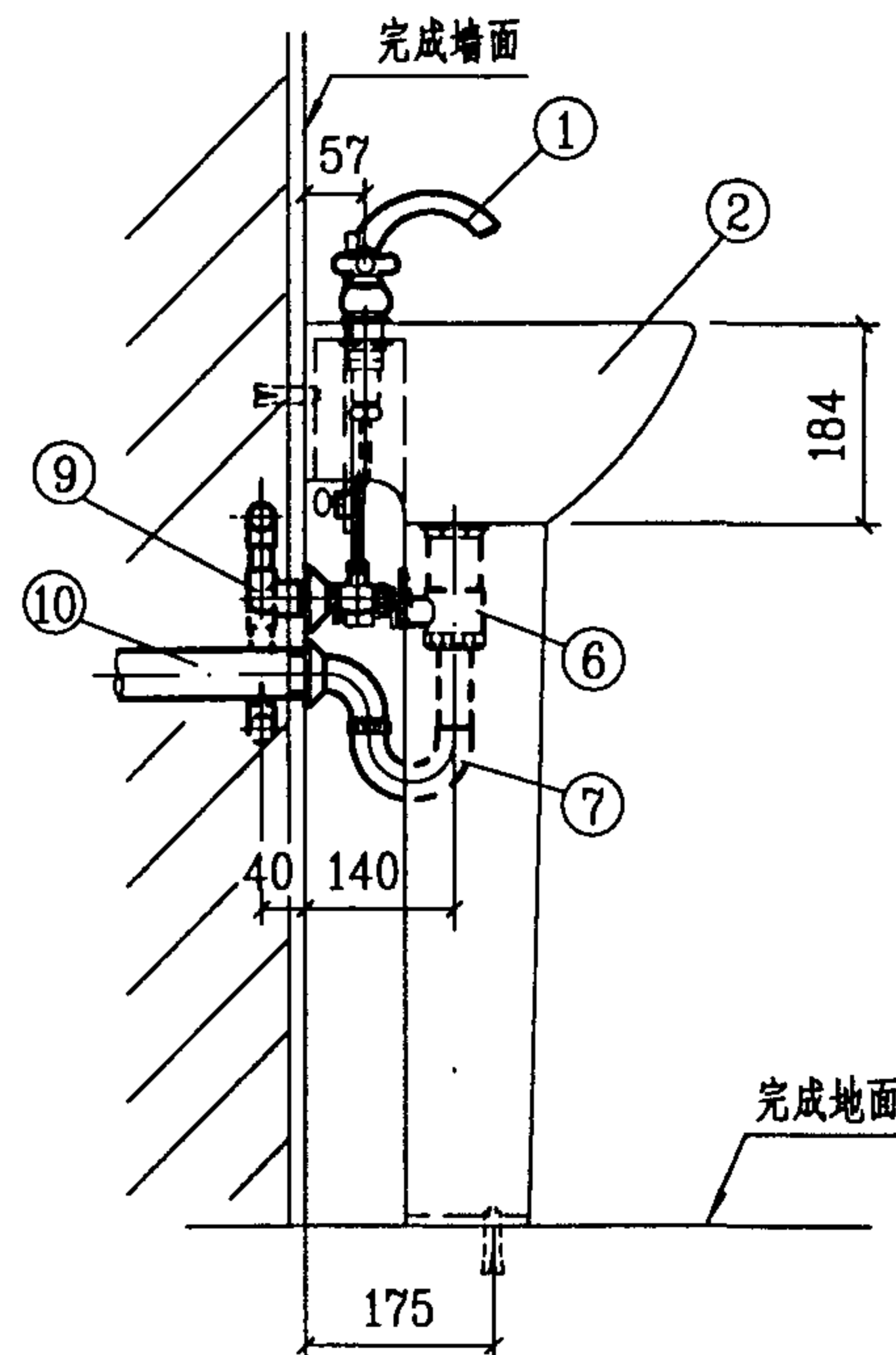
侧面图
