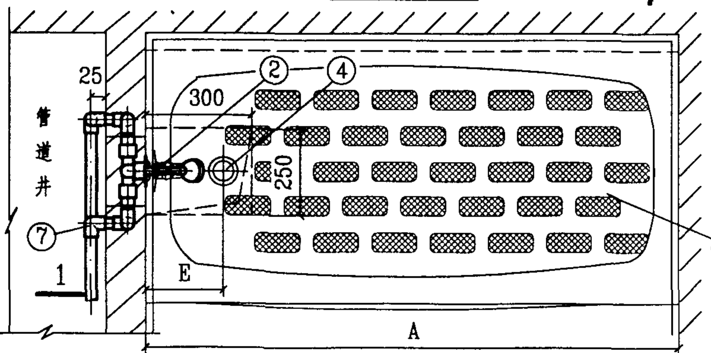
平面图
