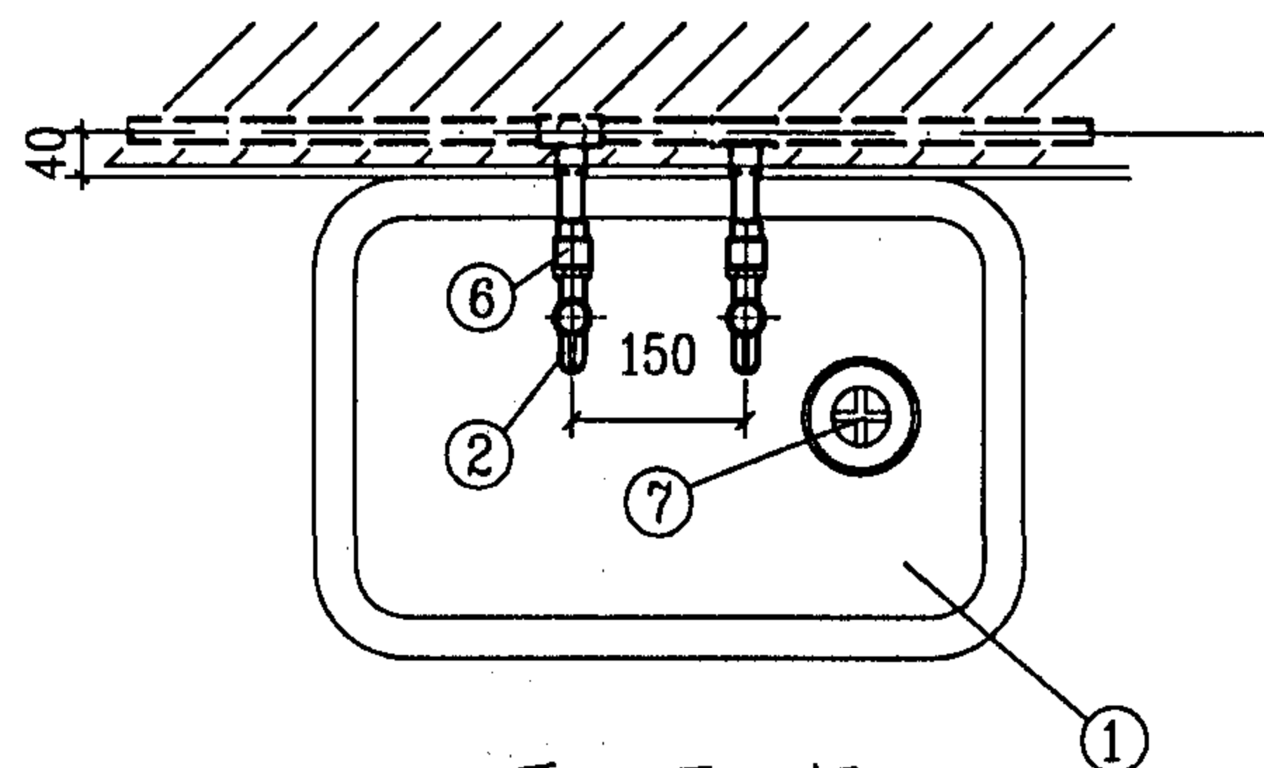
平面图
