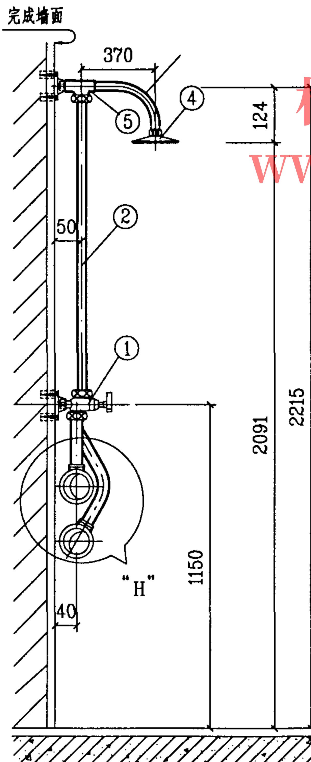
侧面图
