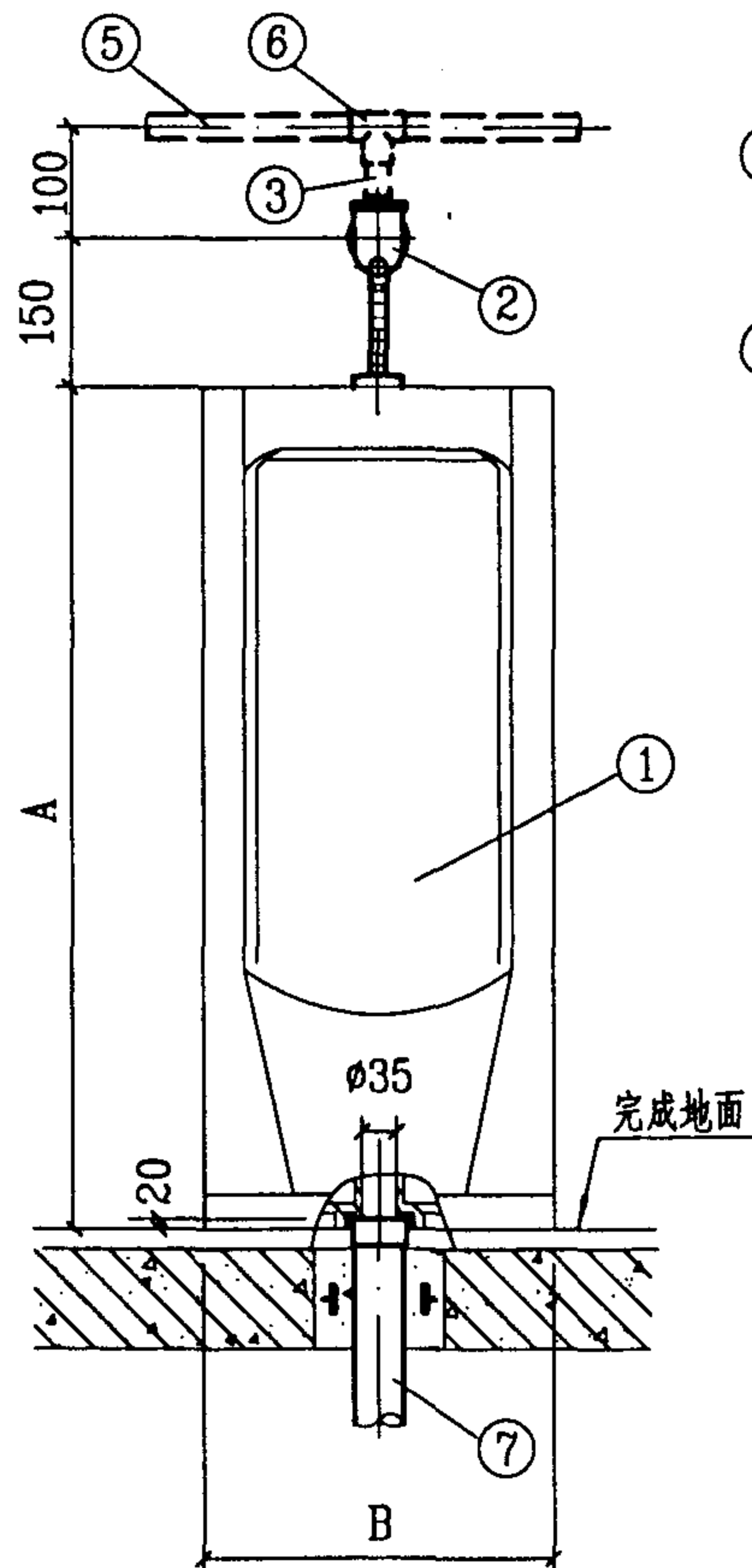
立面图
