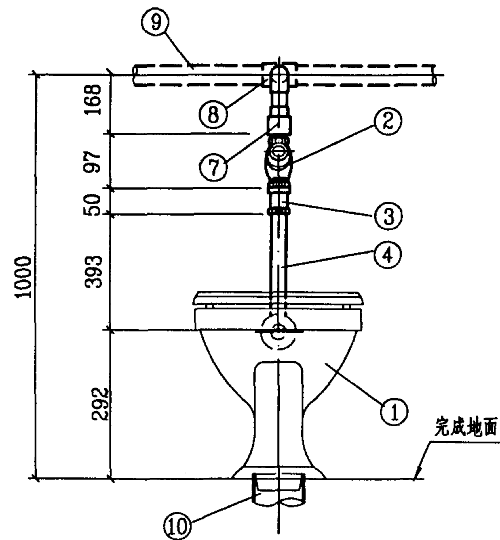
立面图
