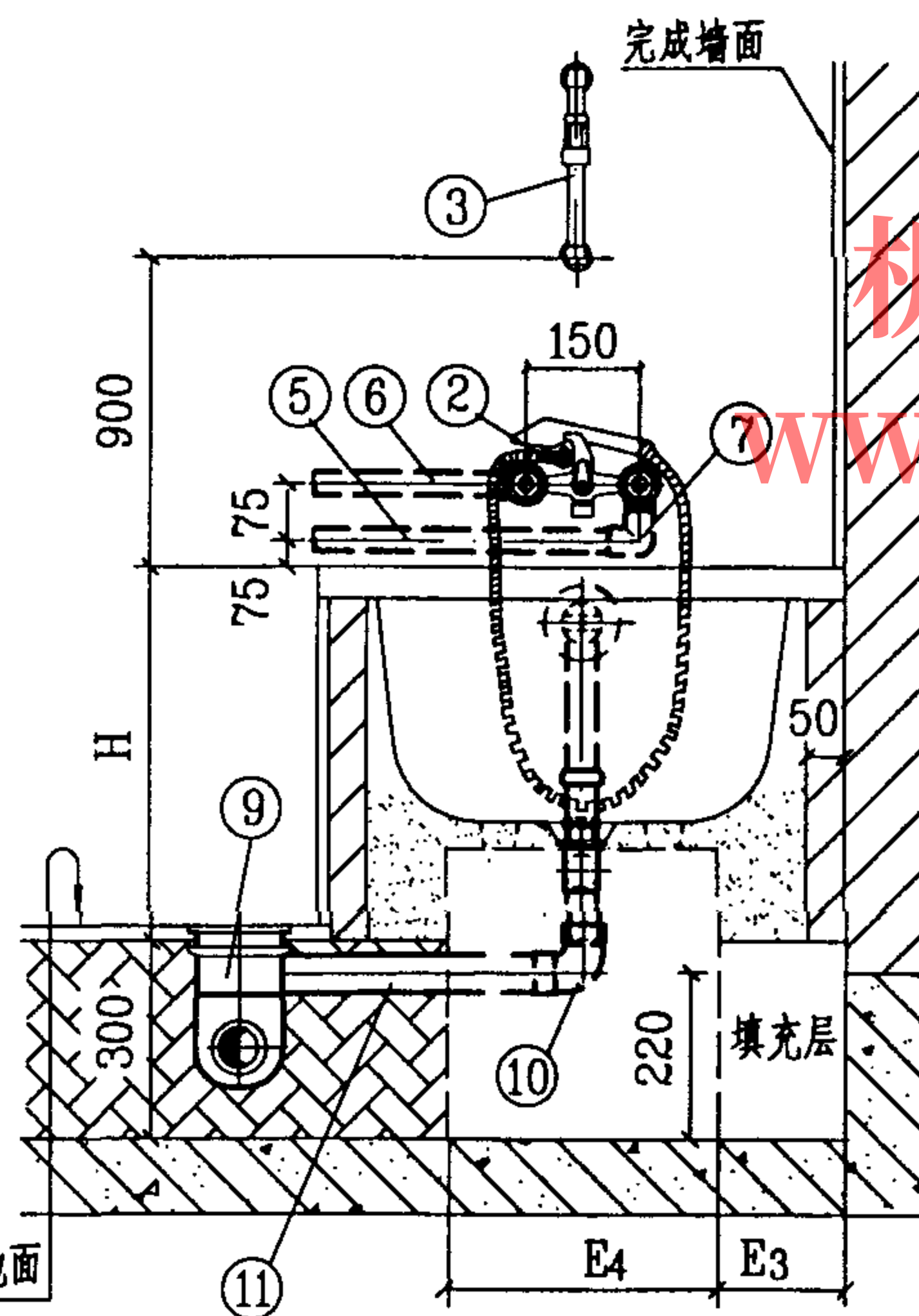
2-2 剖面图
