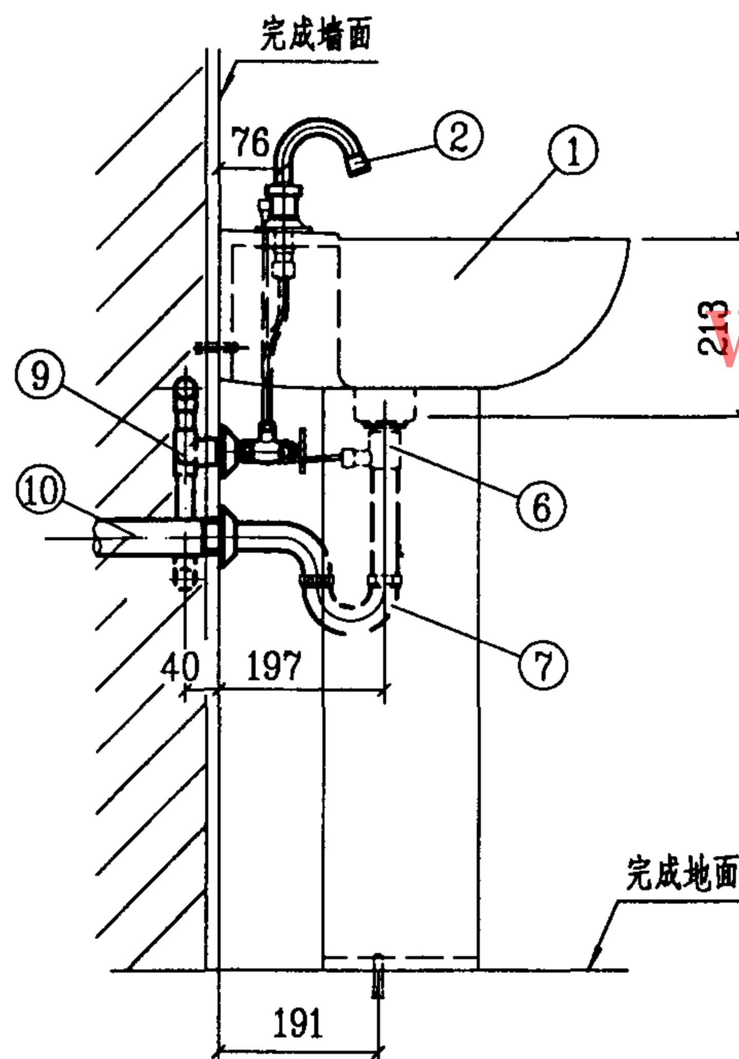
侧面图
