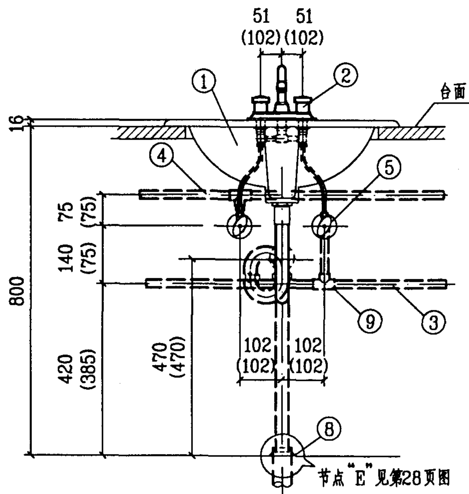
1-1 剖面图
