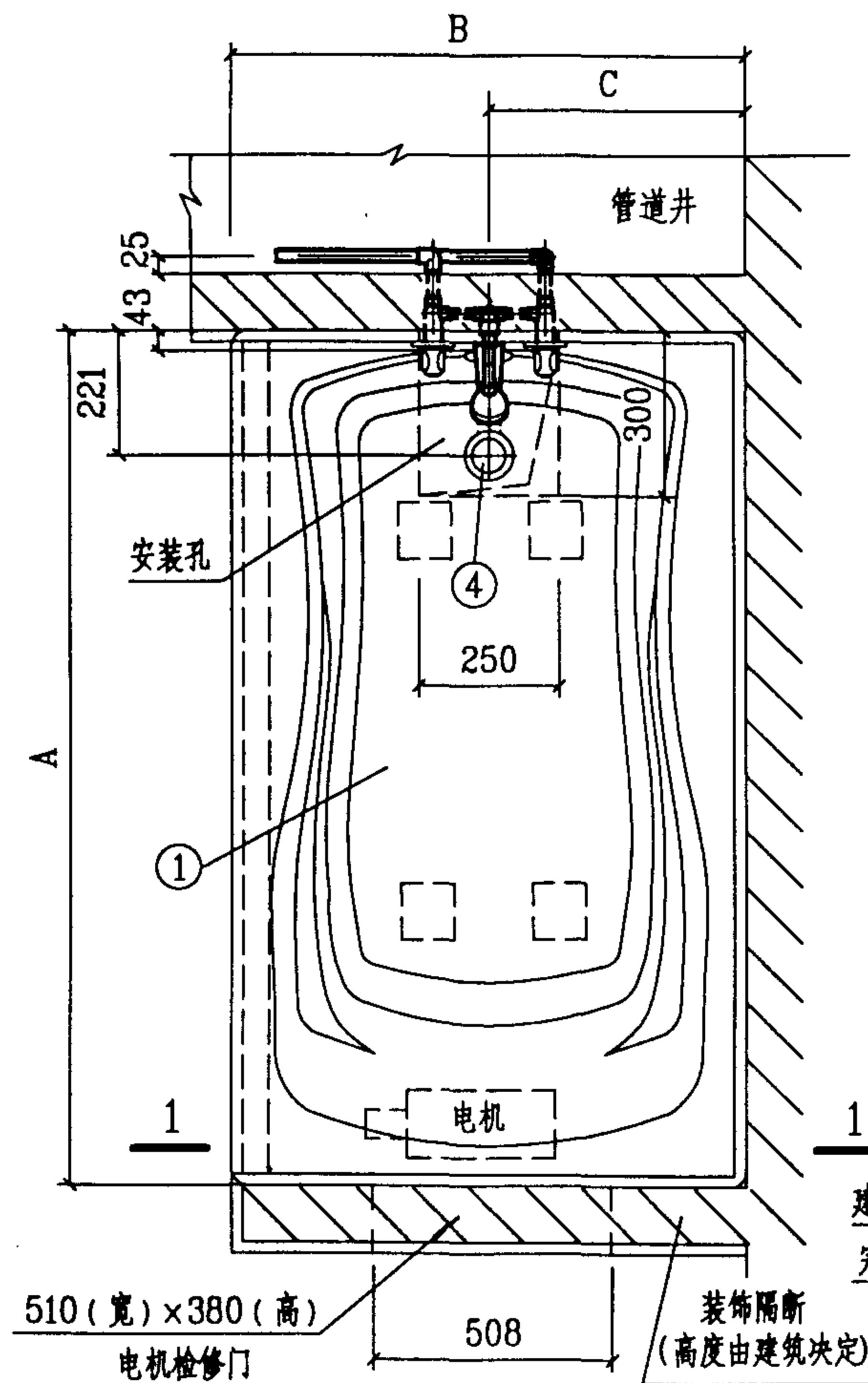
平面图
