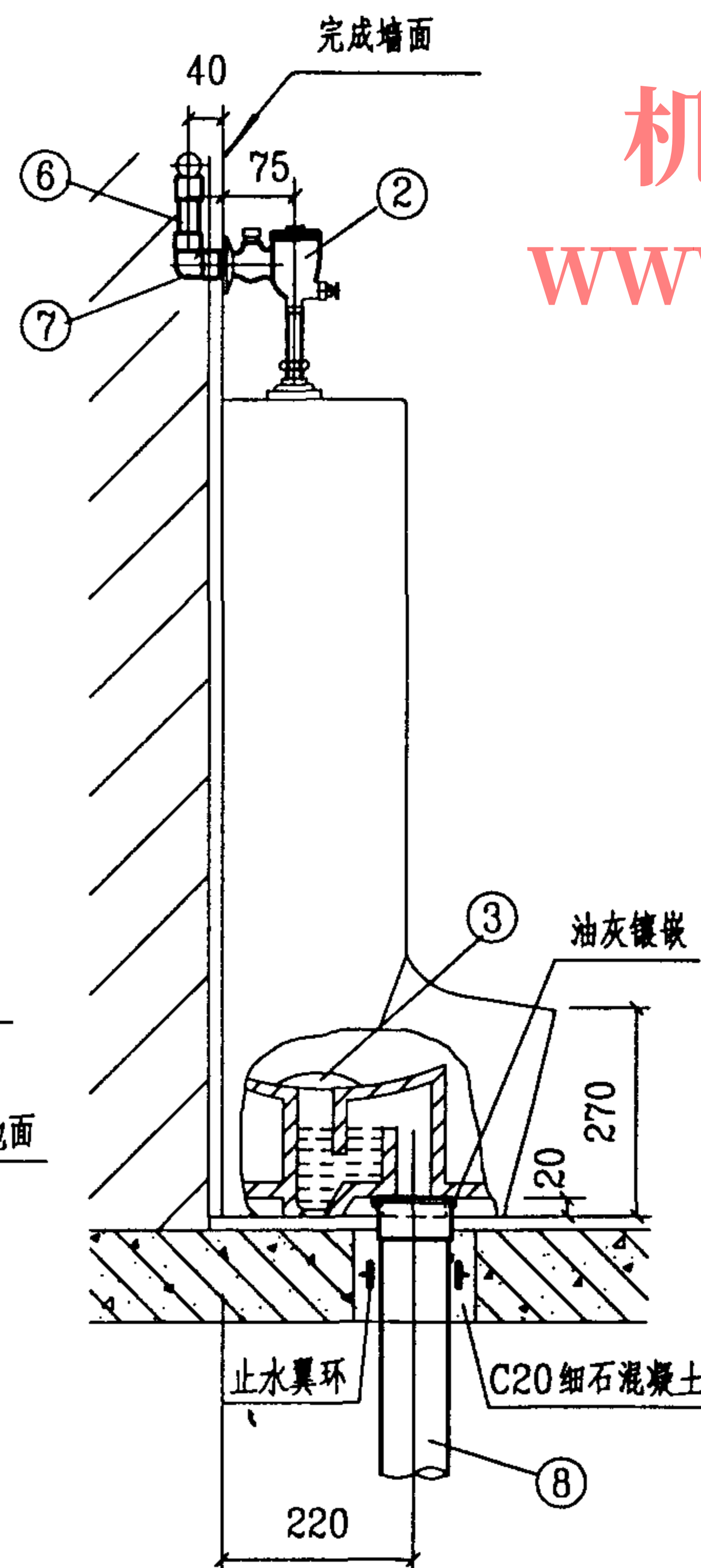
侧面图
