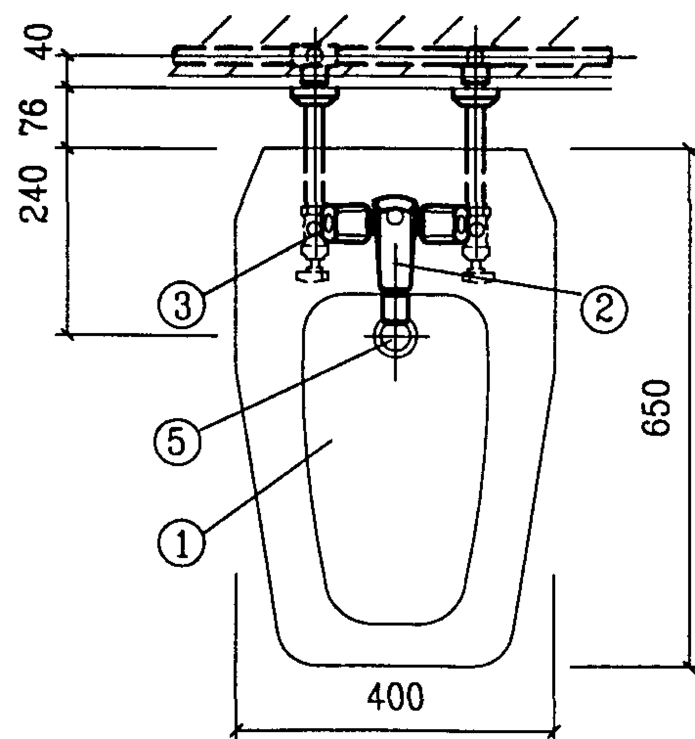
平面图
