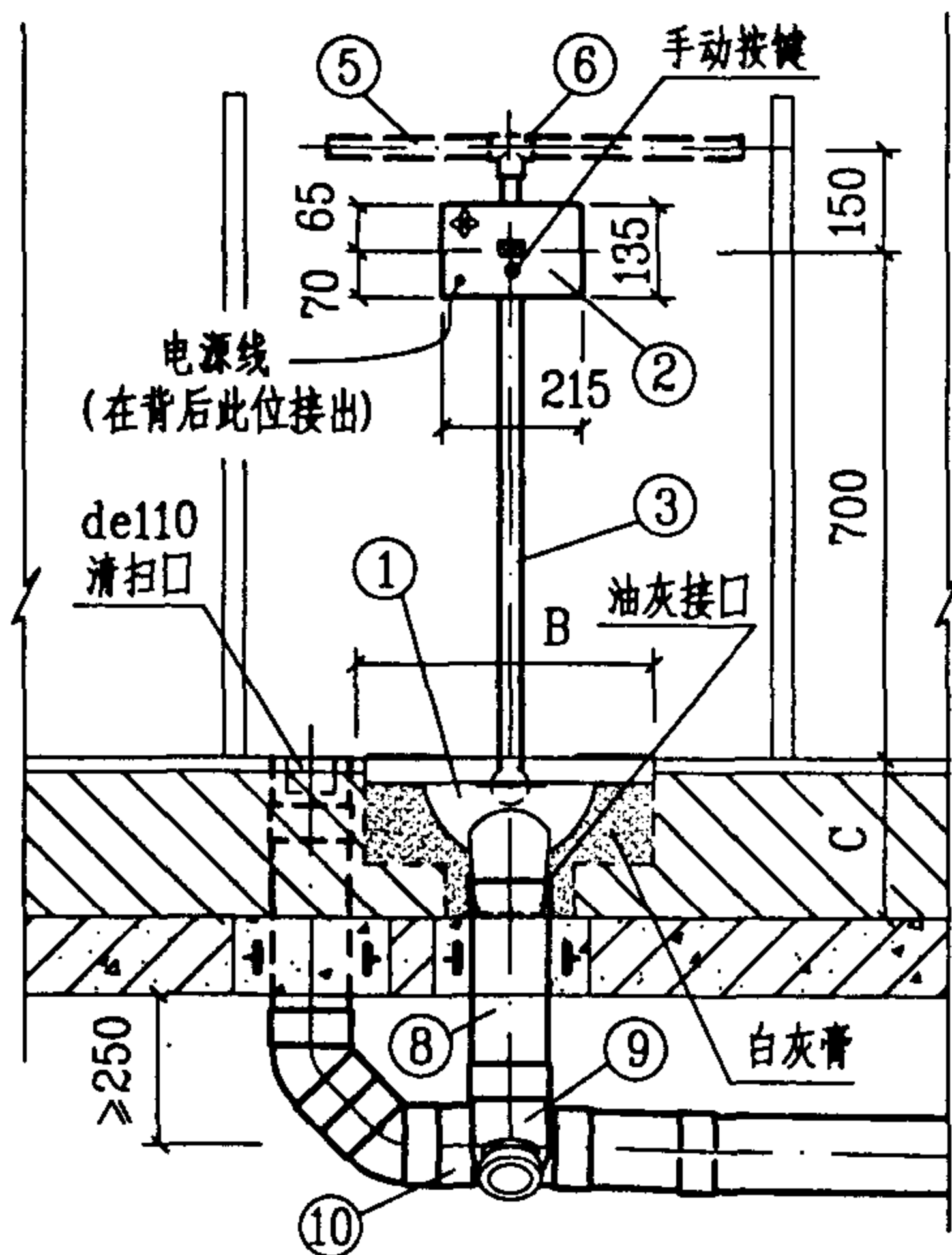
1-1 剖面图
