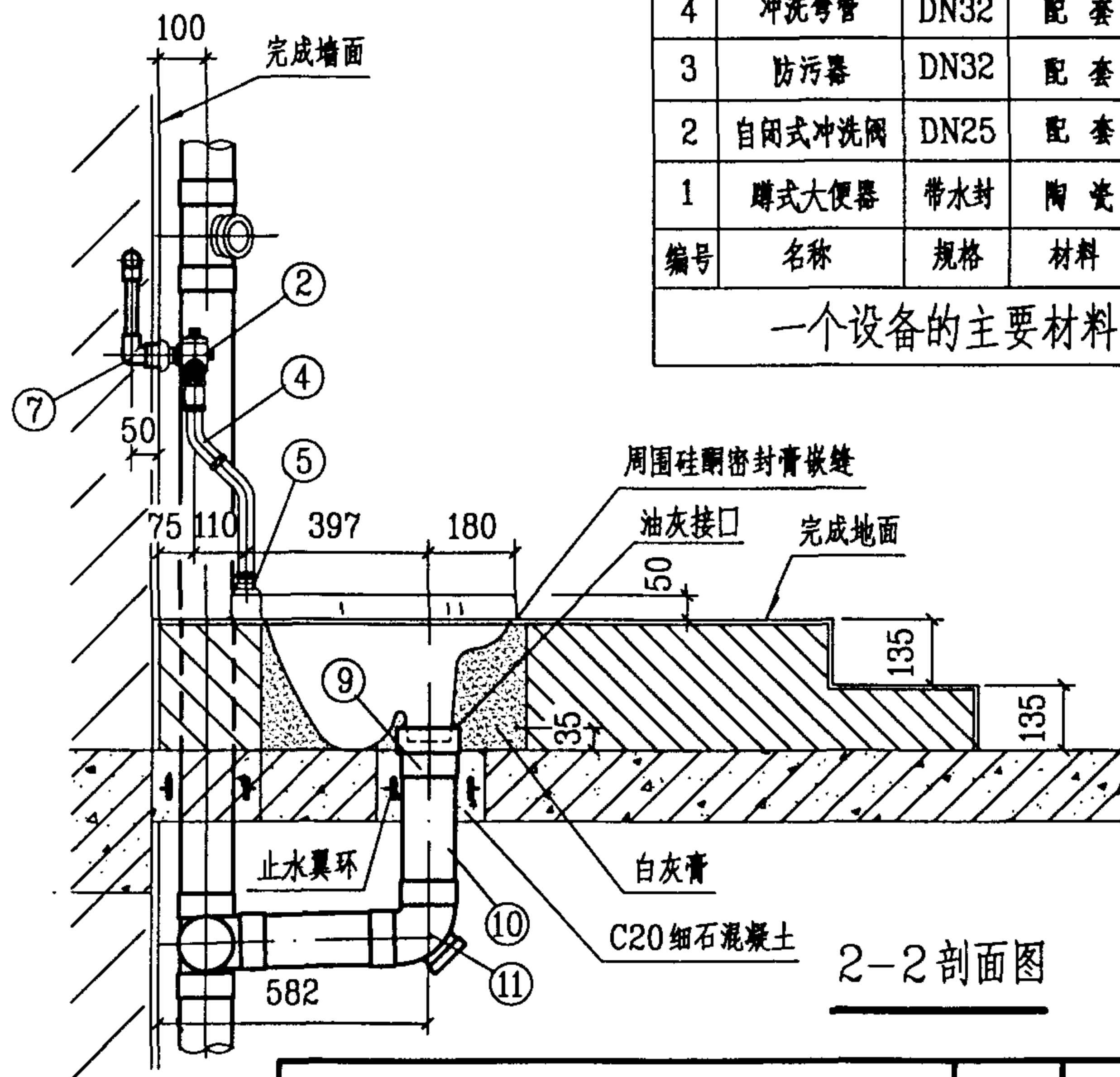
自闭式冲洗阀蹲式大便器安装图(三)
