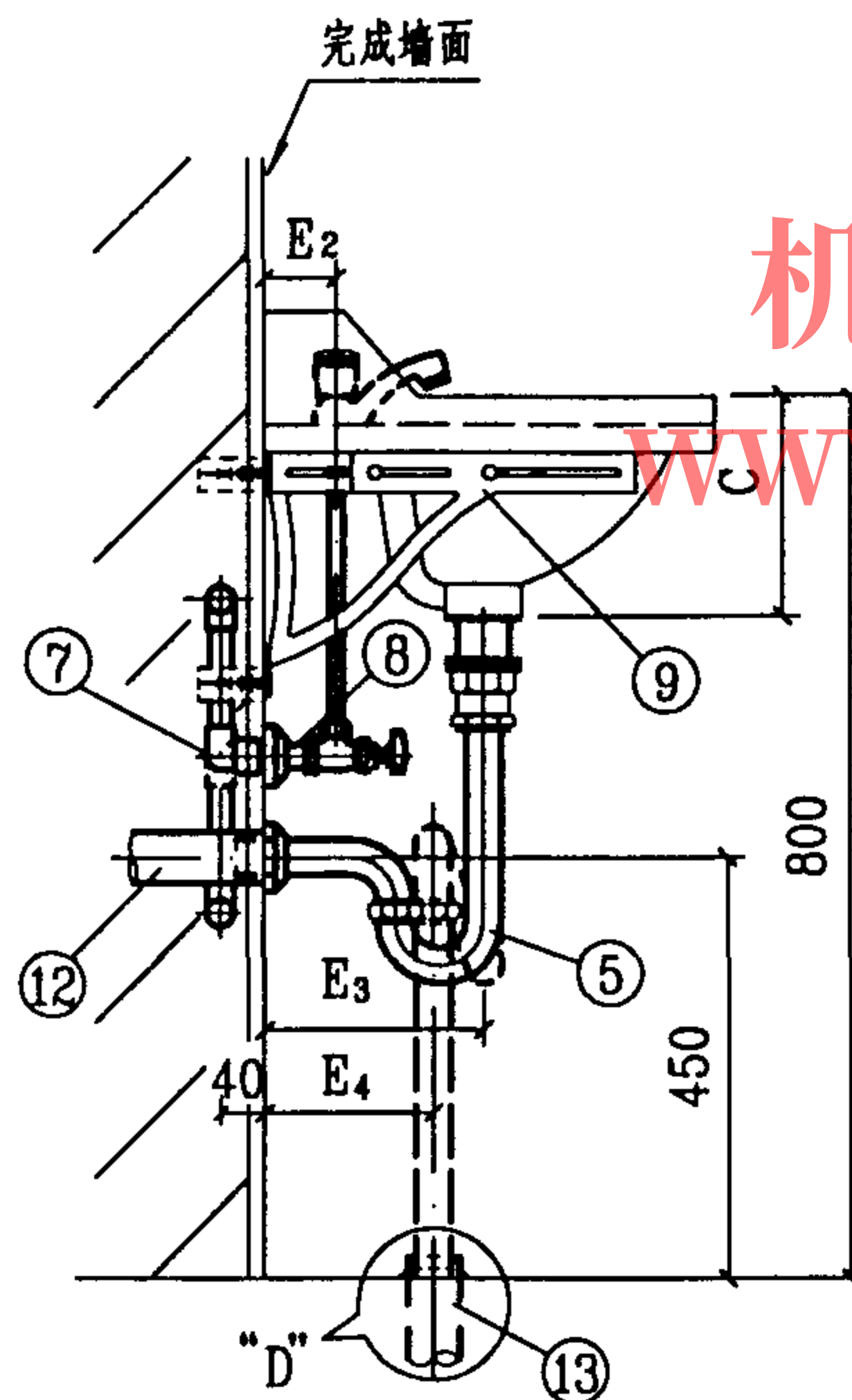
侧面图
