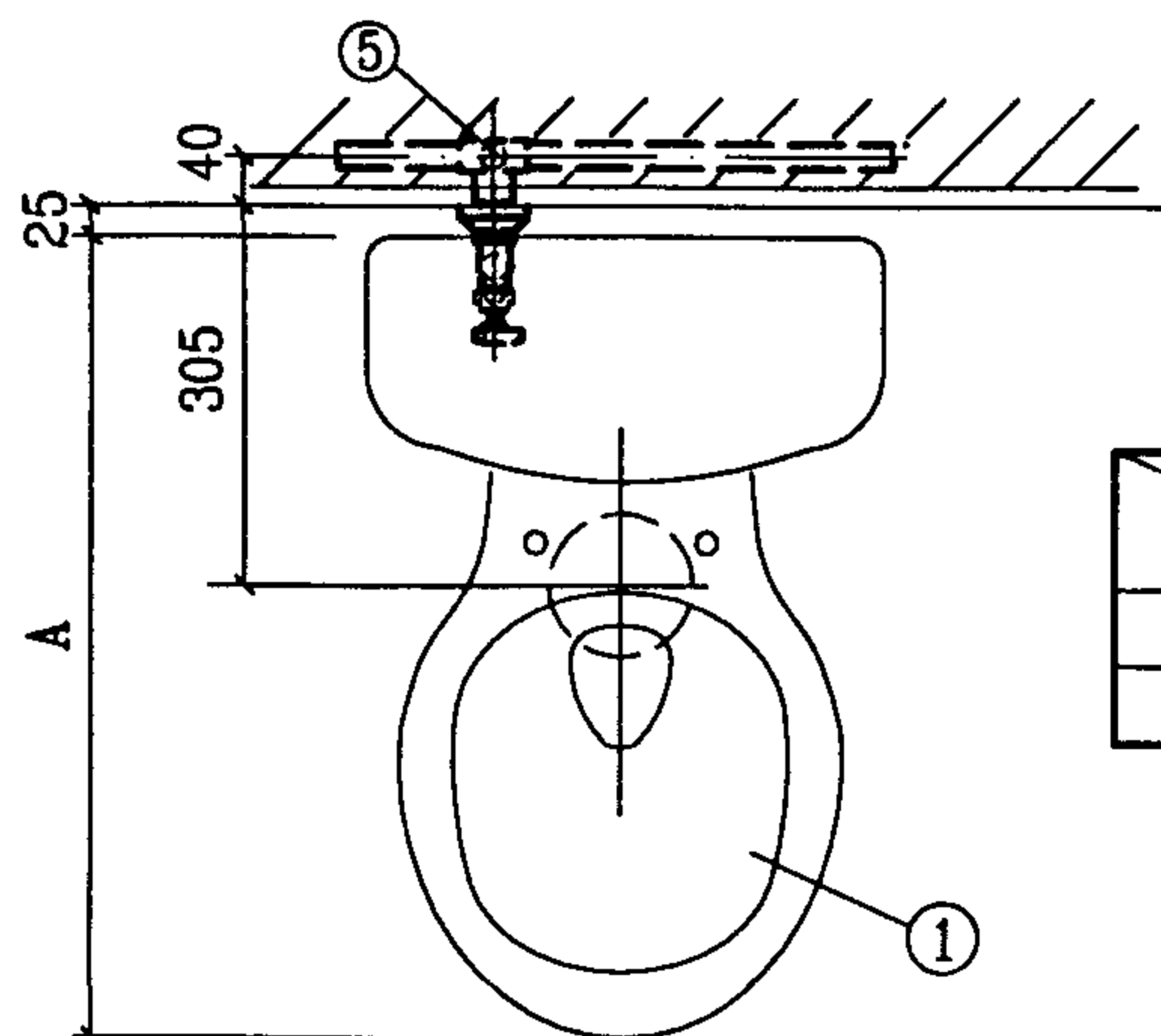
平面图
