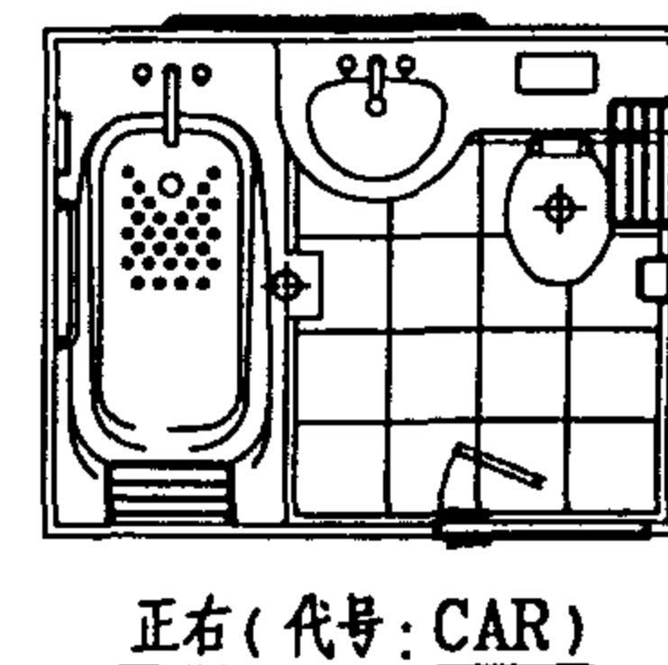
整体卫生间 BU1620C 型平面图
