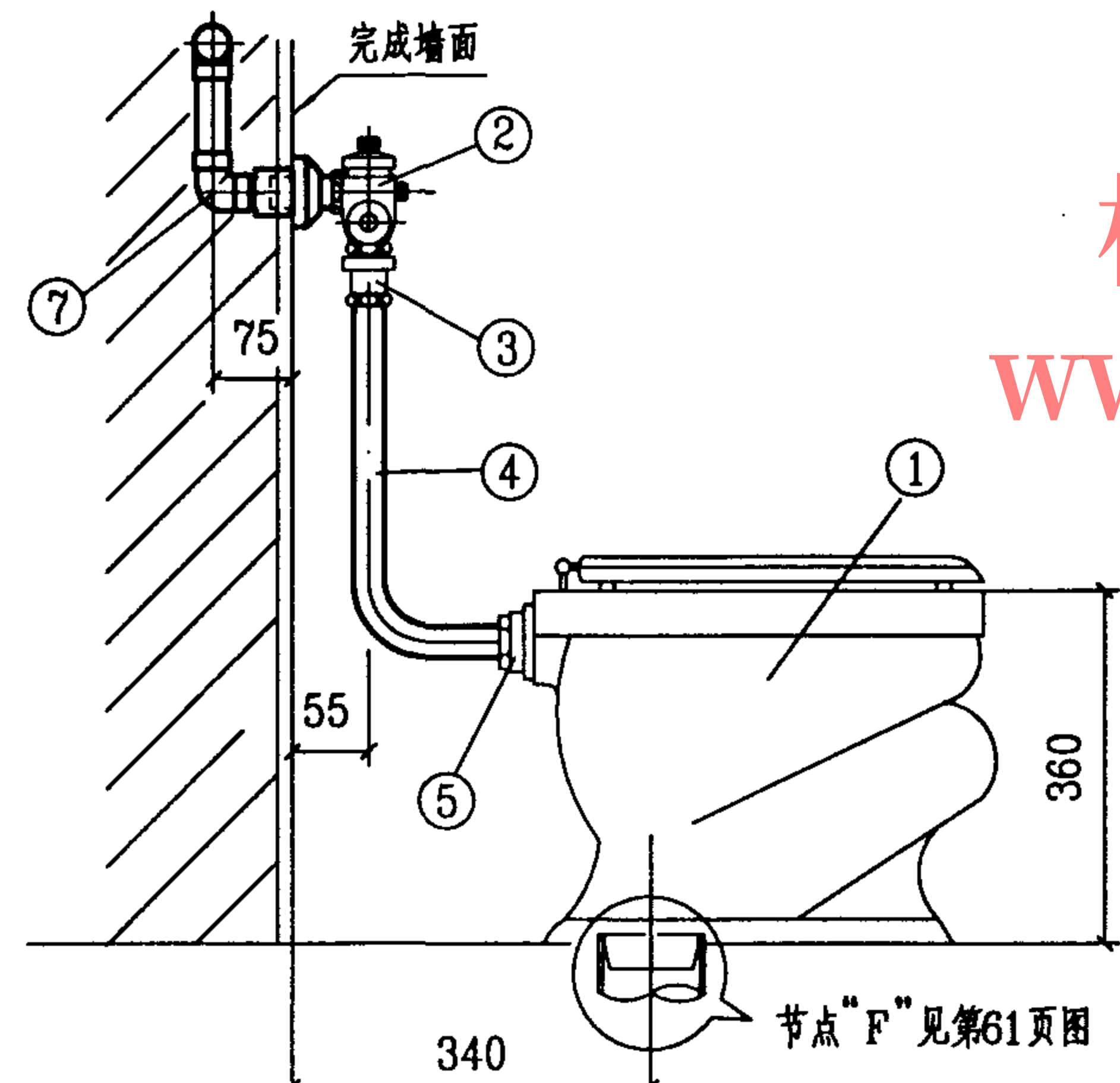
侧面图
