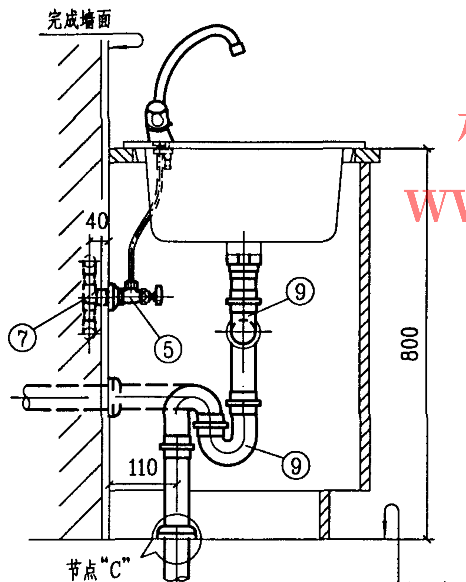
2-2 剖面图
