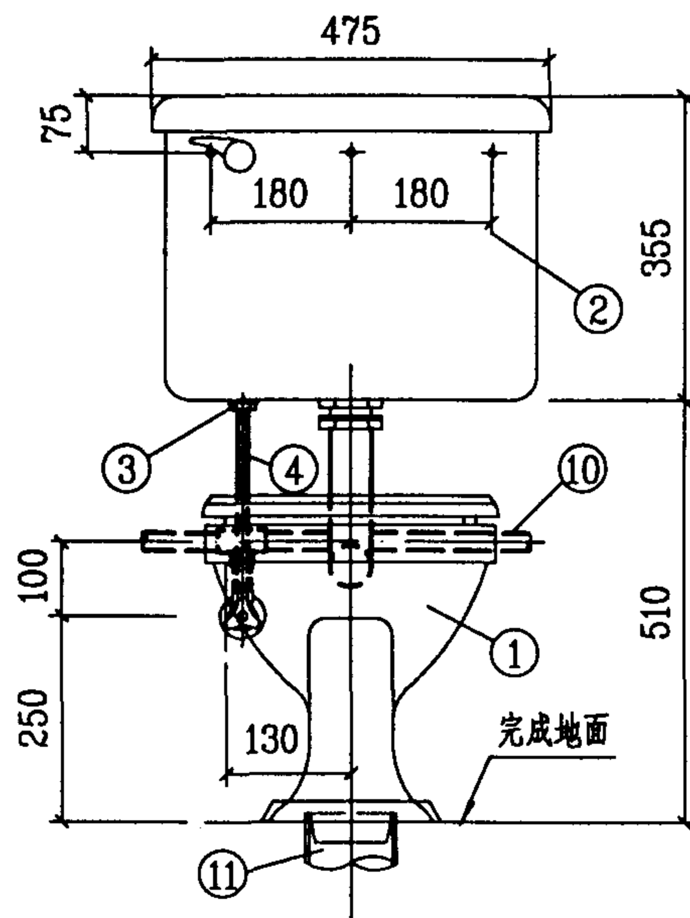
立面图
