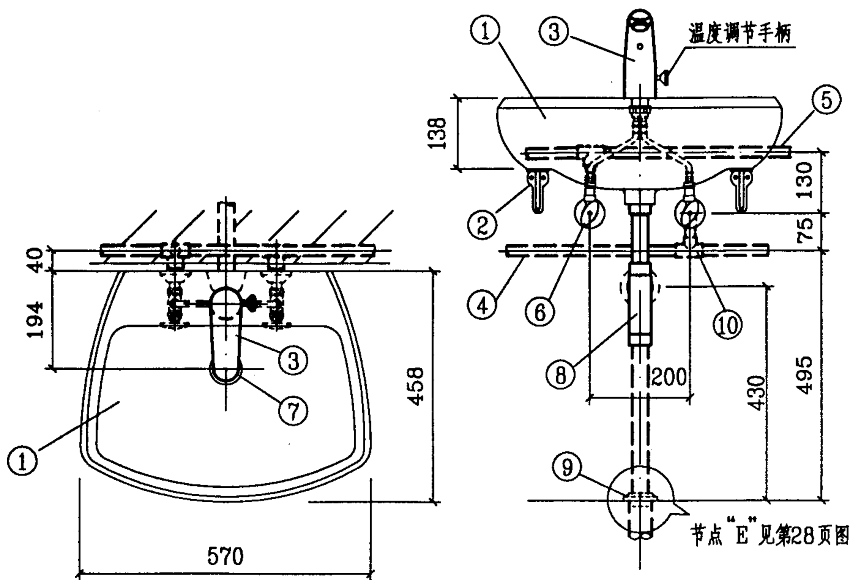
平面图
