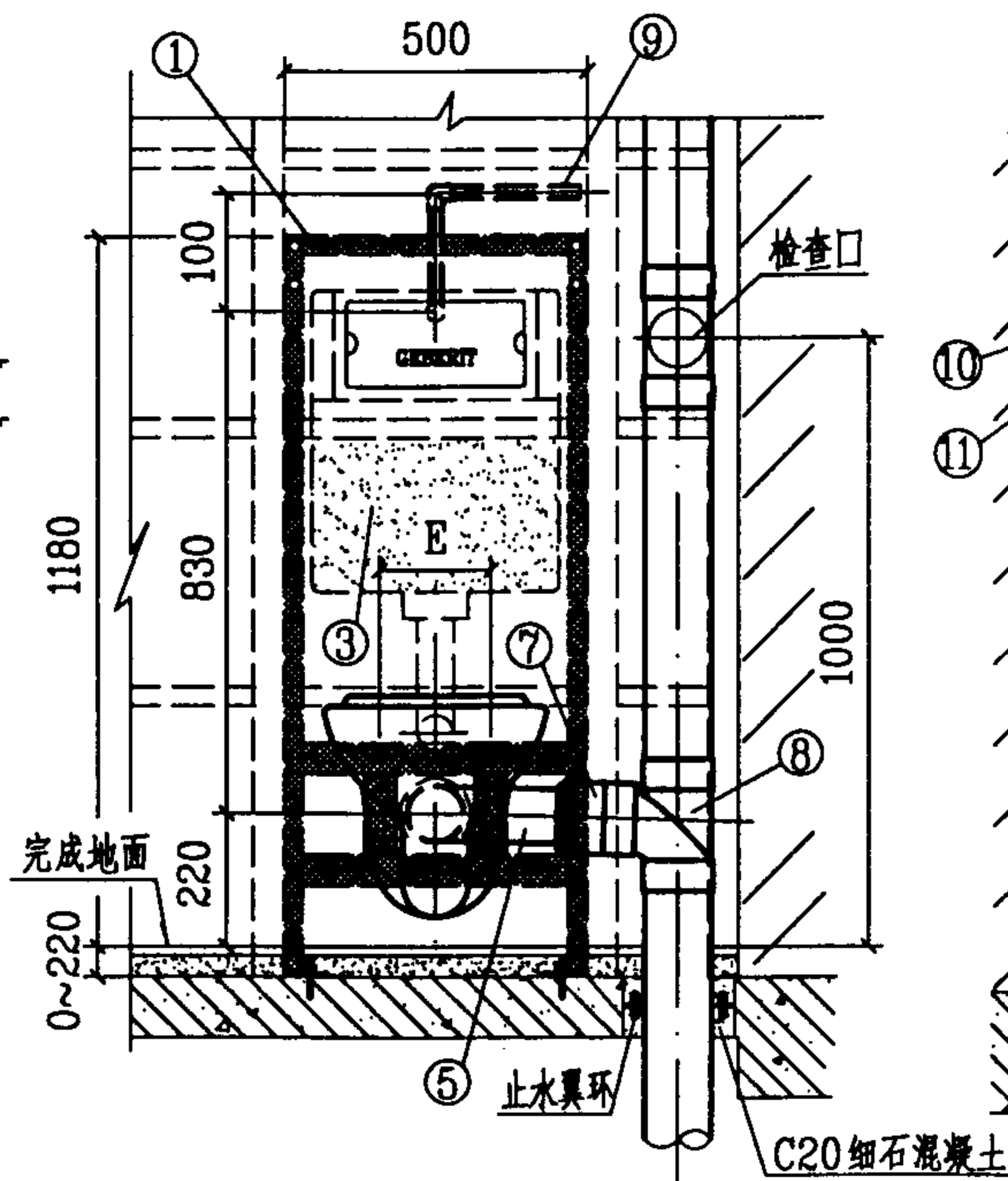
立面图
