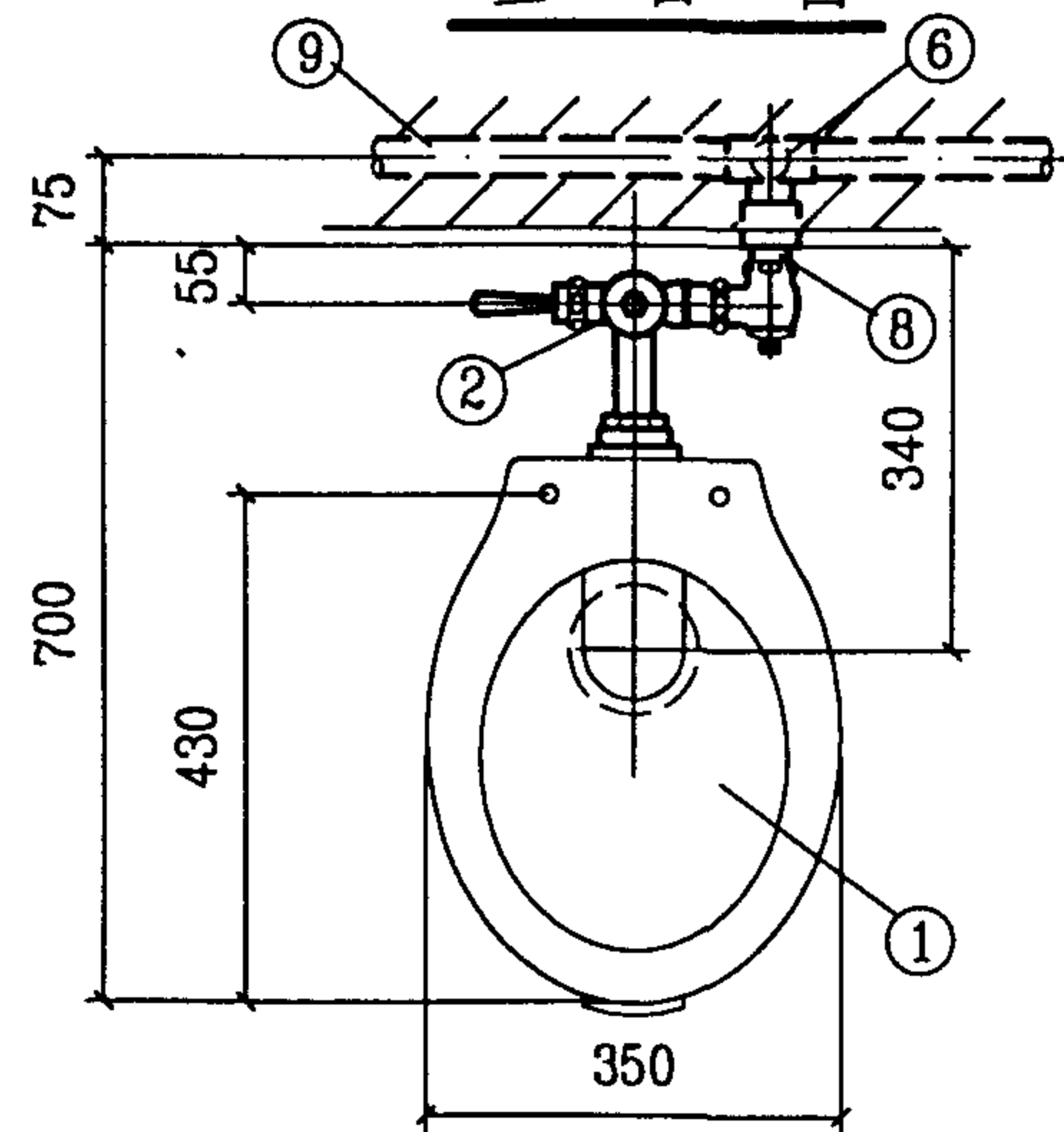
平面图
