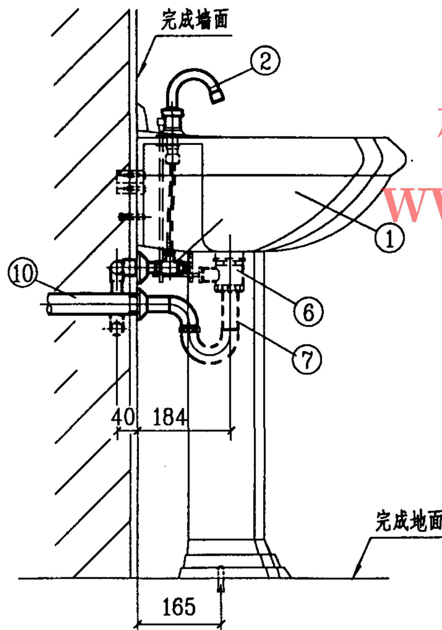
侧面图
