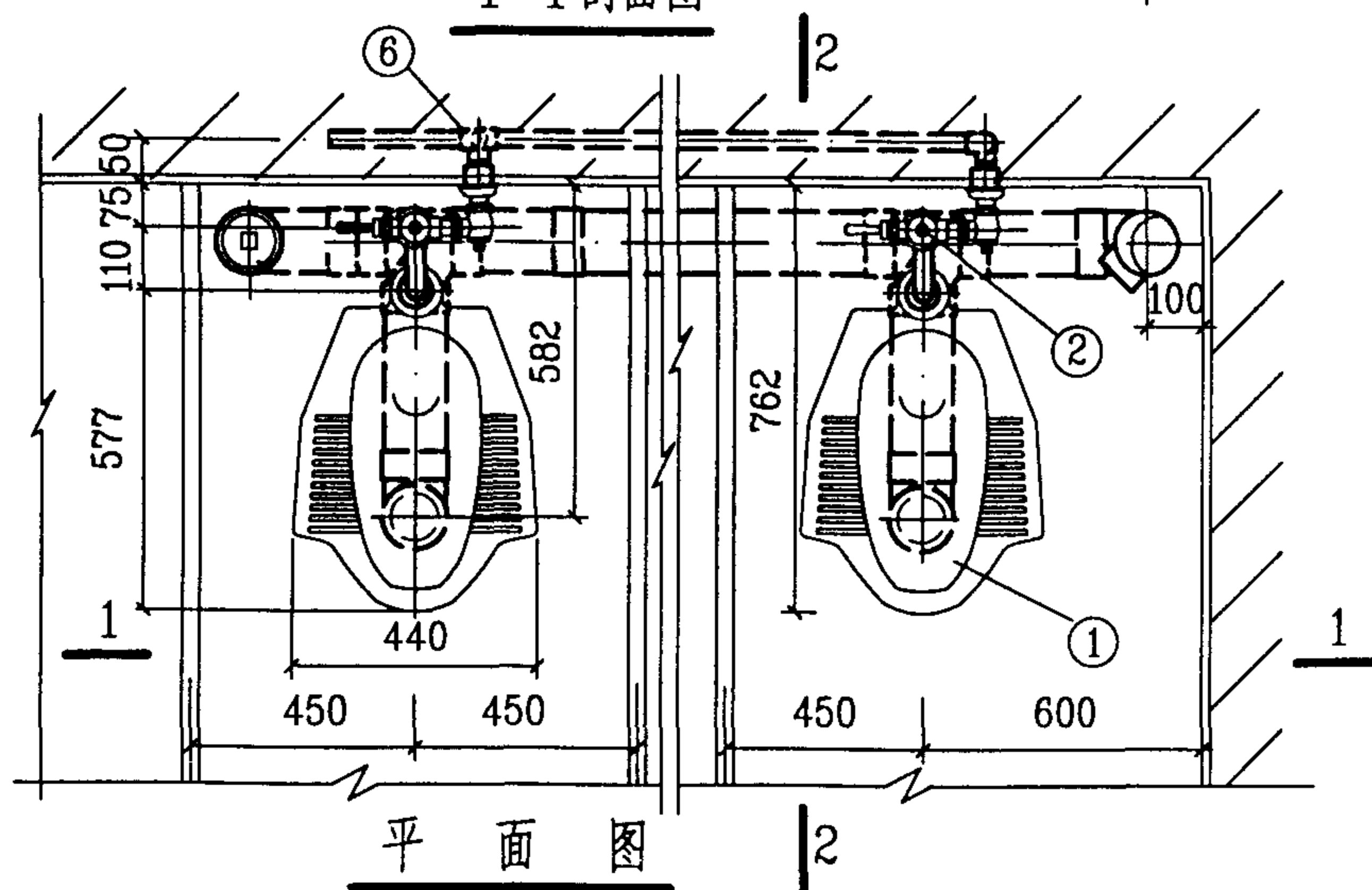
1-1 剖面图
