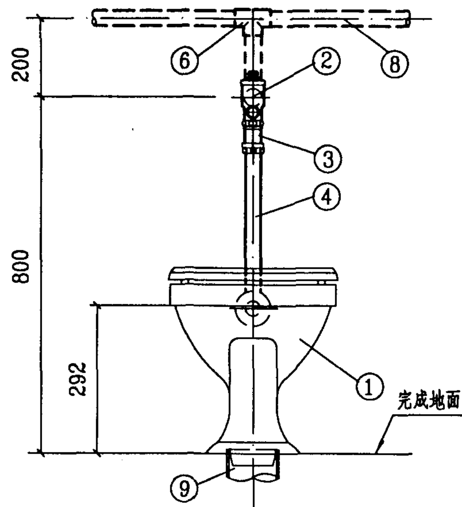
立面图
