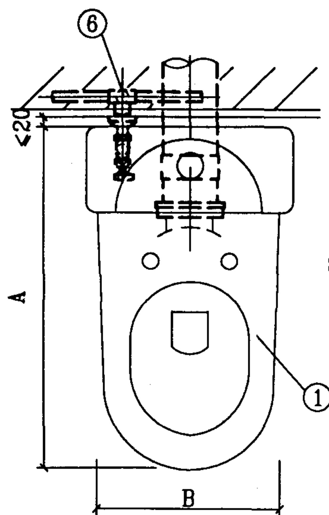
平面图
