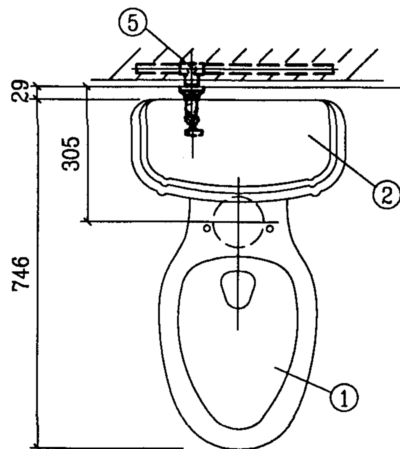
平面图
