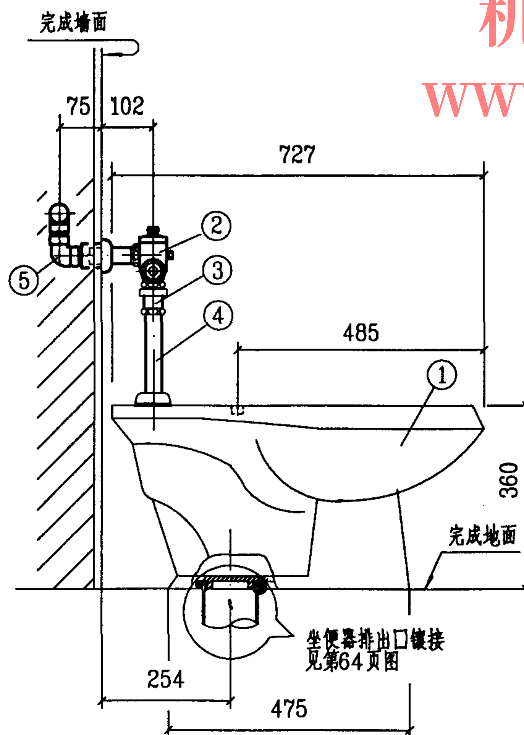
侧面图
