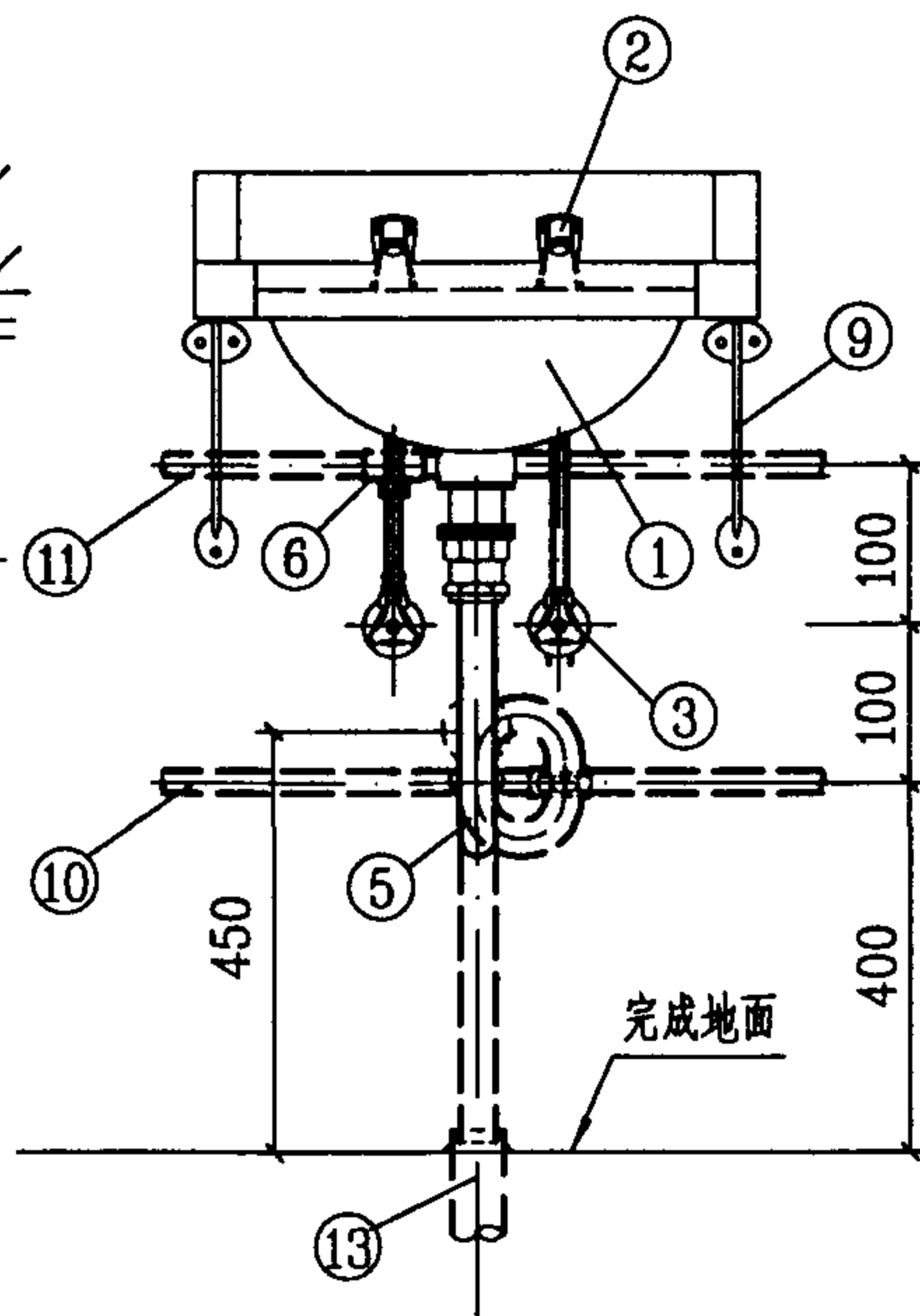
立面图
