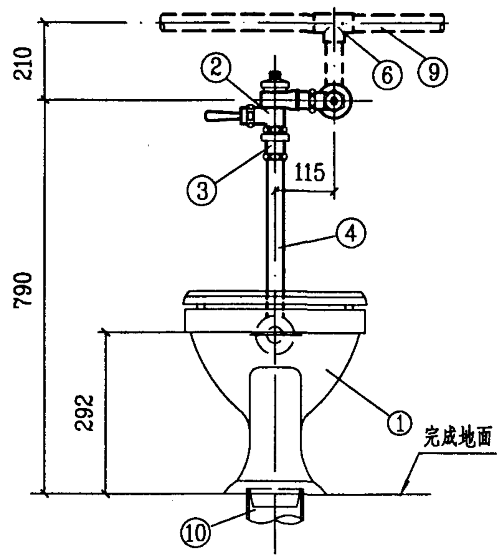
立面图
