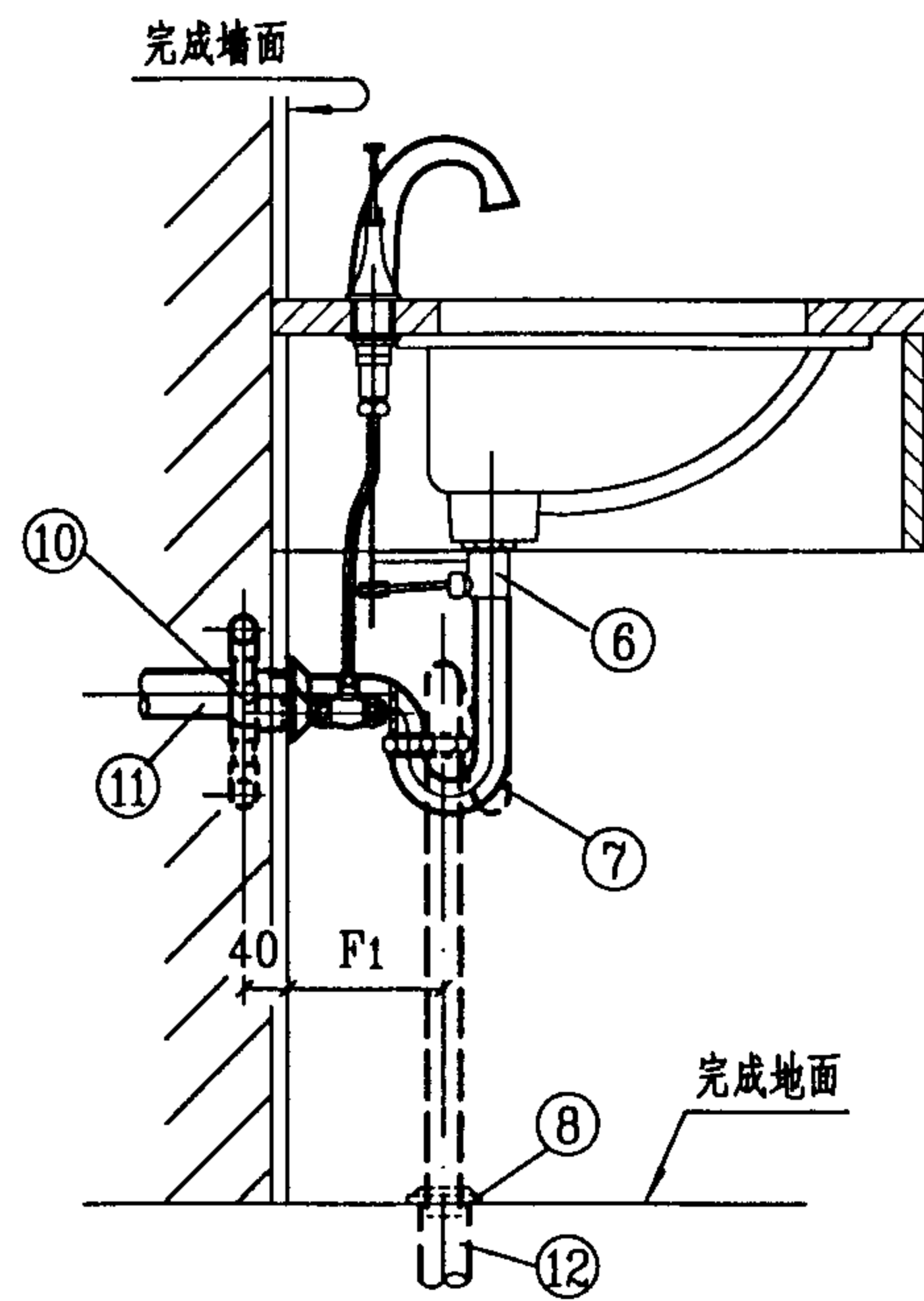
2-2 剖面图
