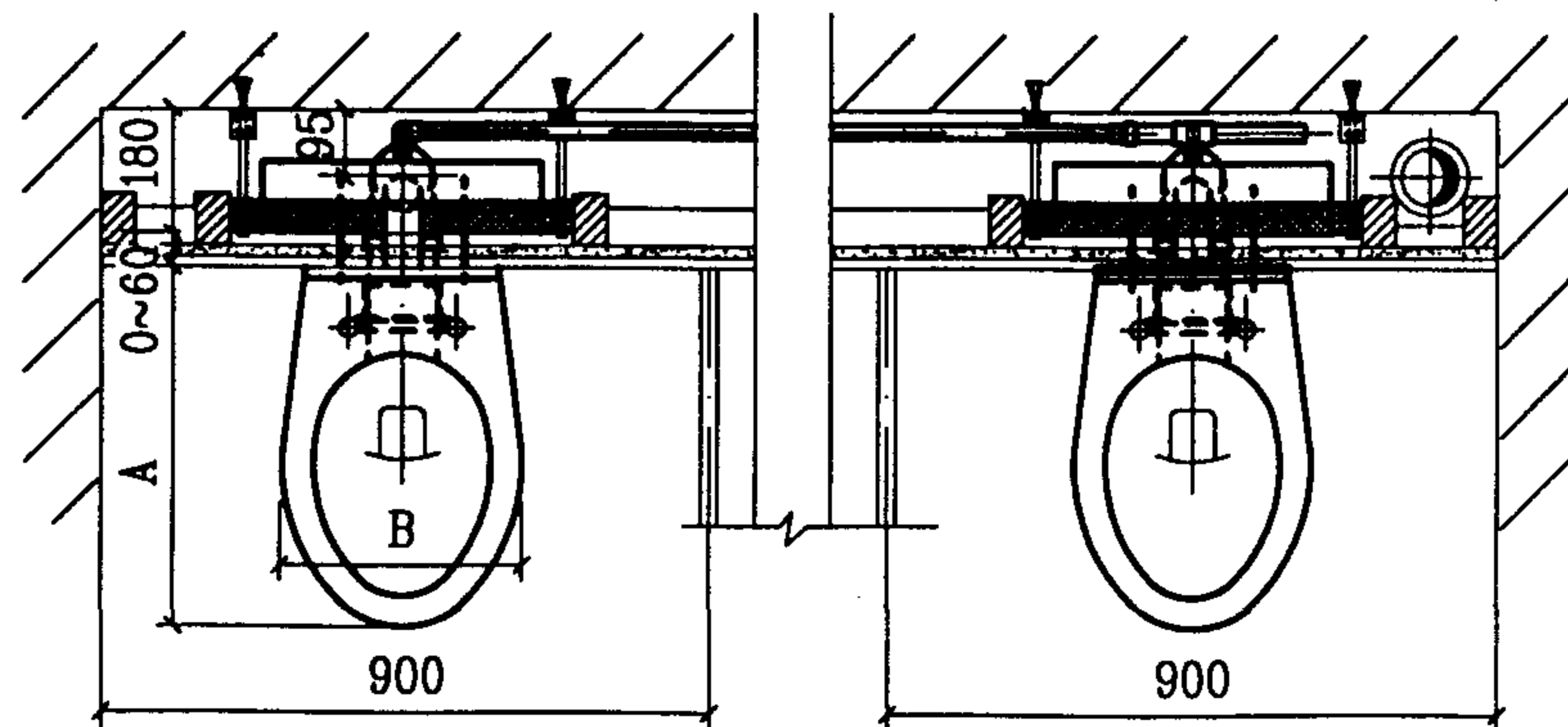
平面图
