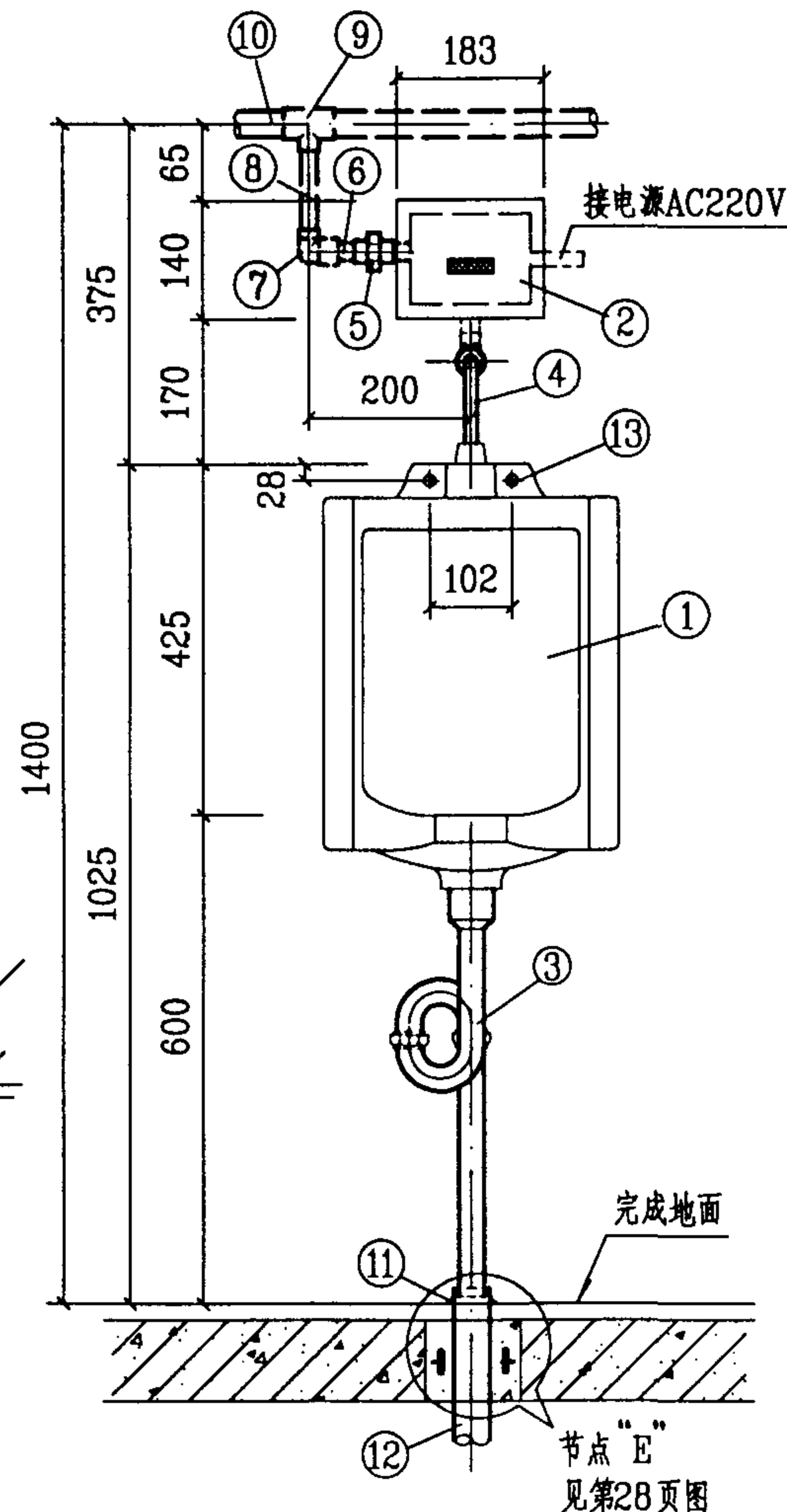
立面图
