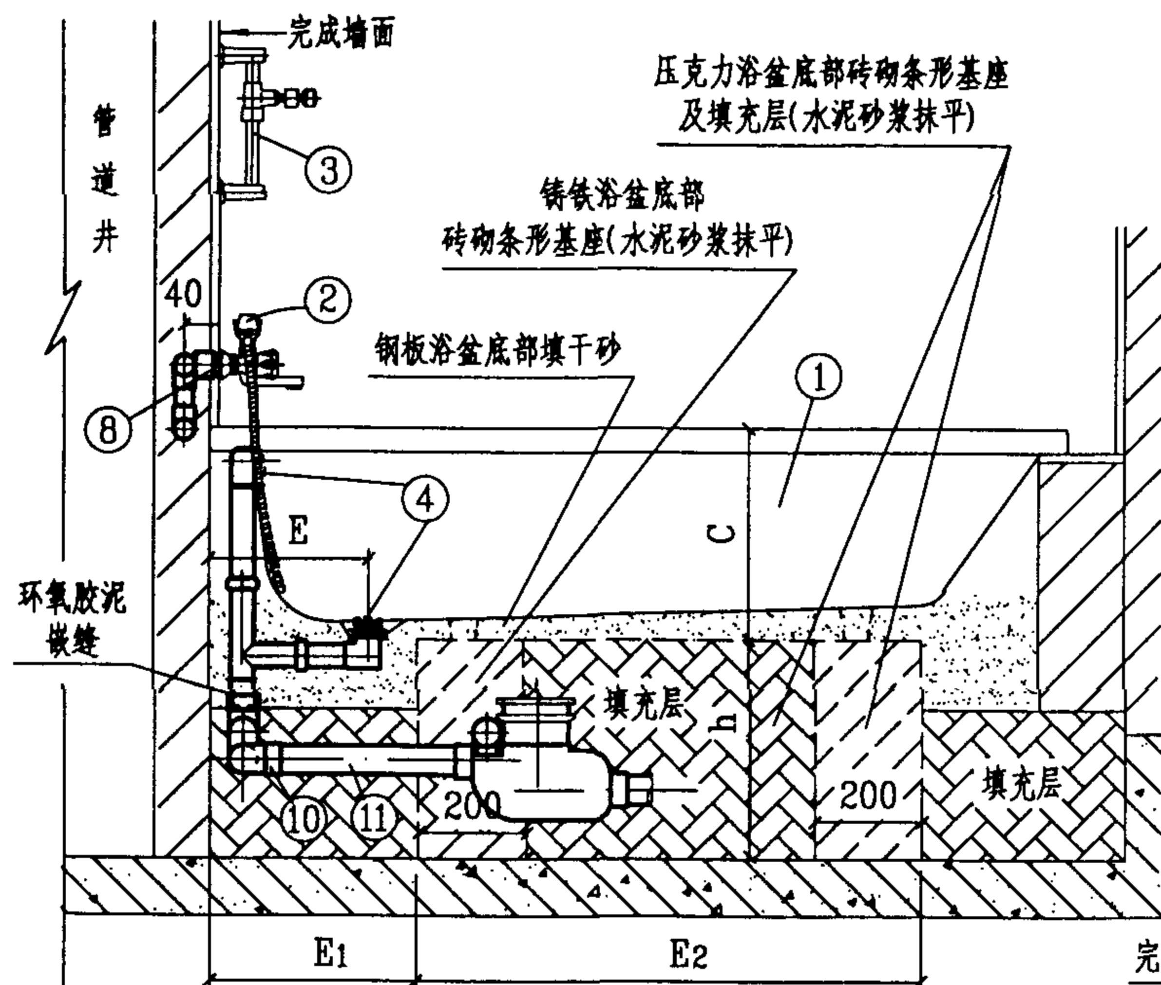
1-1 剖面图
