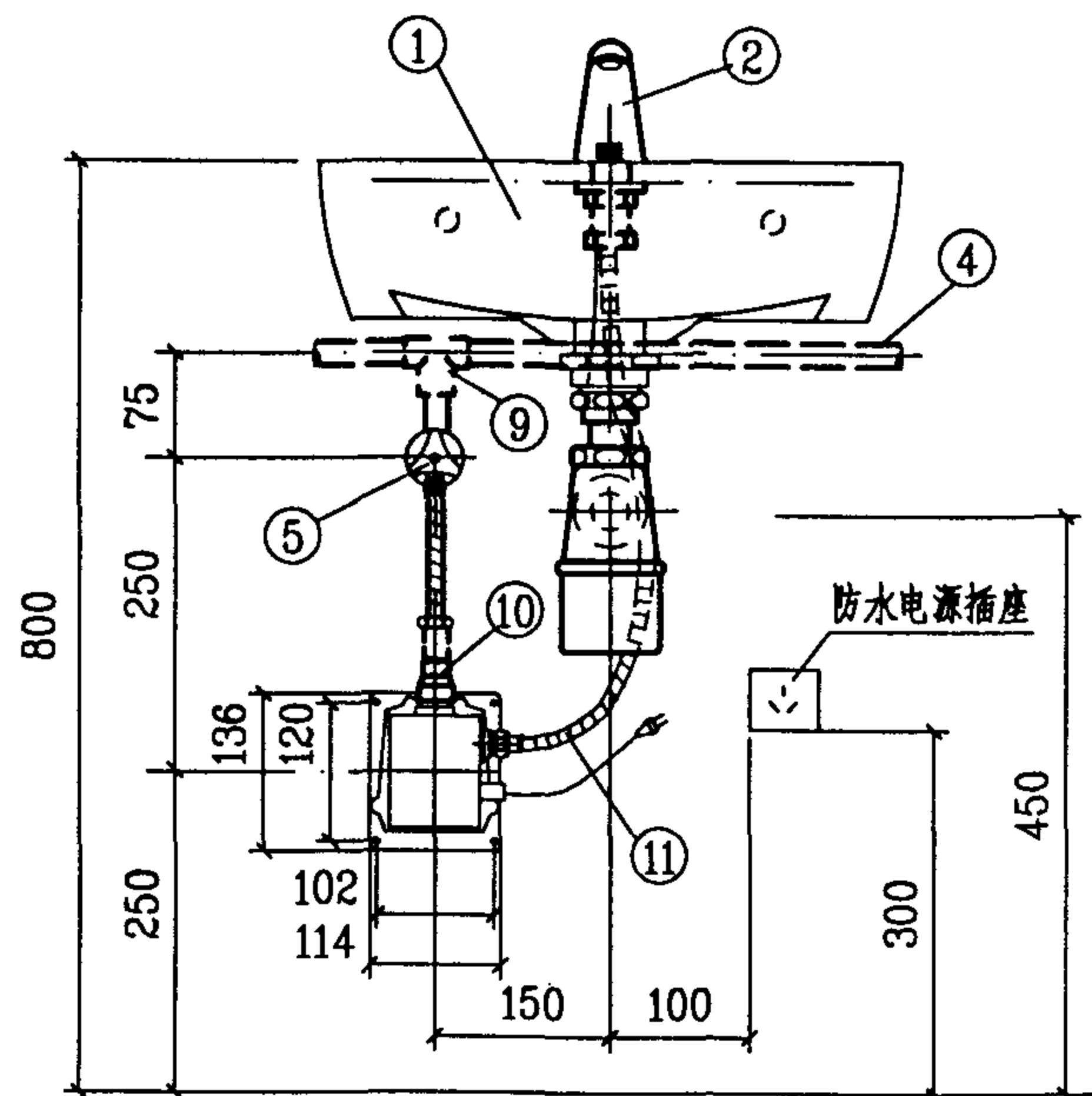
立面图
