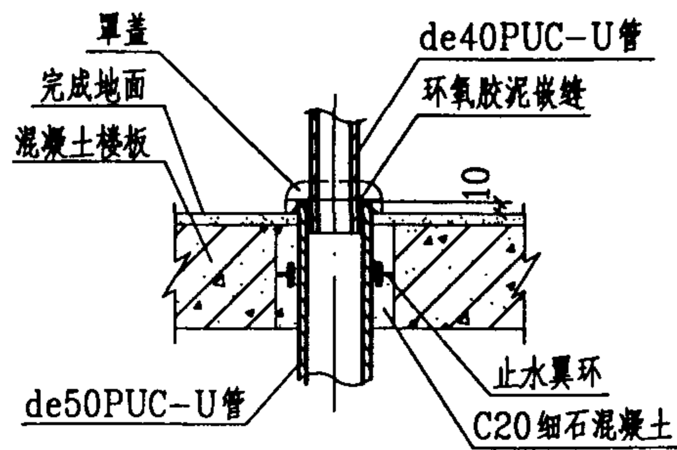
节点 "C"
