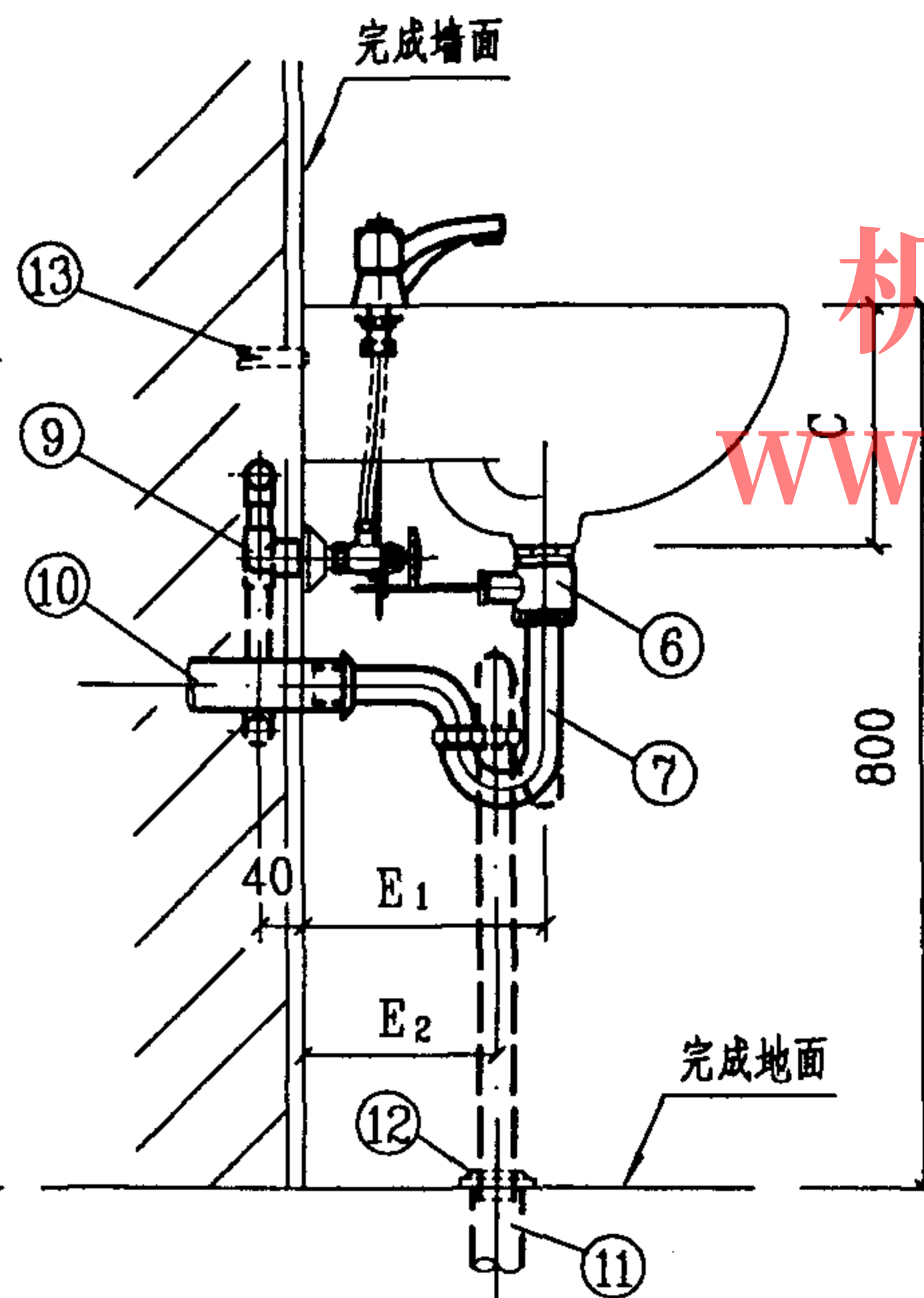
侧面图
