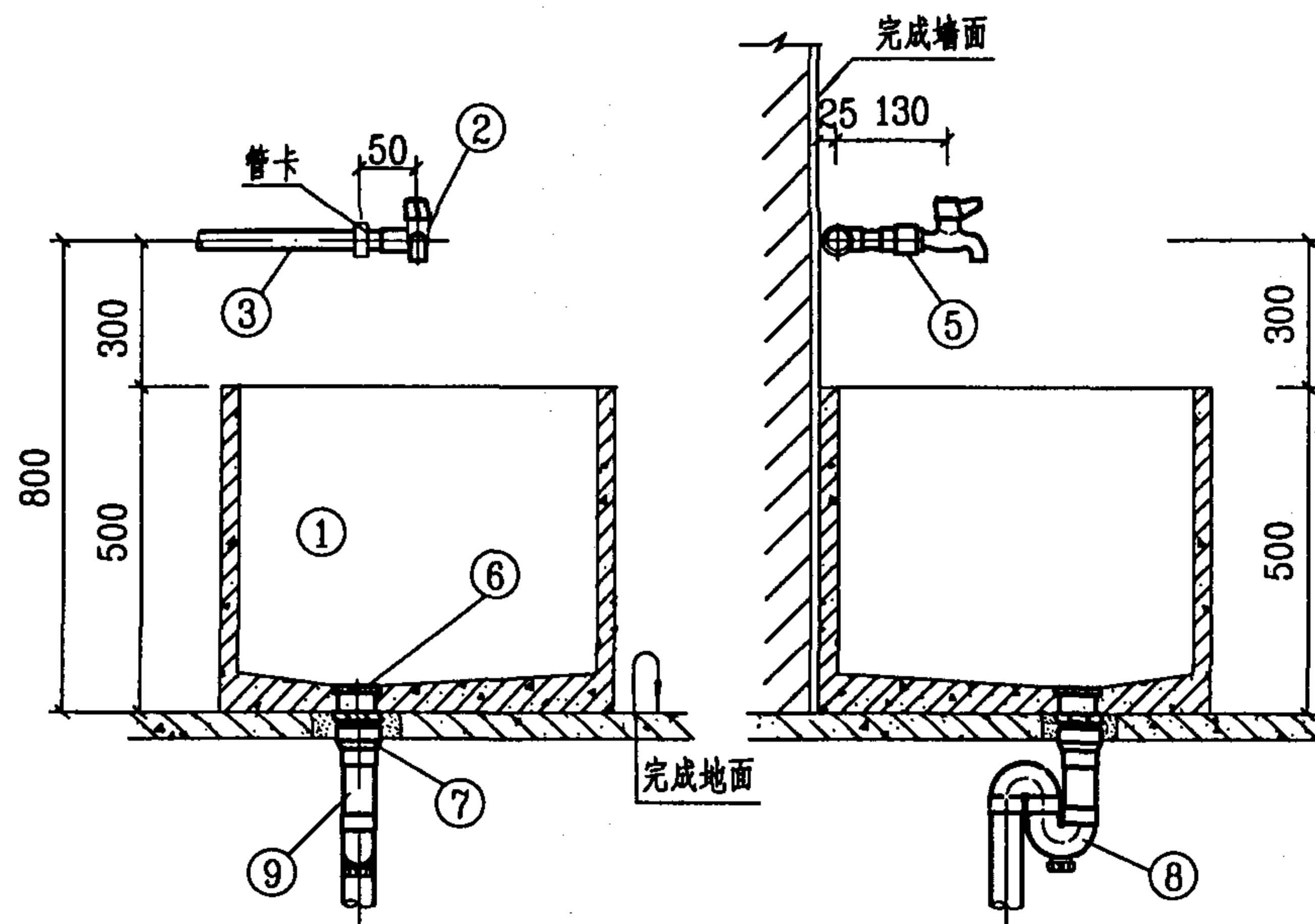
1-1剖面图
