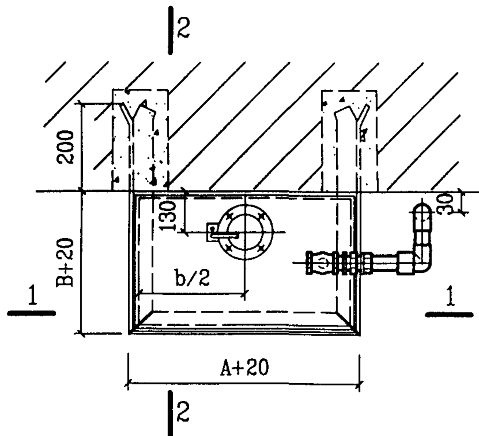
平面图
