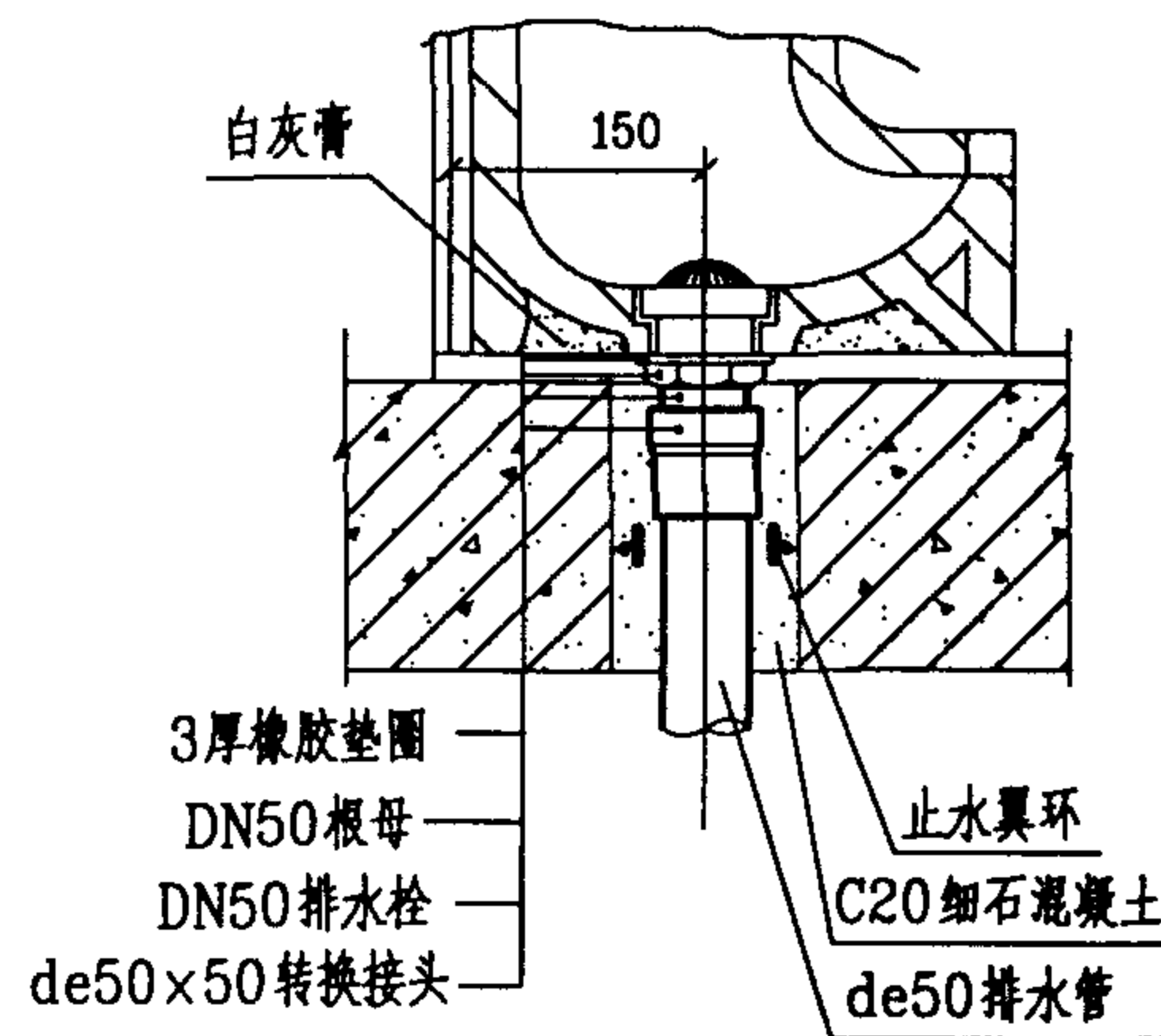
节点 "G"
