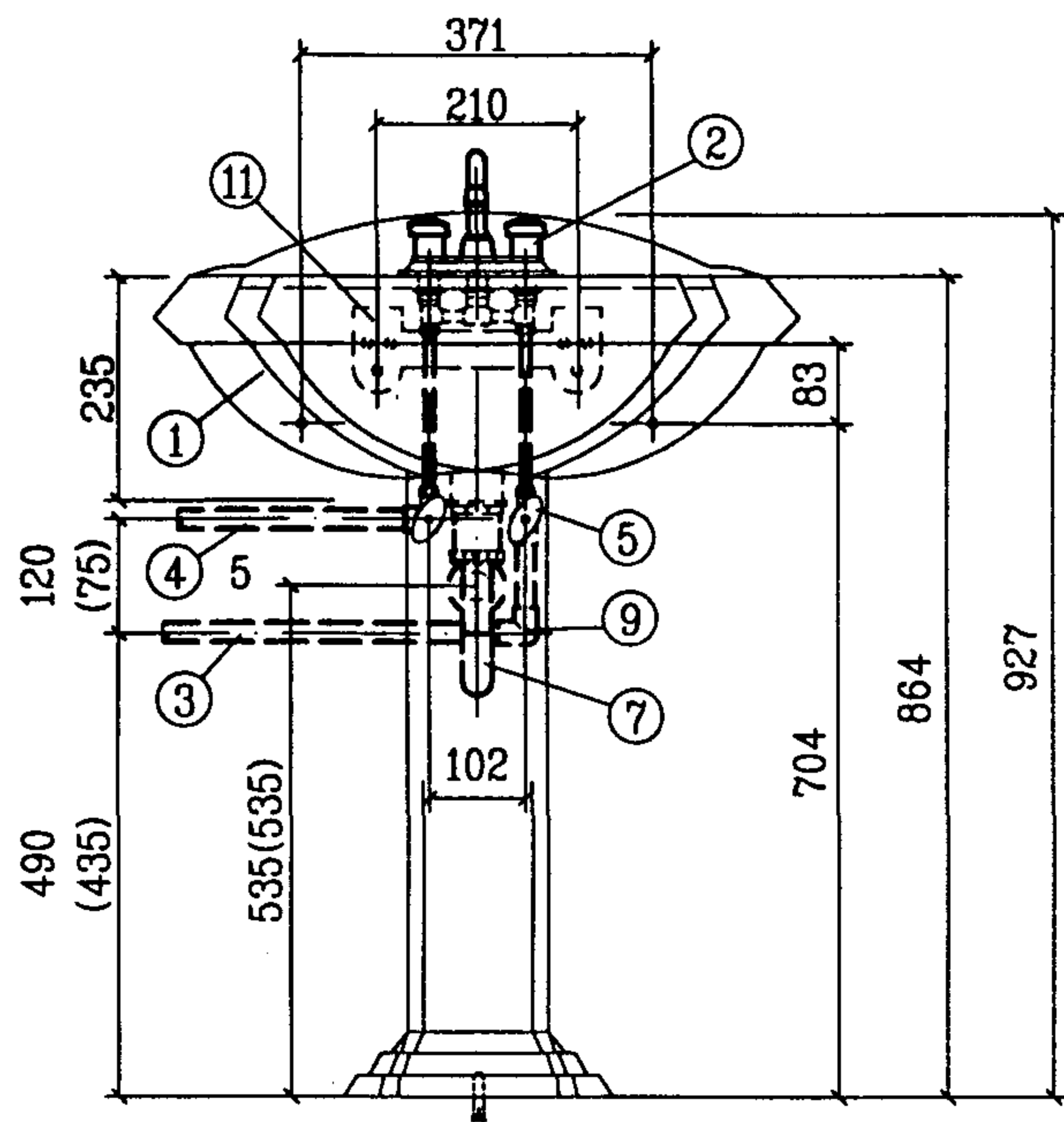
立面图
