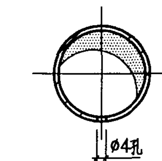
穿孔出水管大样图
