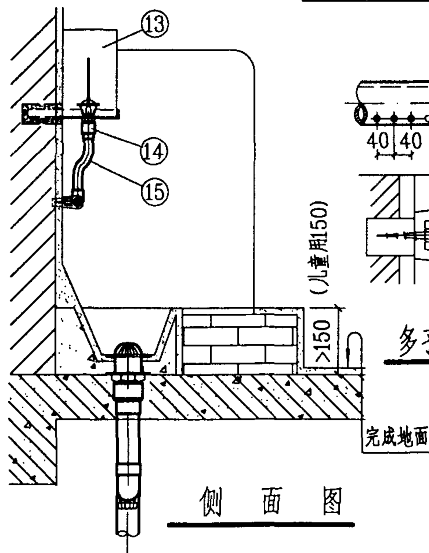
自动冲洗小便槽安装图(甲、乙型)
