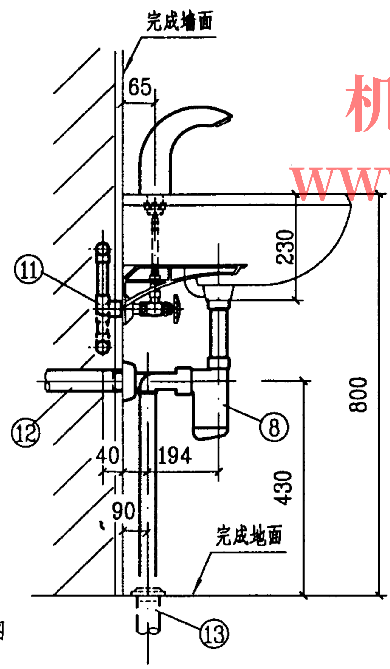
侧面图
