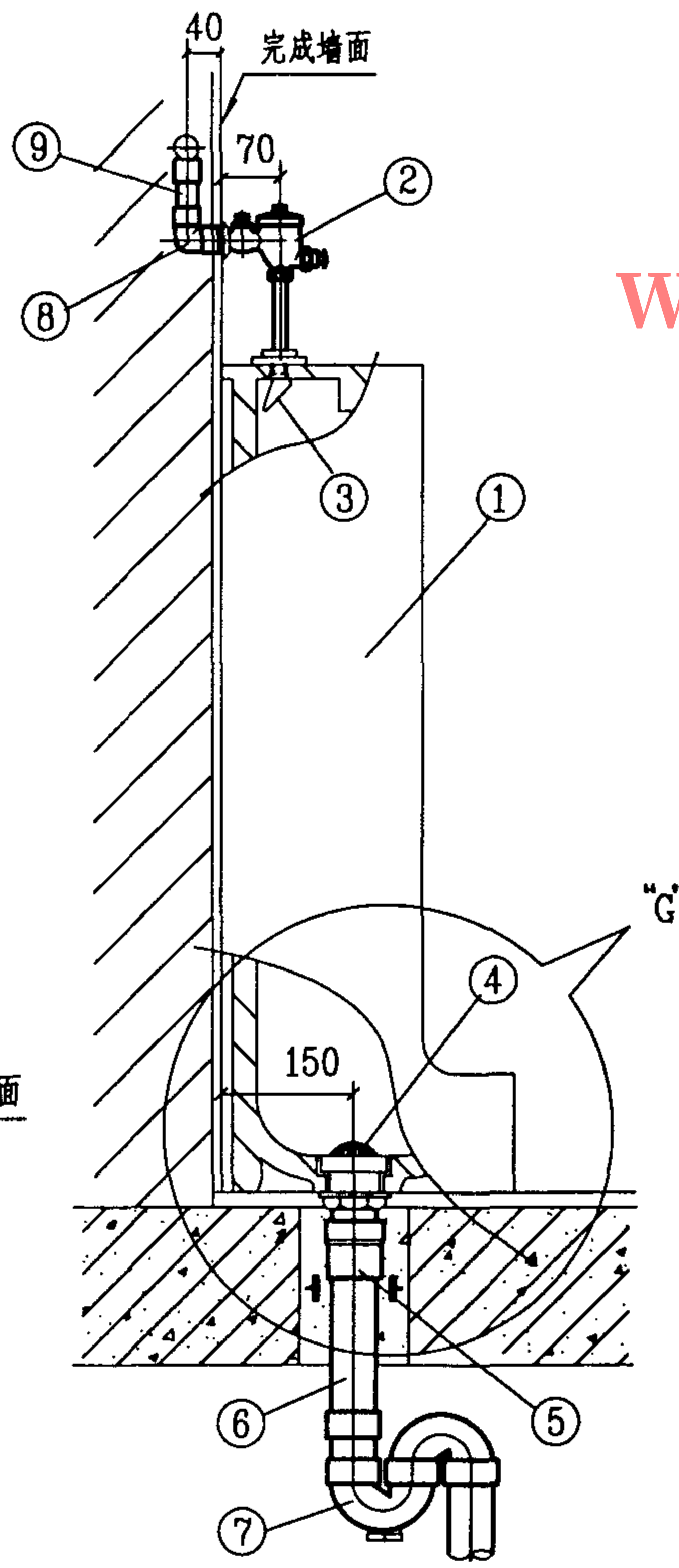
侧面图
