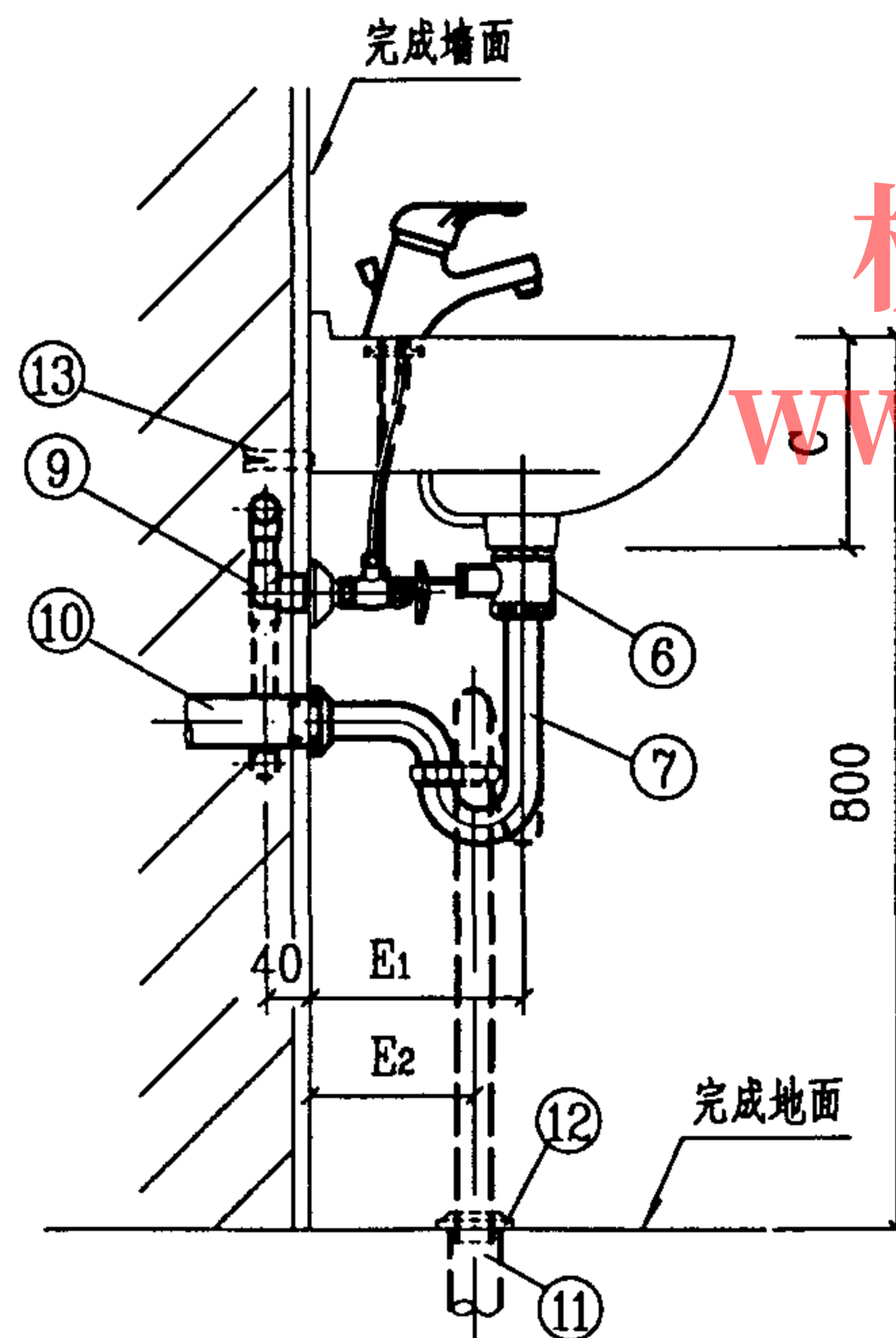
侧面图
