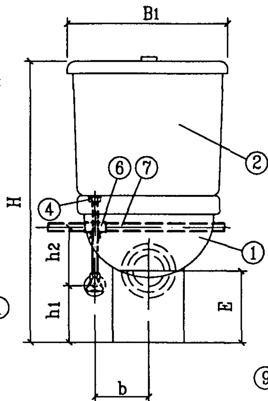
立面图
