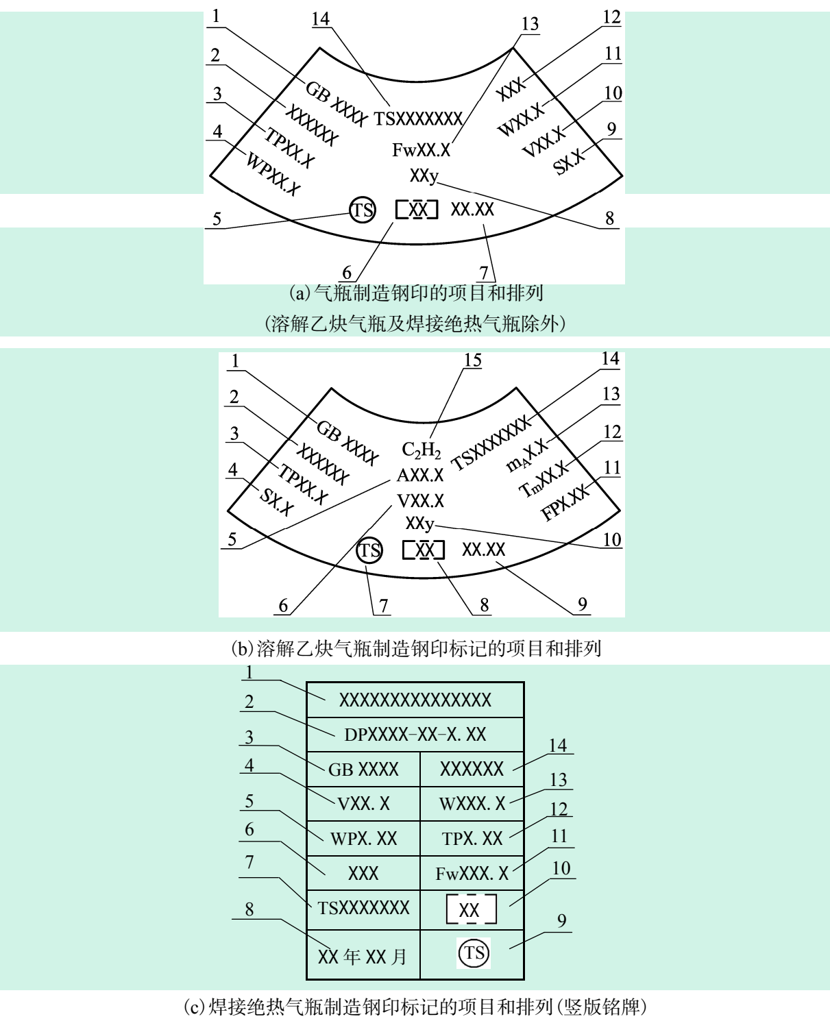
图 B-2 制造钢印标记的项目和排列
