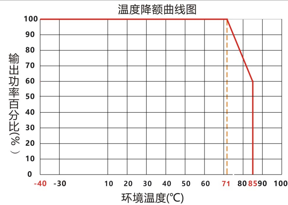
工作环境温度降额曲线图
