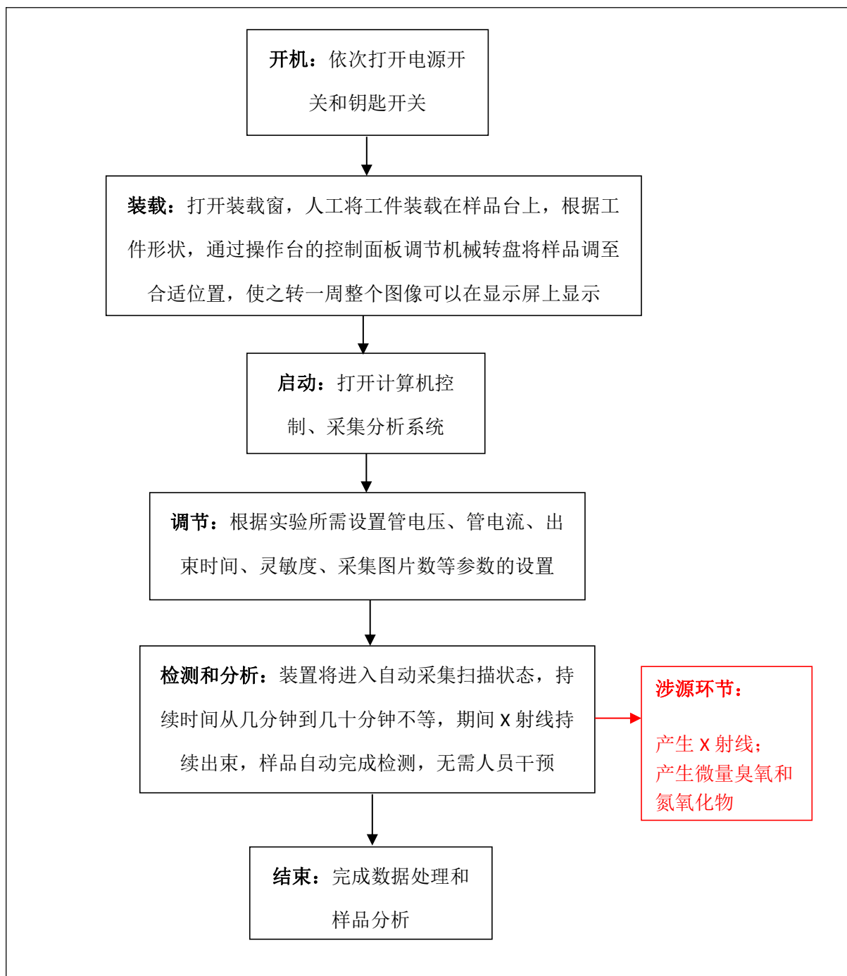
图 3-5 操作流程
