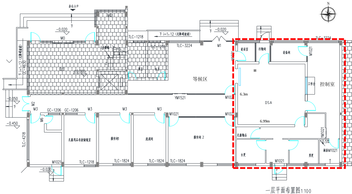
图 1-2 本项目 DSA 机房改建后平面布局图（虚线框内为 DSA 机房改建后布局）
