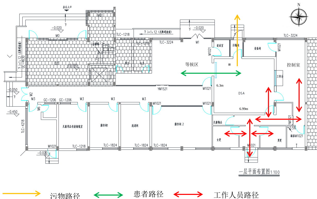
图 9-4 本项目辐射工作场所人流物流示意图
