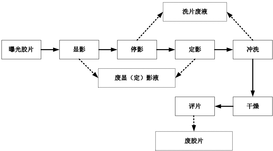
图 9-4 暗室洗片工艺流程及产污环节示意图
