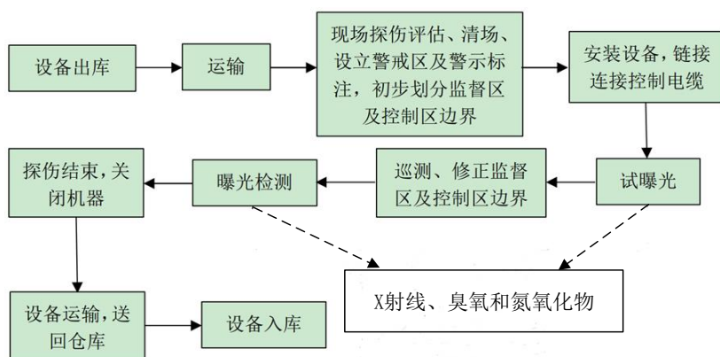
图 9-3 移动探伤工艺流程及产污环节示意图
